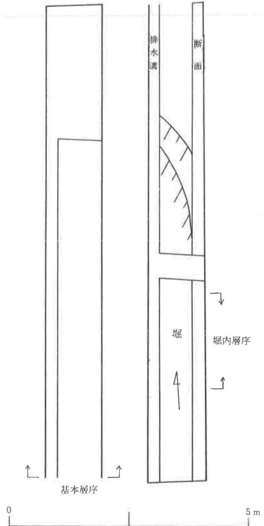
図15 遺構平面図
