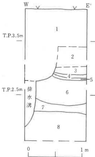
図14 基本層序
