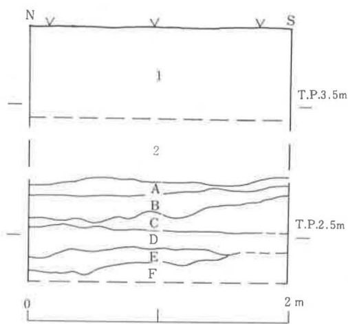
図16 堀内層序
