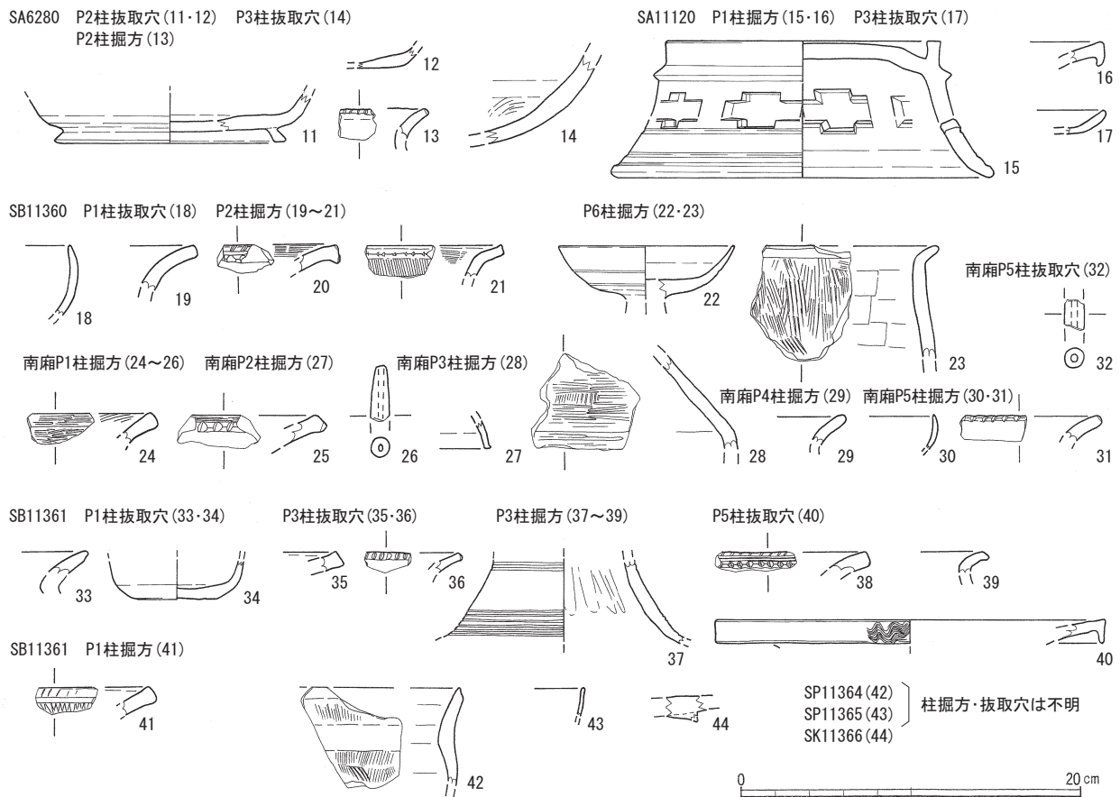
第II-10図 第199次調査 出土遺物実測図2 (1:4)
