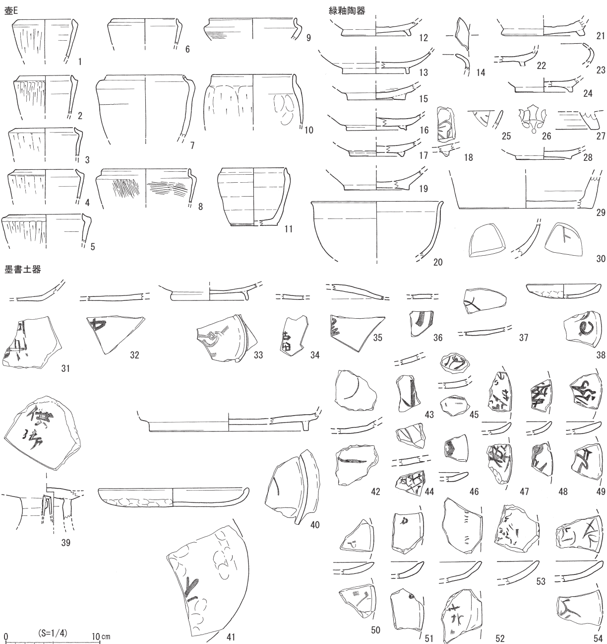
第三-1図 重要考古資料 遺物実測図1 (1:4)
