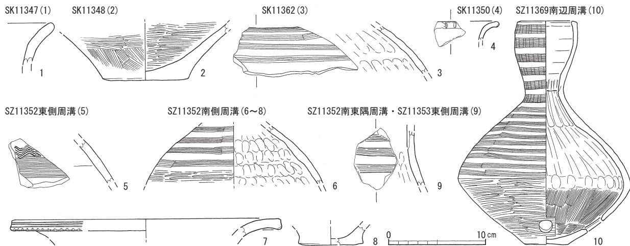
第Ⅱ-9図 第199次調査 出土遺物実測図1 (1:4)
