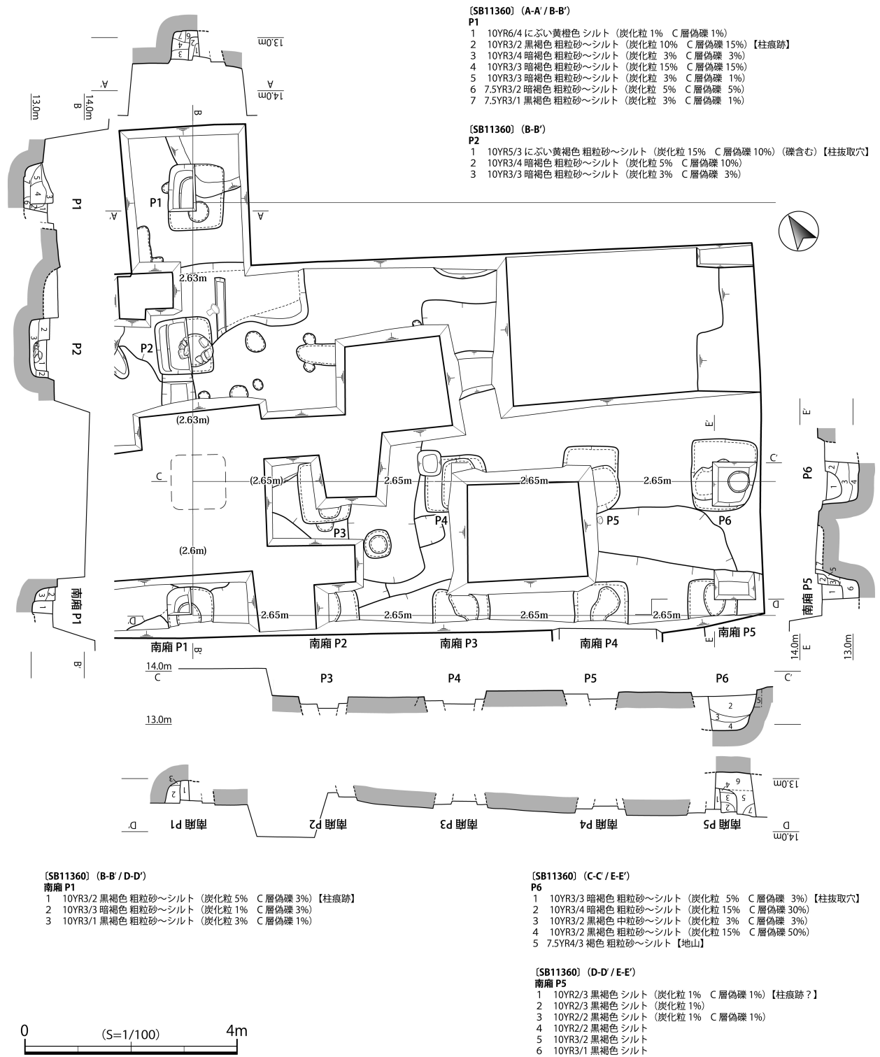
第II-7図 SB11360平面・断面図 (1:100)
