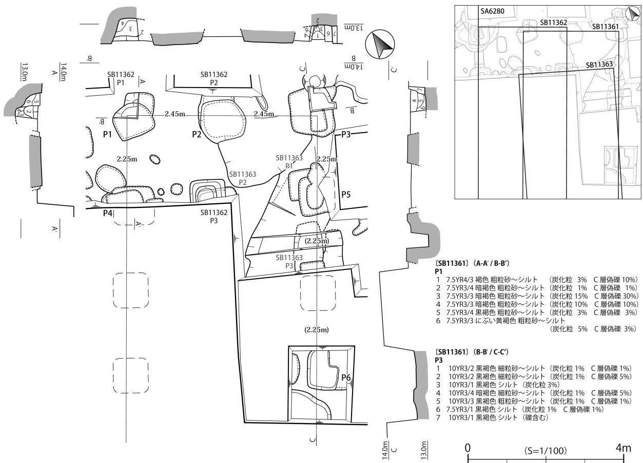
第Ⅱ-8図 SB11361平面・断面図(1:100)
