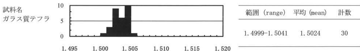
図1 火山ガラスの屈折率測定結果
