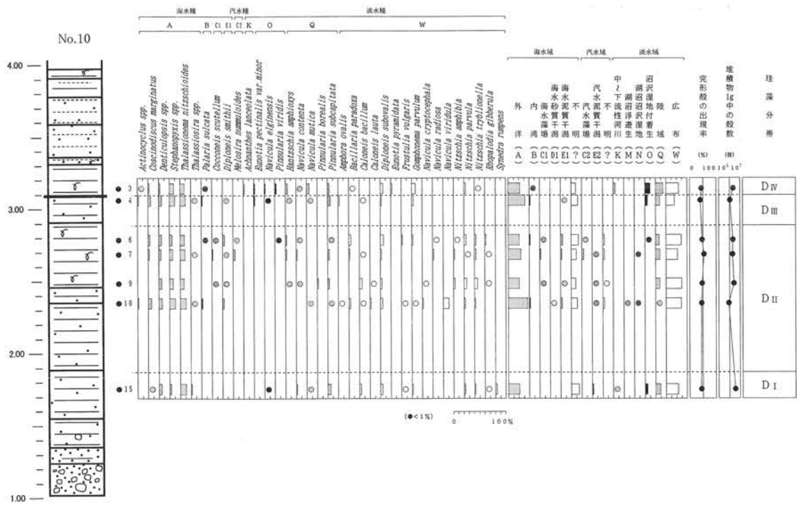
図1 No.10地点ボーリング堆積物中の珪藻化石分布図（2%以上の分類群を表示）
