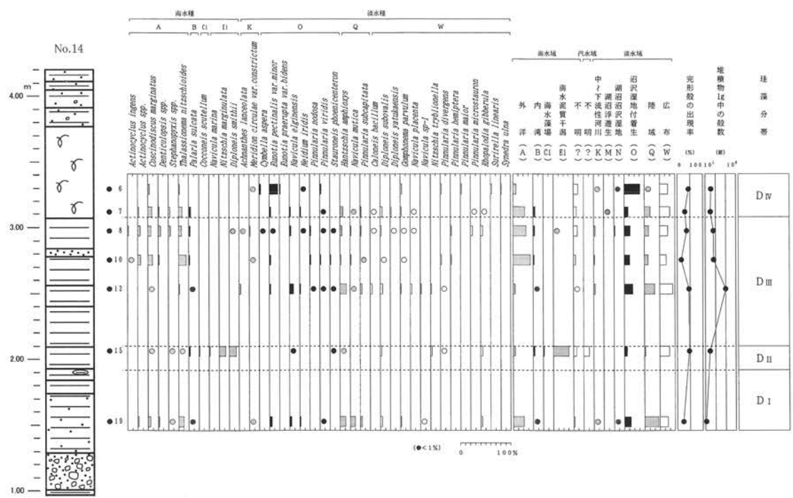
図2 No.14地点ボーリング堆積物中の珪藻化石分布図（2%以上の分類群を表示）
