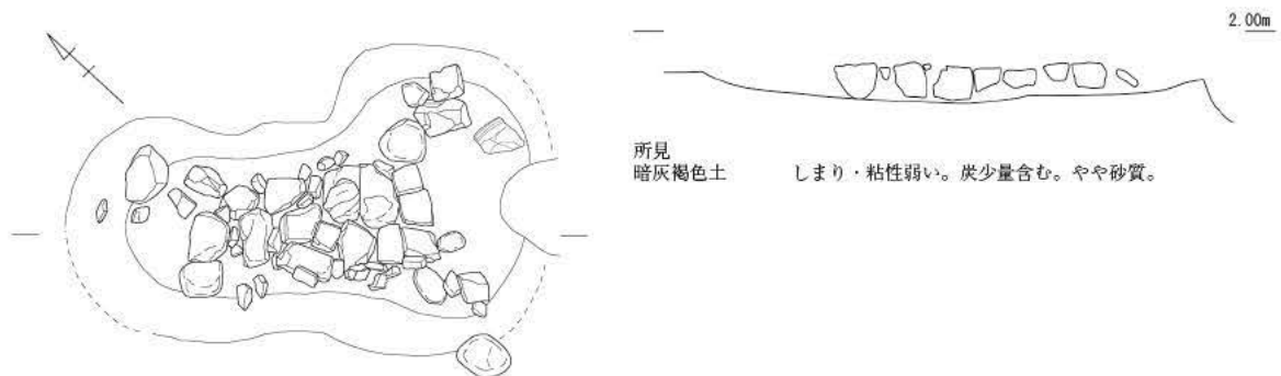
第16図 2号土坑平面図 (S=1/40)
