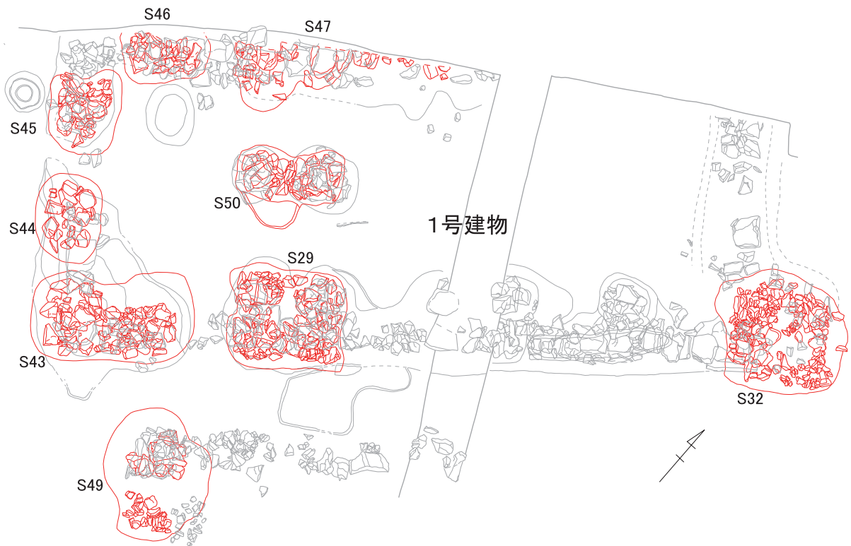
第8图 1号建物基础平面图 (S=1/80)
