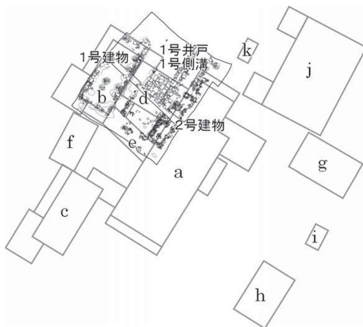
第25図 A区検出遺構と大正8年頃警露館模式図(S=1/500)
