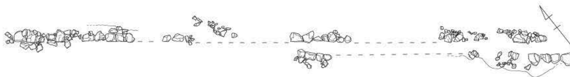
第20図 3号側溝平面図 (S=1/160)
