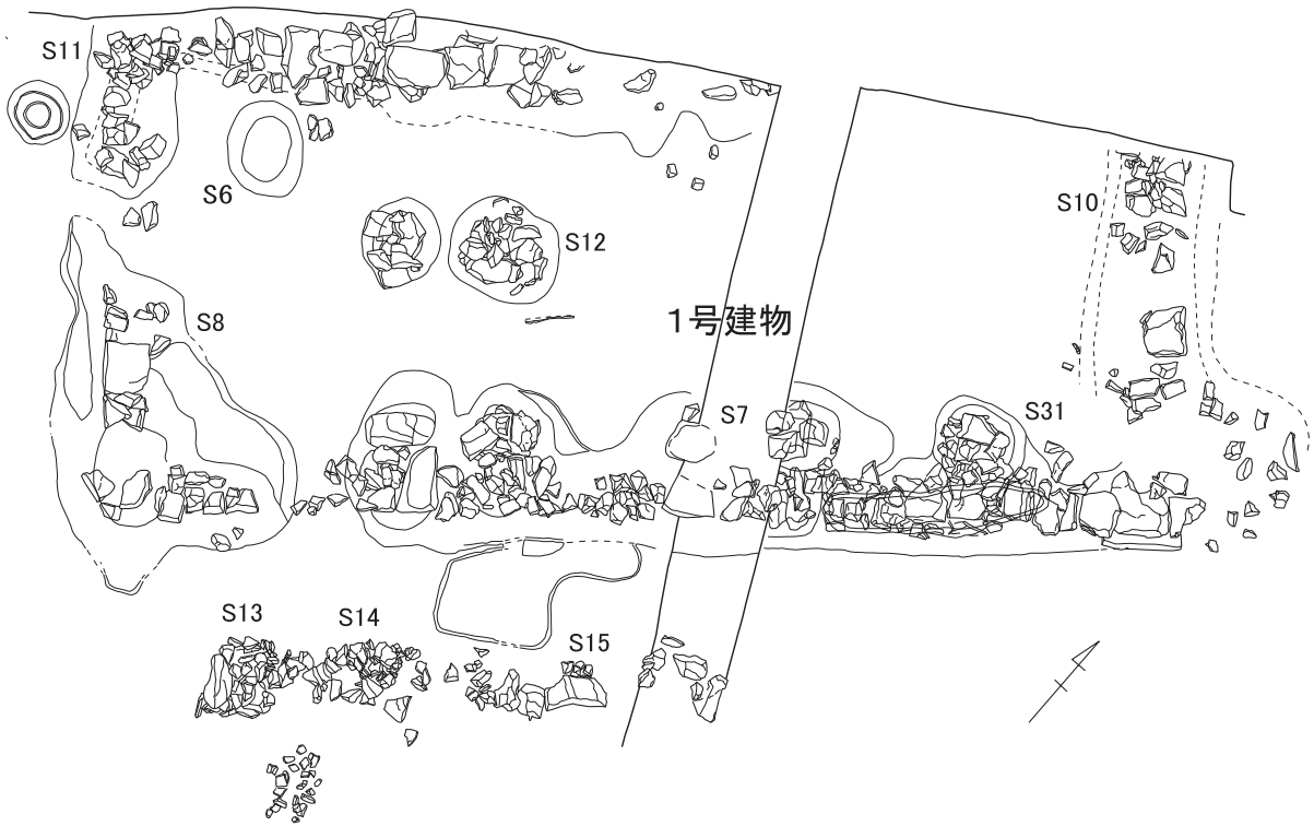
第7图 1号建物礎石平面图 (S=1/80)
