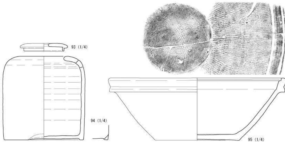
第19図 4号土坑出土遺物(2) (S=1/3)
