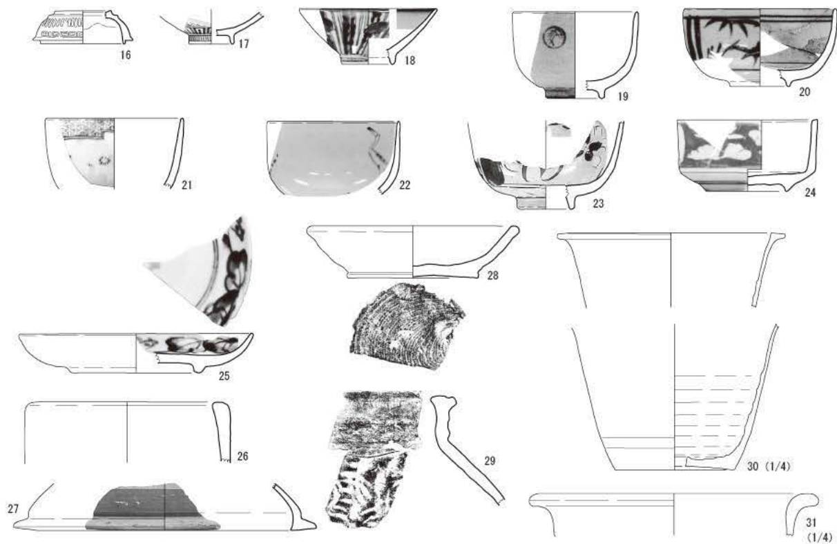
第9図 1号建物出土遺物 (S=1/3)
