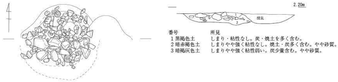
第14図 1号土坑平面図 (S=1/40)
