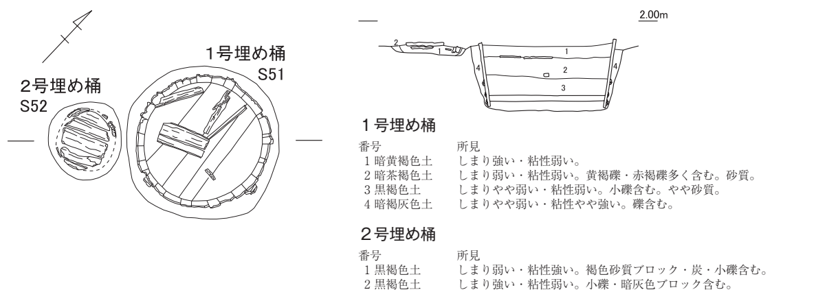
第22図 1号埋め桶・2号埋め桶平面図・断面図 (S=1/80)
