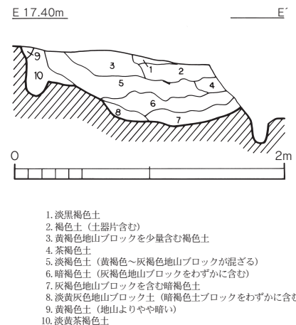
第4図 K-1土層断面図（1/40）
