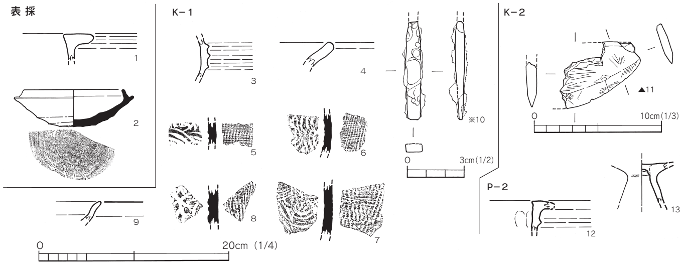
第6図 出土遺物実測図(1/4、※1/2、▲1/3)
