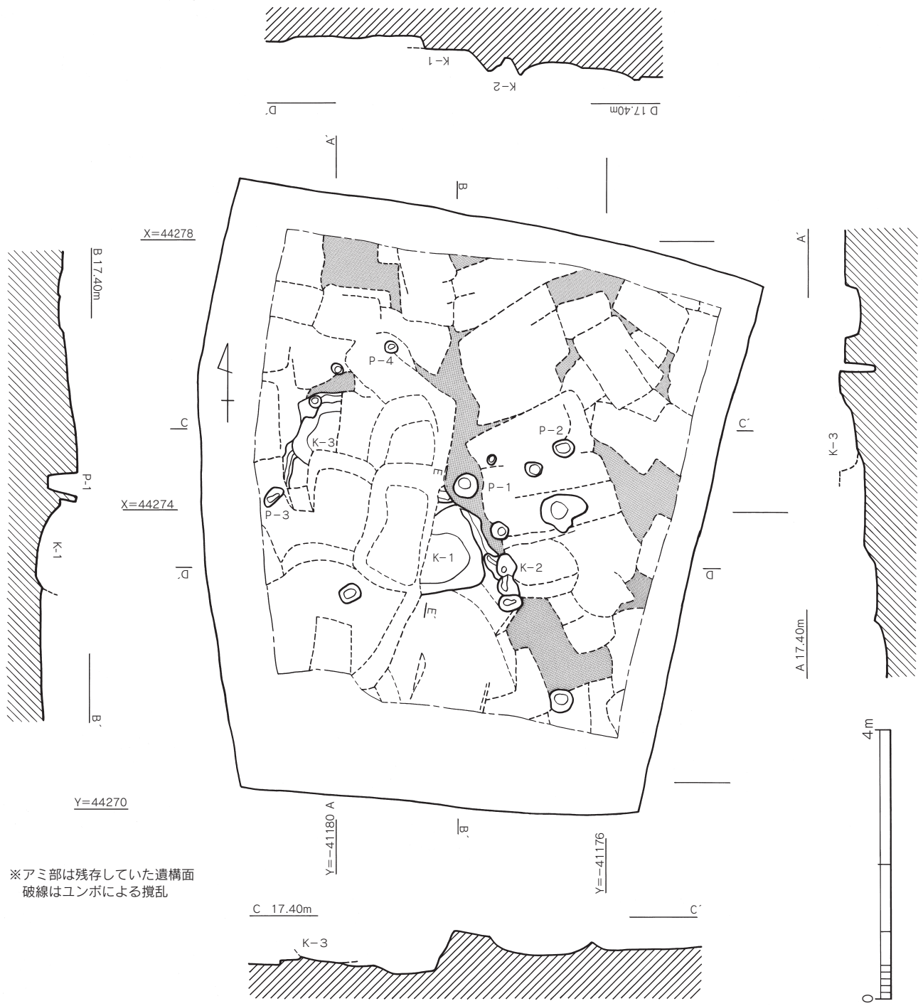
第5図 遺構配置図 (1/80)
