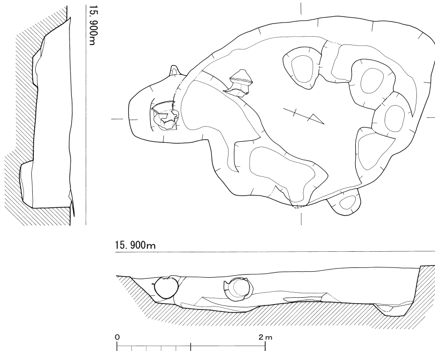
第8図 1号祭祀土坑実測図 (S=1/40)
