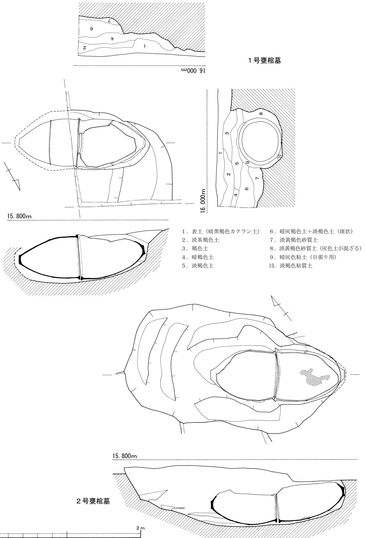
第4図 1・2号甕棺墓実測図 (S=1/30)
