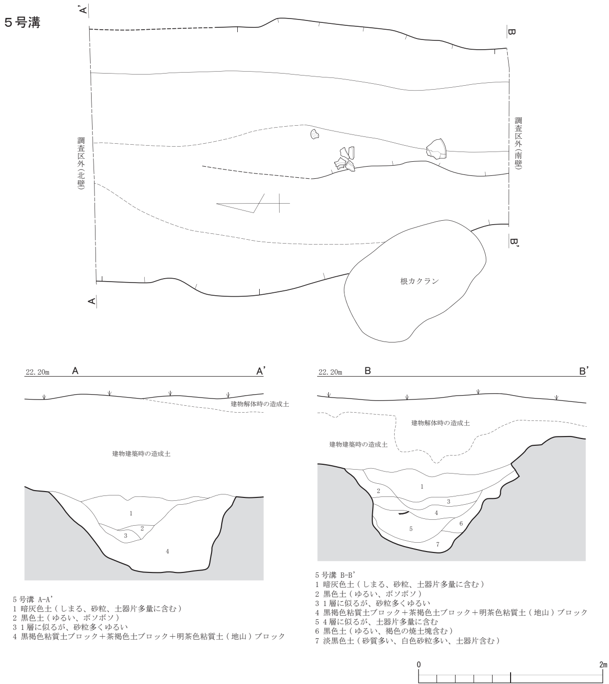
第7図 5号溝実測図 (S = 1 / 40)
