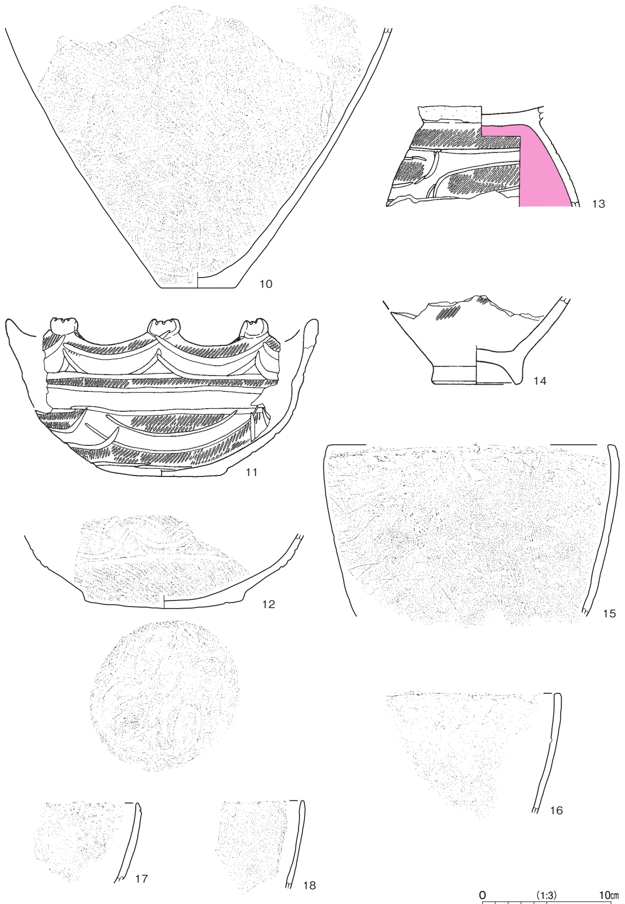
第 109 图 第 1357 号土坑出土遗物实测图 (3)
