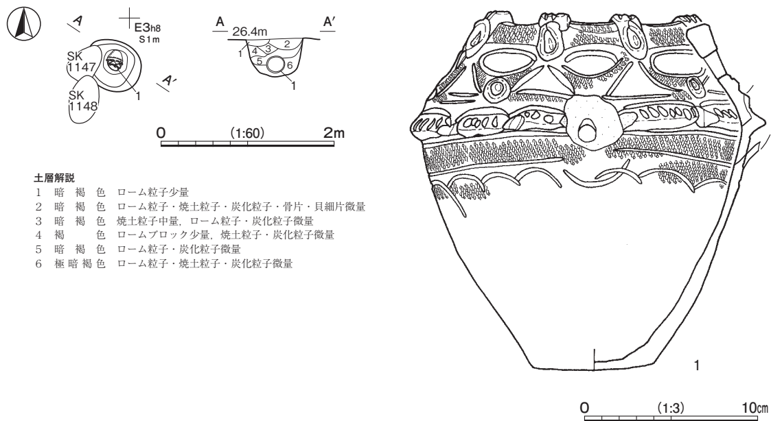
第 91 図 第 1145 号土坑・出土遺物実測図
