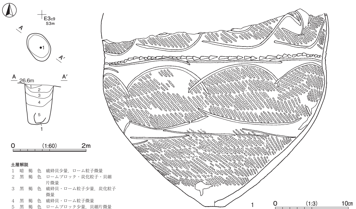
第85図 第891号土坑・出土遺物実測図
