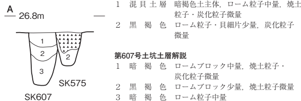
第 170 図 縄文時代土坑実測図 (9)
