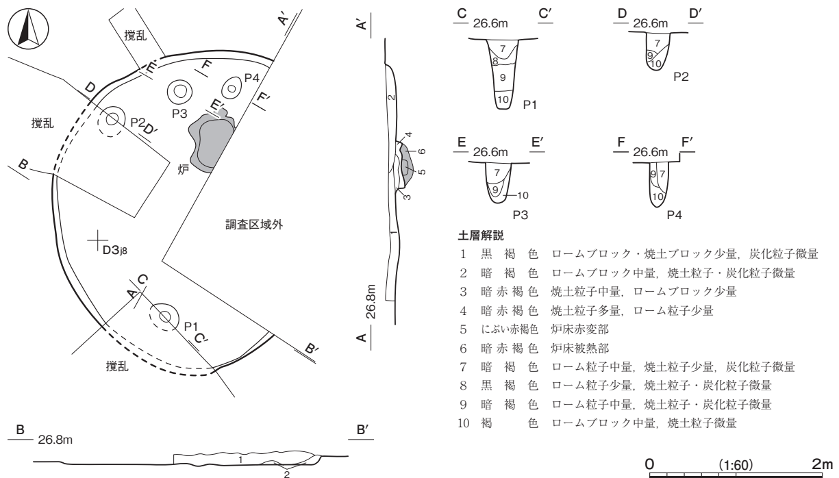
第 24 図 第 24 号竪穴建物跡実測図
