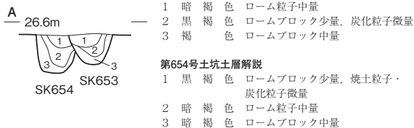
第 174 図 縄文時代土坑実測図 (13)
