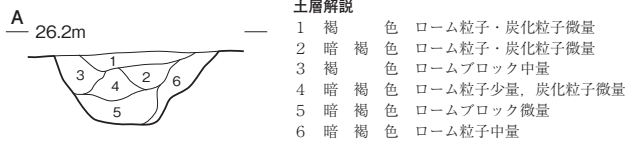
第 194 図 縄文時代土坑実測図 (33)
