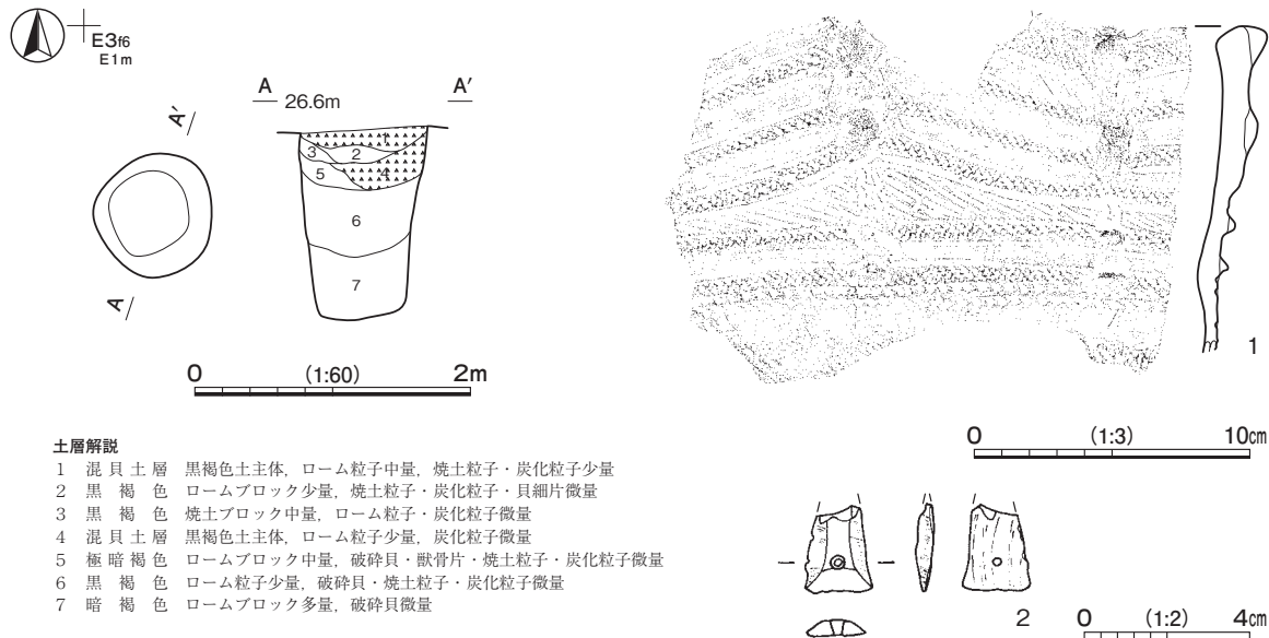
第 82 図 第 816 号土坑・出土遺物実測図
