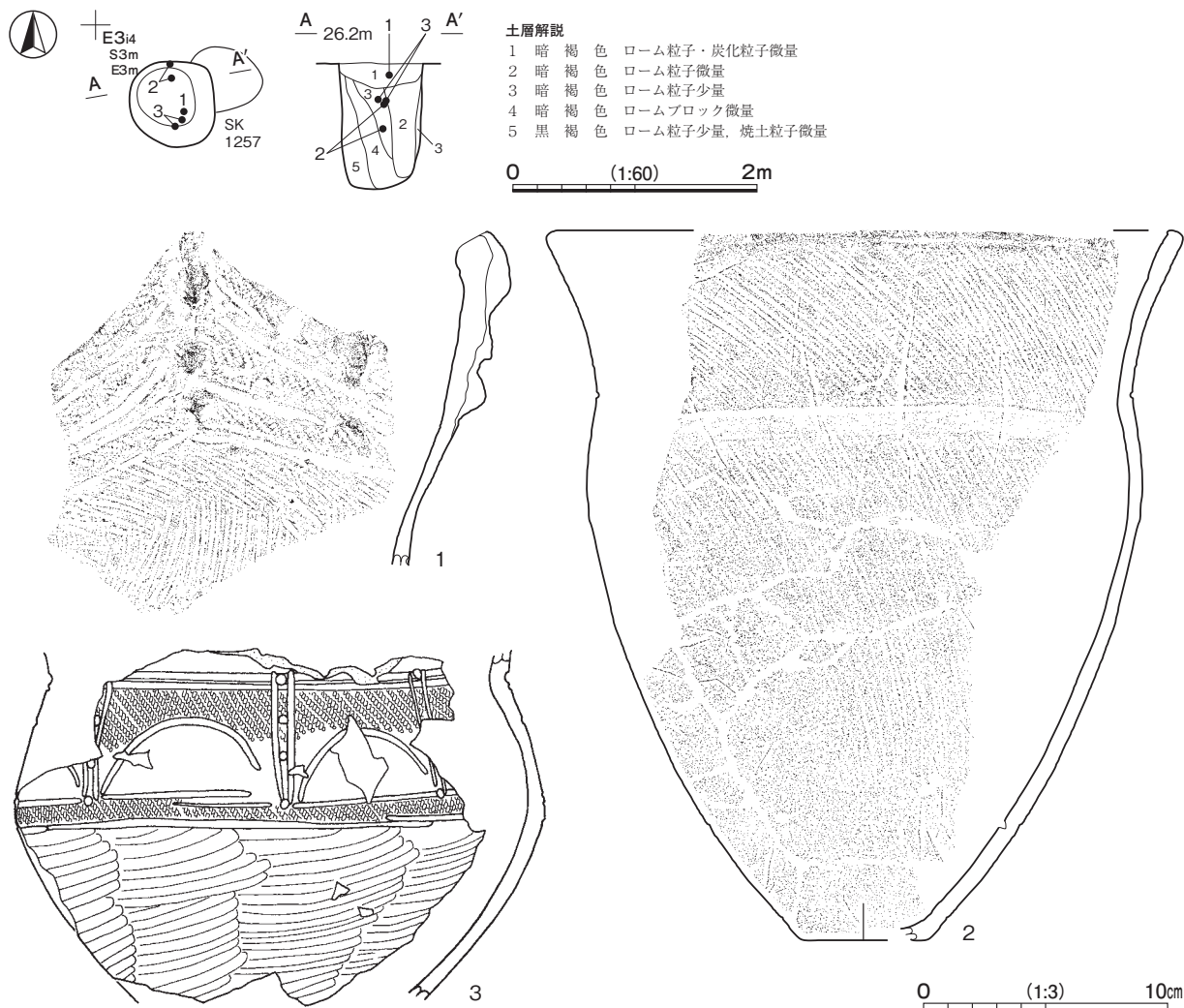
第 92 図 第 1230 号土坑・出土遺物実測図
