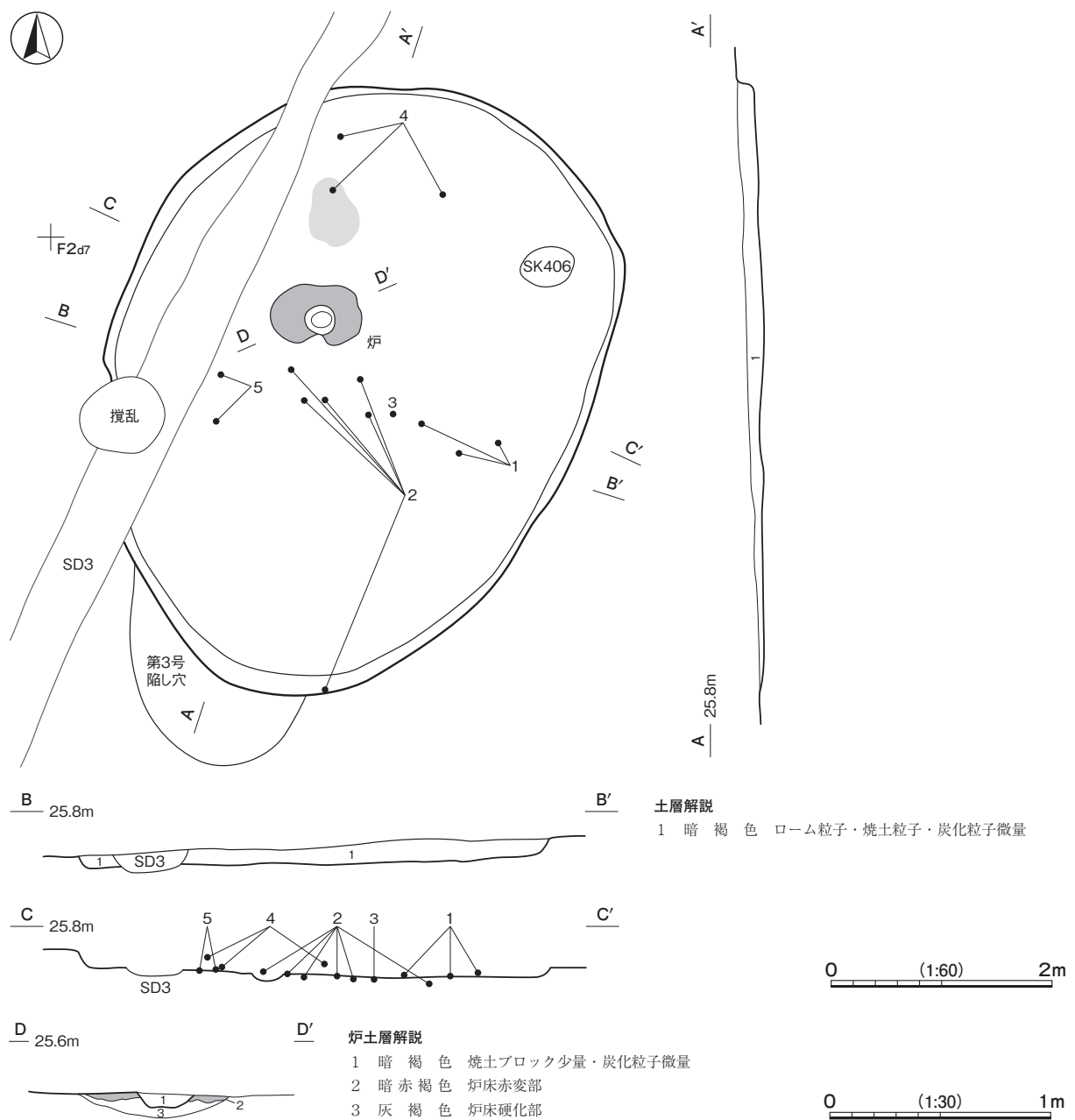
第21図 第23号竪穴建物跡実測図
