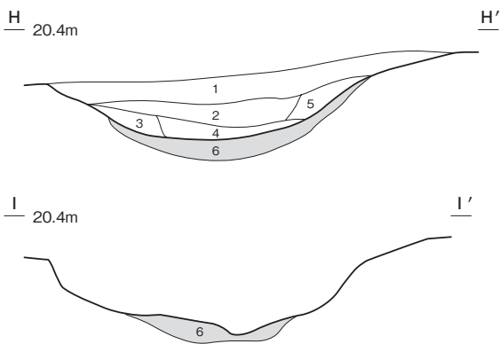
第 52 図 第 32 号竪穴建物跡実測図 (2)
