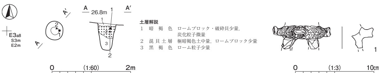
第 67 図 第 495 号土坑・出土遺物実測図
