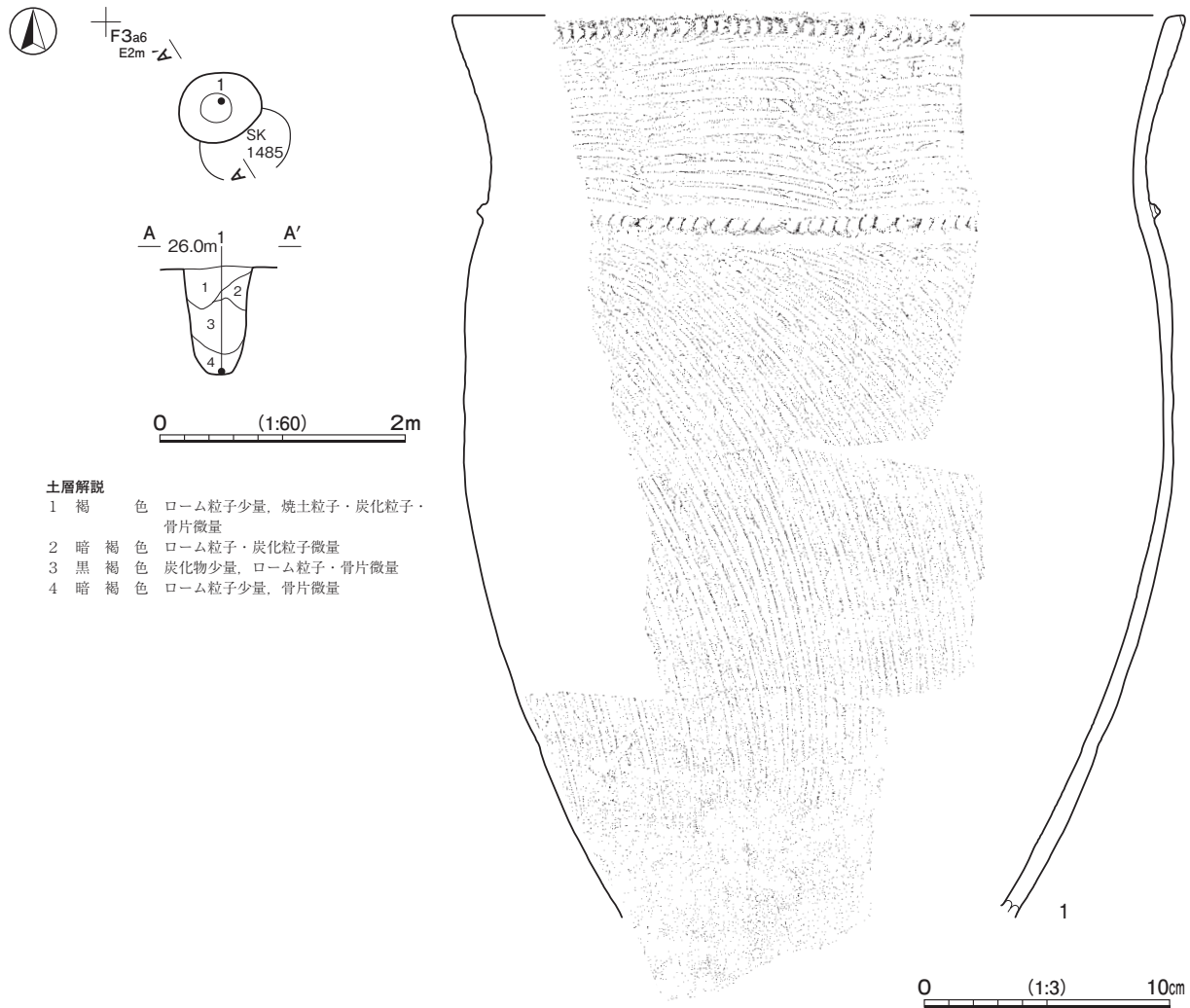
第122図 第1482号土坑・出土遺物実測図
