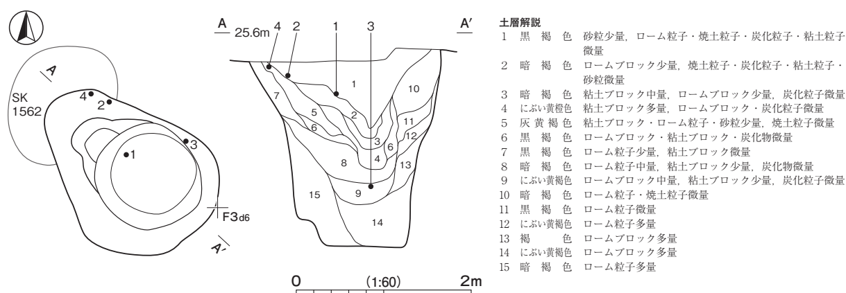
第118図 第1464号土坑実測図
