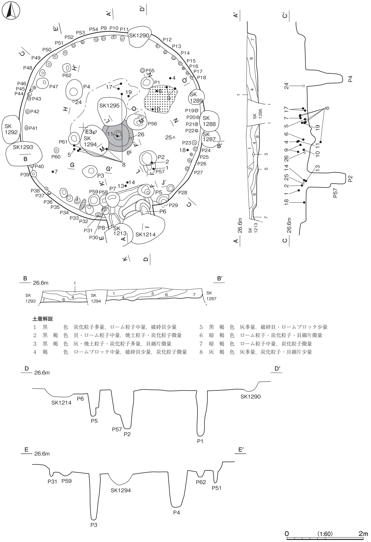
第 26 図 第 25 号竪穴建物跡実測図 (1)
