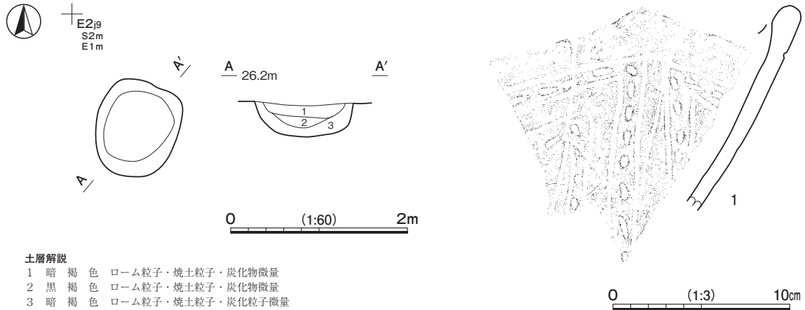
第 59 図 第 363 号土坑・出土遺物実測図
