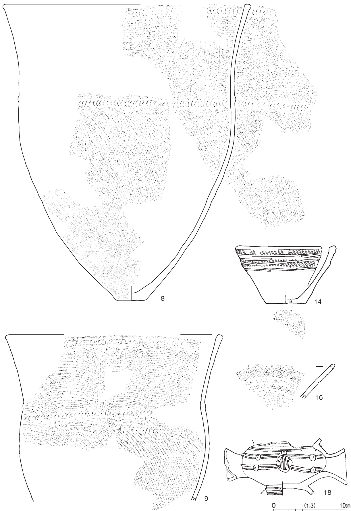
第 29 图 第 25 号竖穴建物跡出土遺物実測图 (2)
