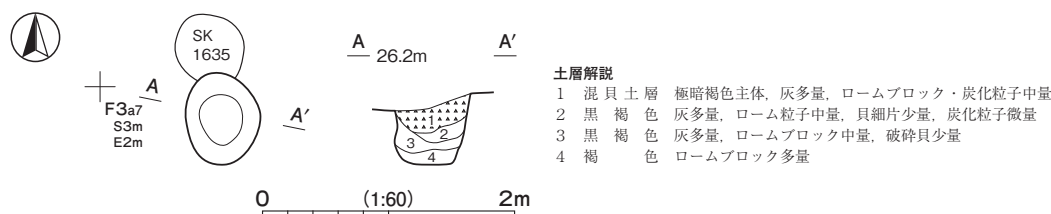
第 142 図 第 1628 号土坑実測図
