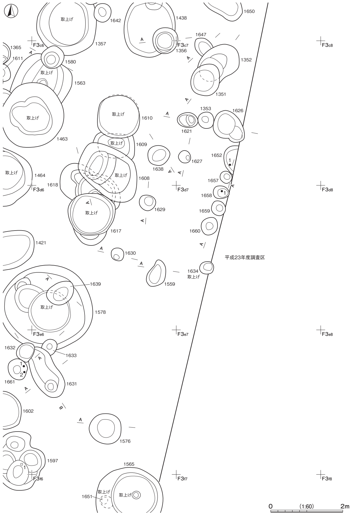
第 160 図 縄文時代土坑⑮区平面図
