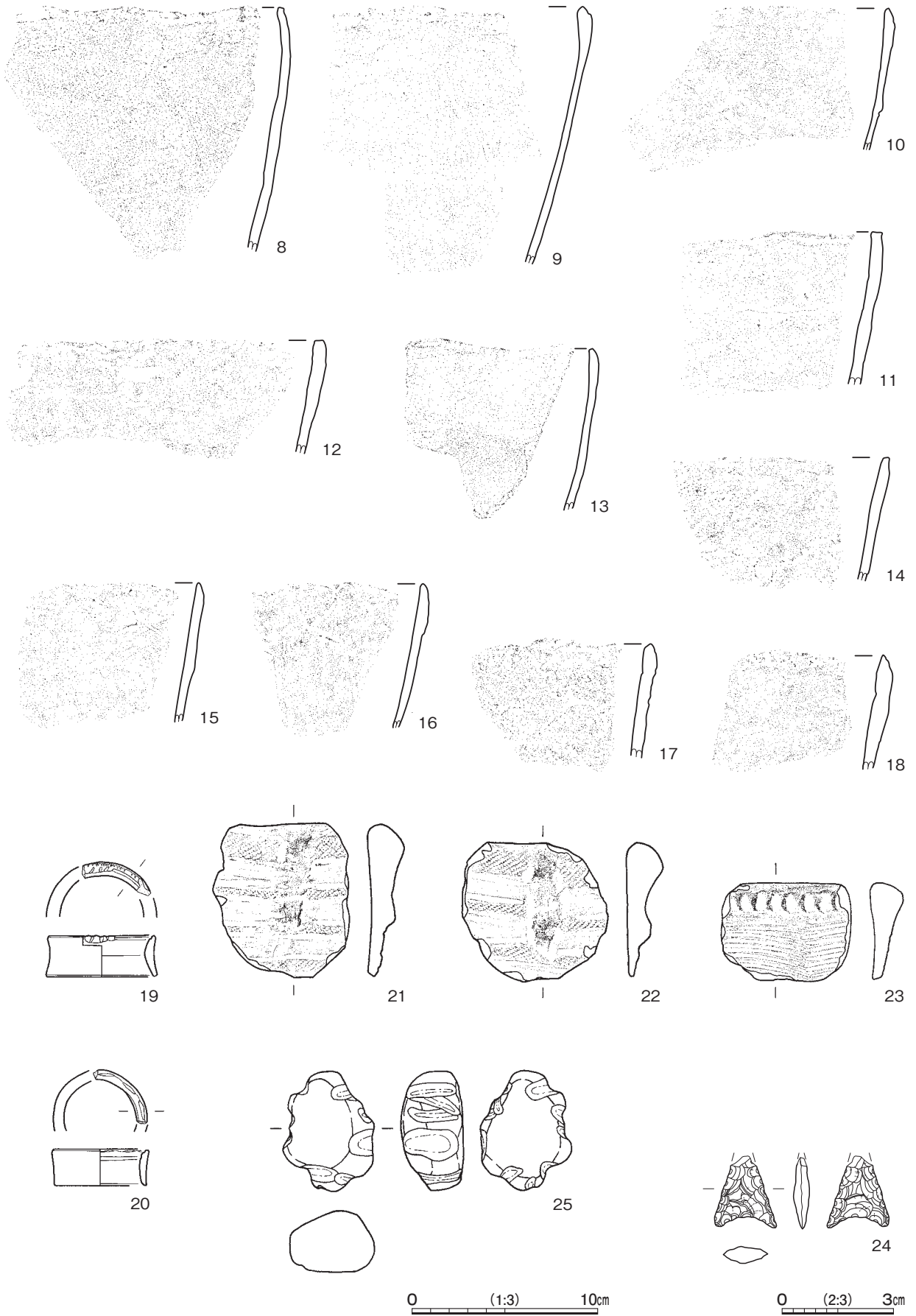
第 99 图 第 1275 号土坑出土遺物実測図 (2)
