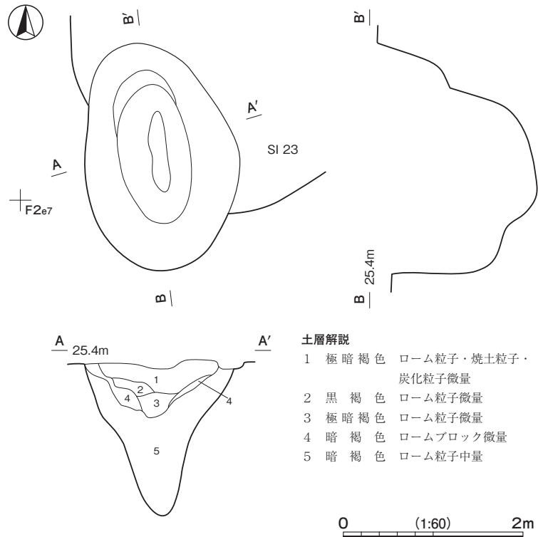
第55図 第3号陥し穴実測図
