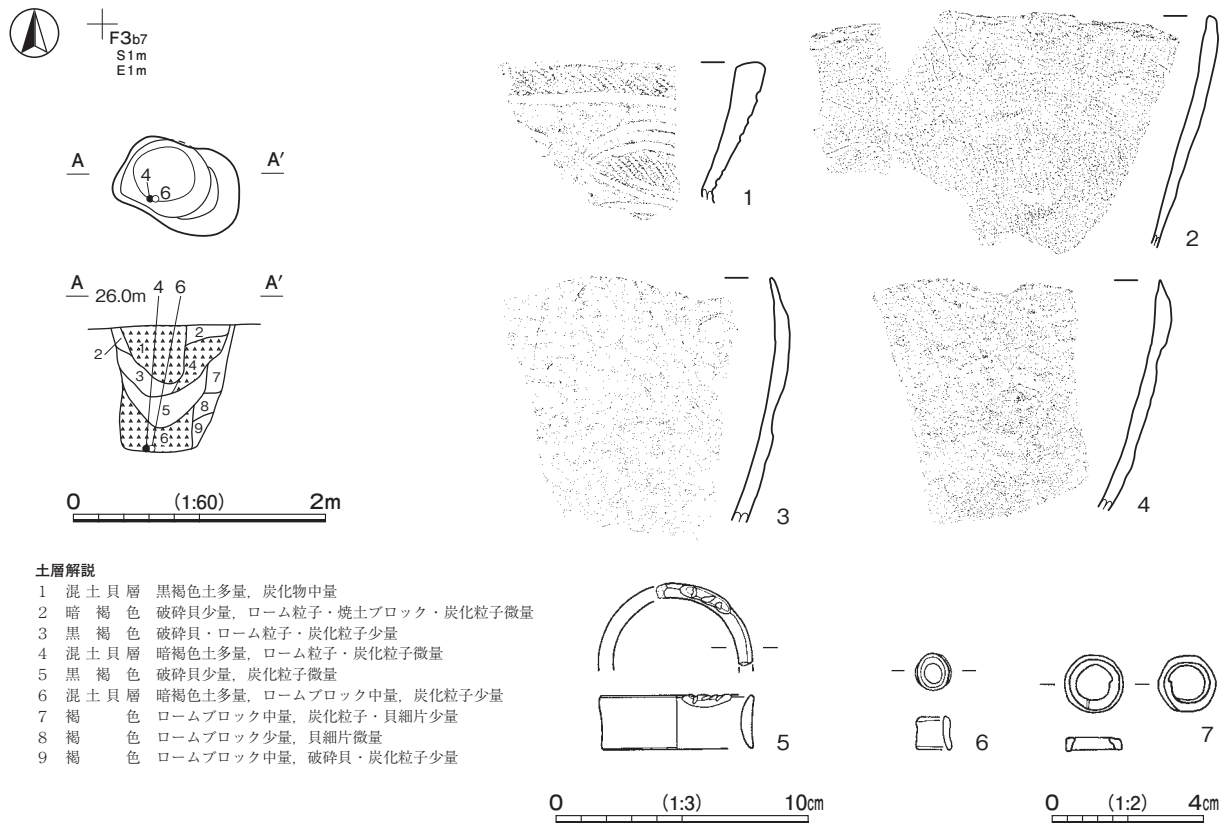
第 137 図 第 1613 号土坑・出土遺物実測図
