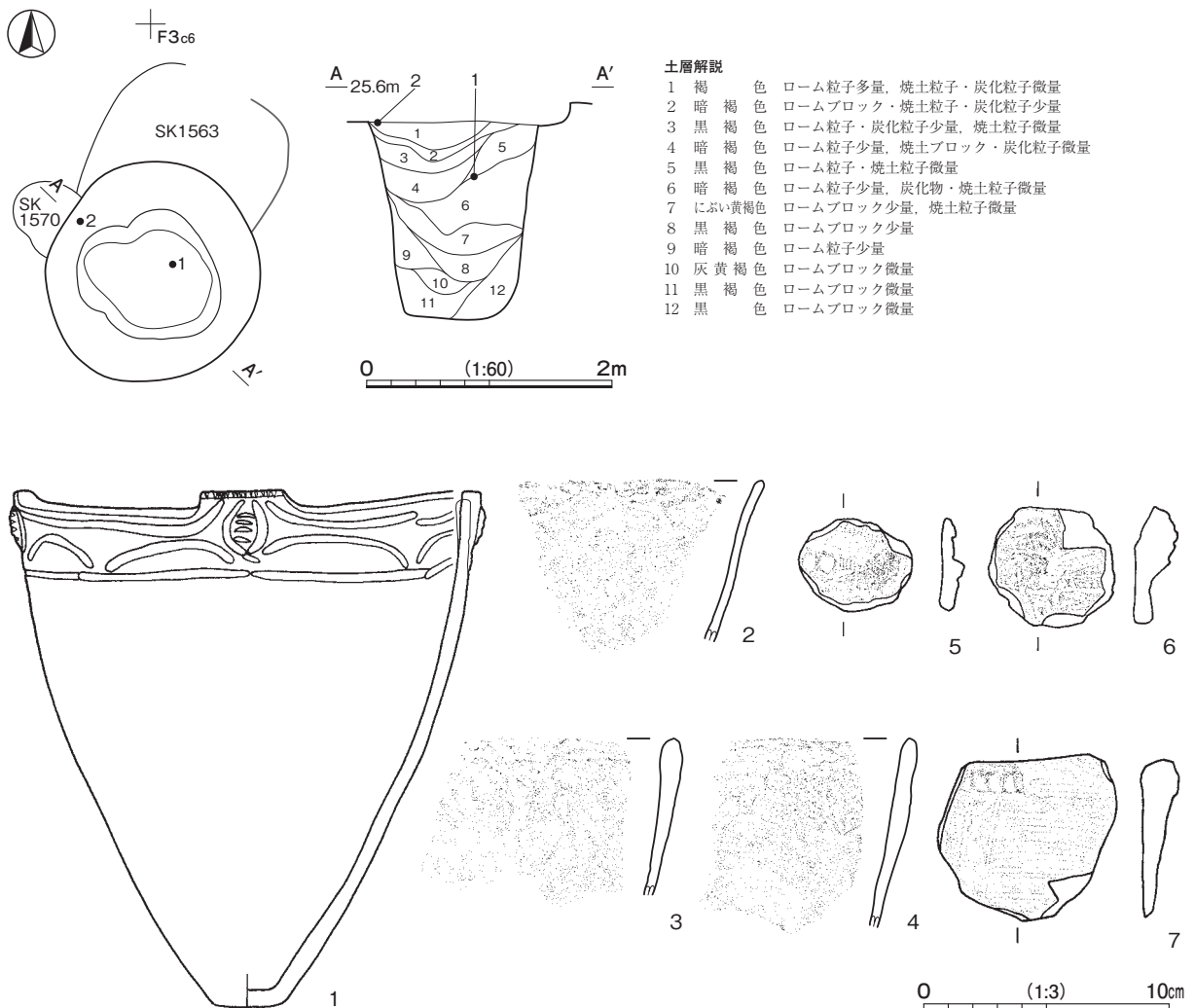
第 117 図 第 1463 号土坑・出土遺物実測図
