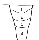
第 169 図 縄文時代土坑実測図 (8)
