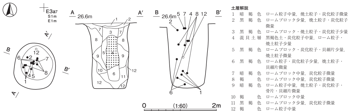
第 65 図 第 491 号土坑実測図
