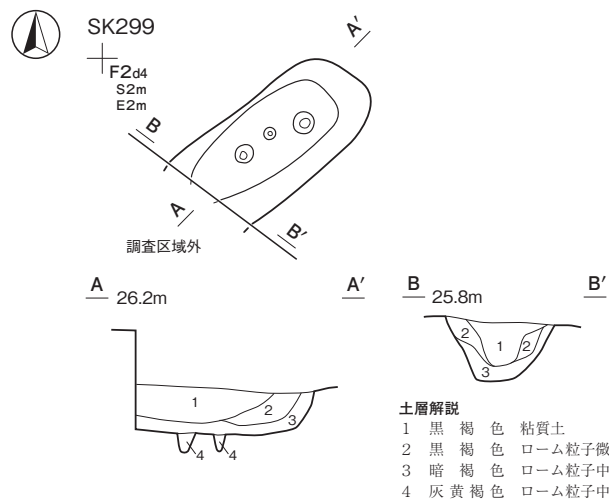
第 216 図 縄文時代土坑実測図 (55)
