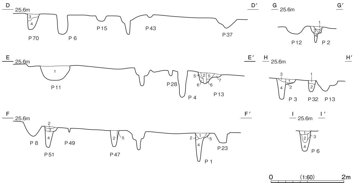
第43図 第28号竪穴建物跡実測図(1)
