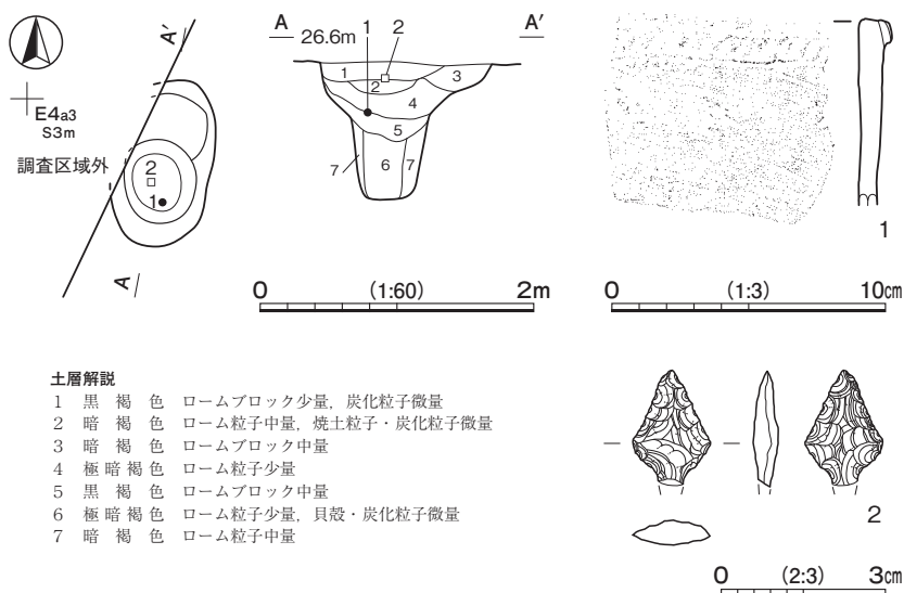
第 70 図 第 688 号土坑・出土遺物実測図
