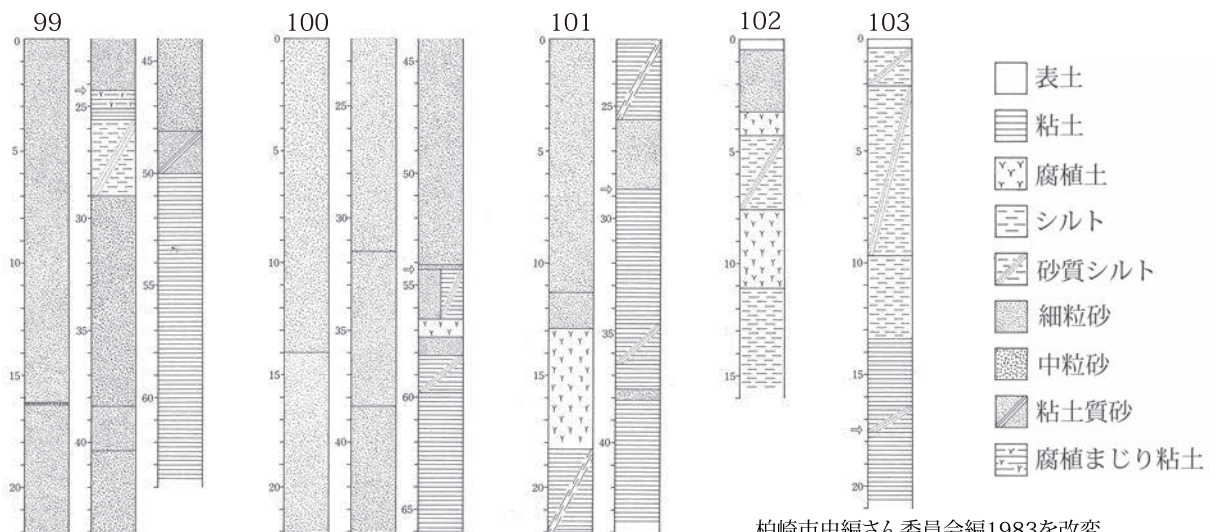
第5図 西岩野遺跡の周辺の地形と地質柱状図
