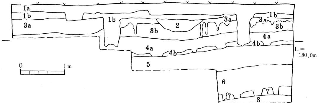
第8図 2トレンチ土層断面図
