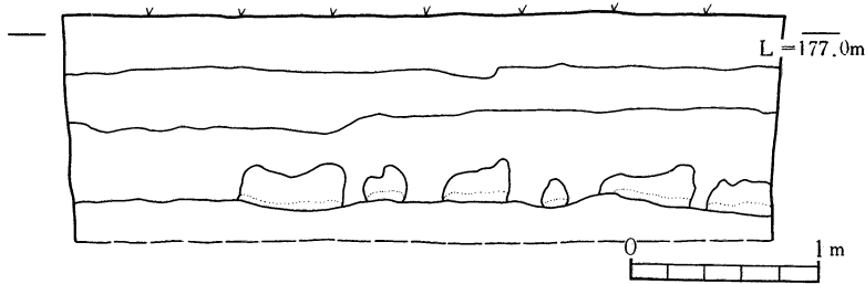
第46図 14トレンチ断面図
