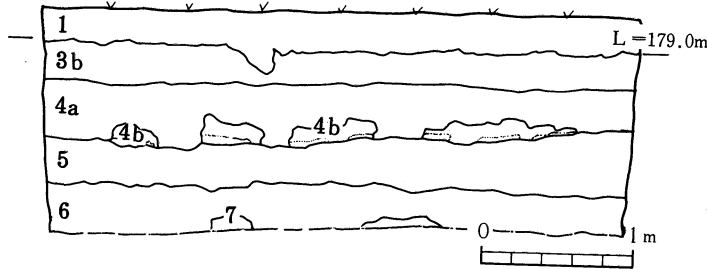
第20図 10トレンチ土層断面図
