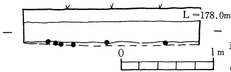
第34図 5 トレンチ平・断面図
