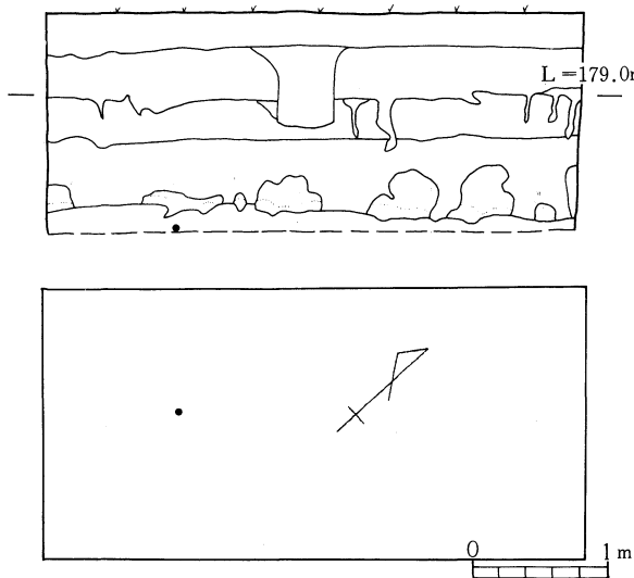
第40図 8トレンチ平・断面図
