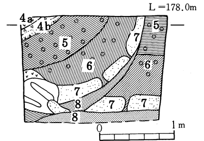
第7図 局部断層断面図
