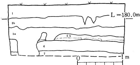
第11図 4 トレンチ断面図
