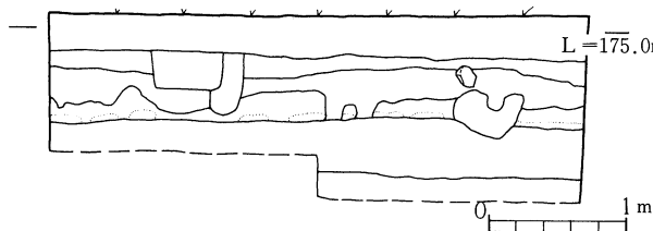
第41図 9トレンチ断面図
