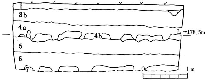
第19図 9トレンチ土層断面図
