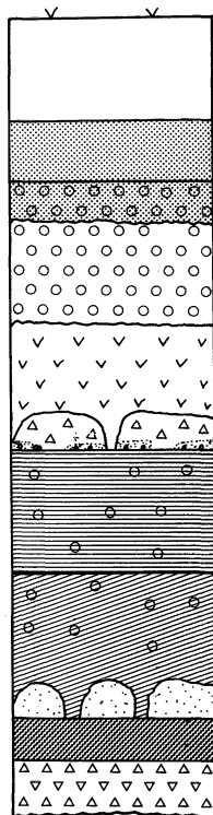
第4図 土層模式柱状図 6層：黒褐色腐植土層。径5mm前後の黄橙色軽石および青灰色の安山
