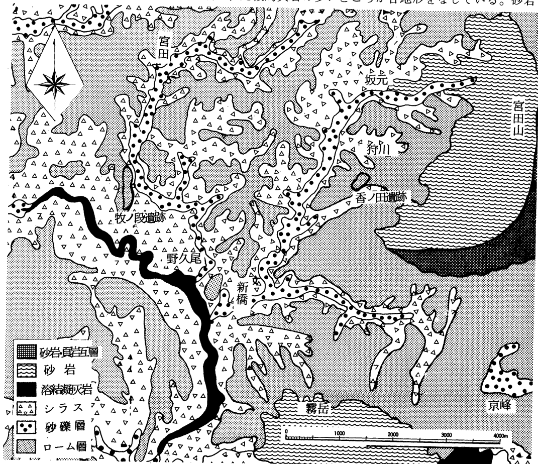
第1図 遺跡周辺の表層地質図 (土地分類基本調査—末吉—1974 原図)
