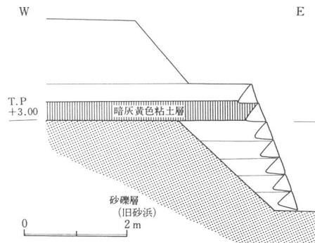
第23図 台場土手推定復元図
