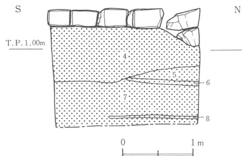
第9図 石垣下土層断面図
