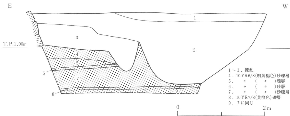
第10図 石垣前面部土層断面図
