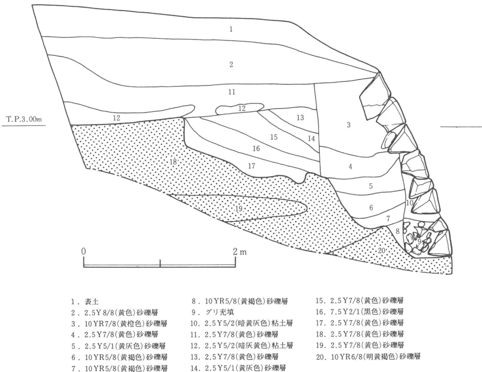
第12図 石垣背面断面図
