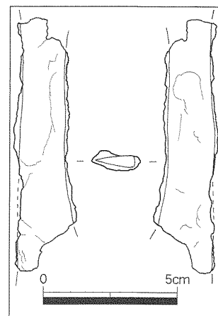
図2 不明鉄製品
