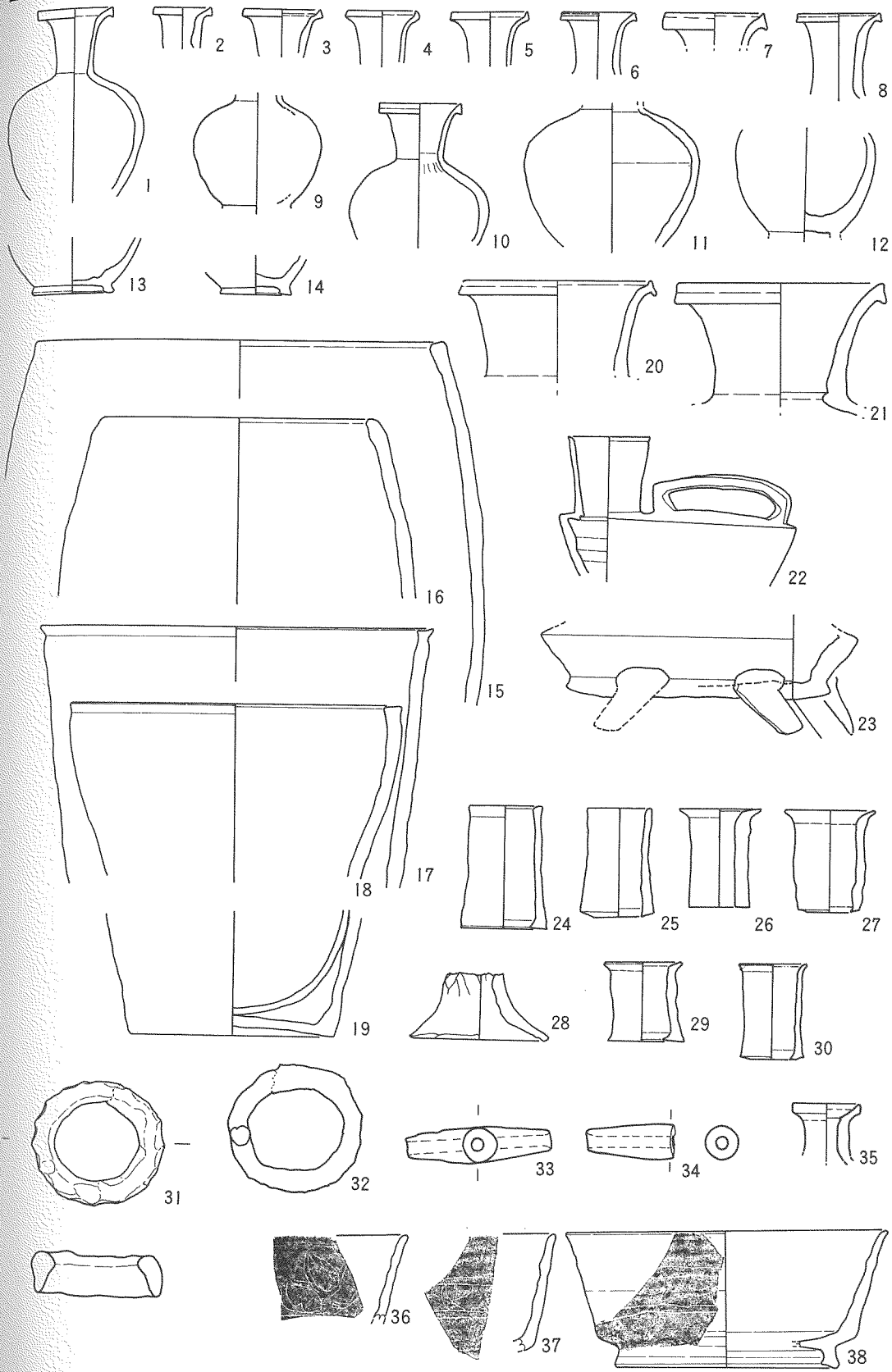
圖版 XI 小型長頸瓶・平瓶・土鍾・特殊品・窯道具等 (33~35 1/2・36~38 1/3) 1 : 4
