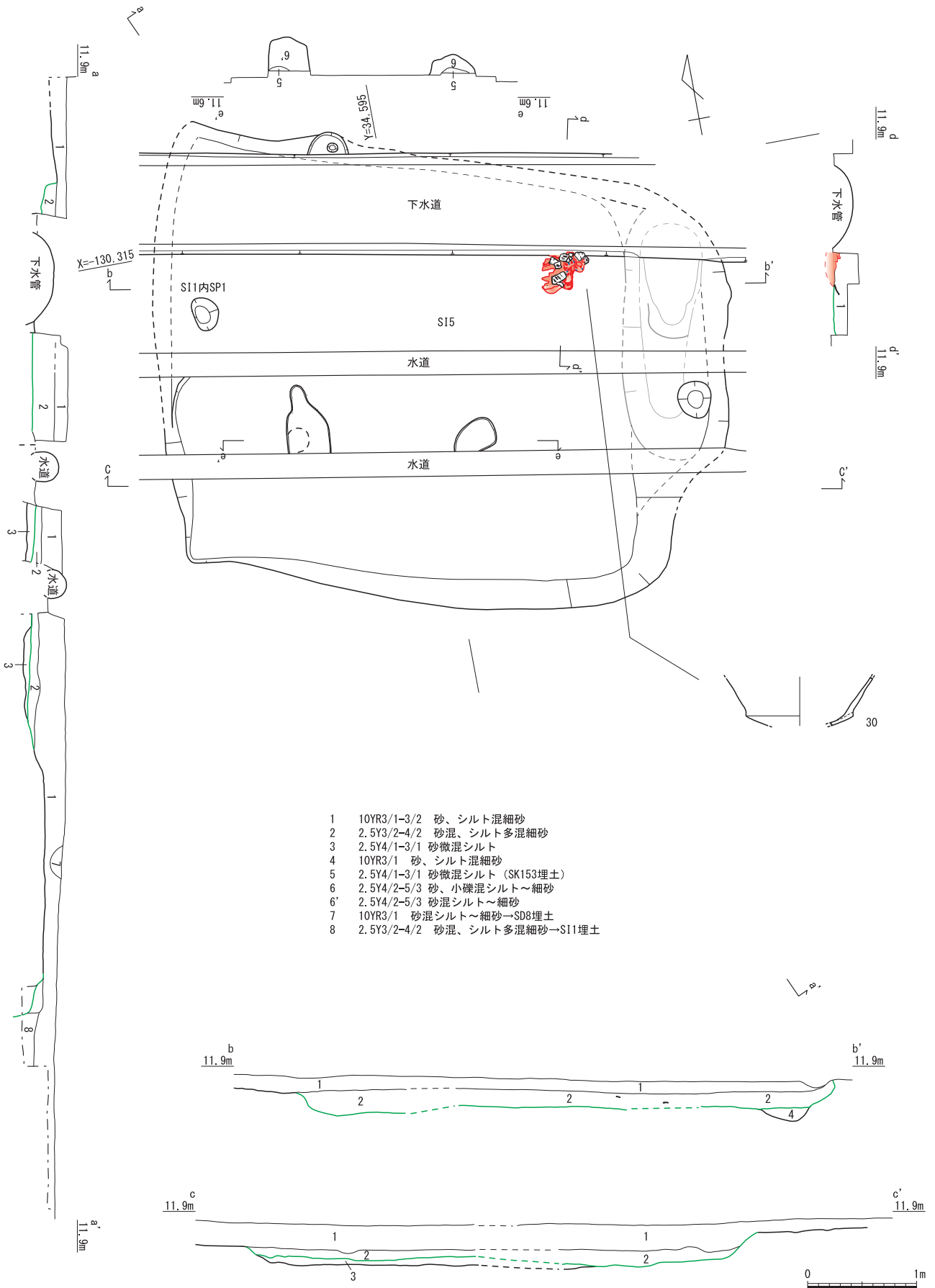
図14 SI5詳細図 S=1 : 50
