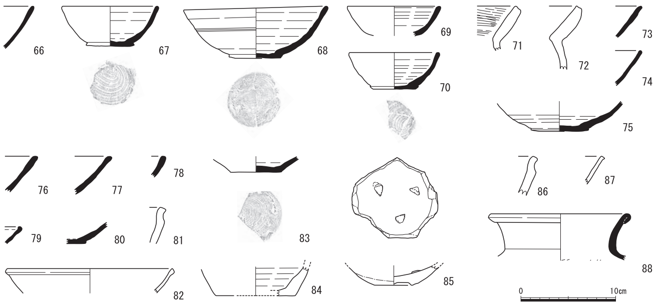
図23 出土遺物実測図4 S=1:4 (65 SD7 66 SP10 67 SP15 68 SP17 69, 70 SP18 71~75 SK5 76~83 SD4-2 84, 85 SD4-1 86 SD1 87 SD3 88 検出中)
