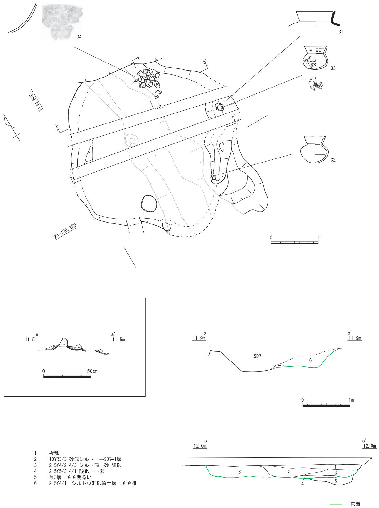
図15 SI6詳細図 S=1:50・S=1:25
