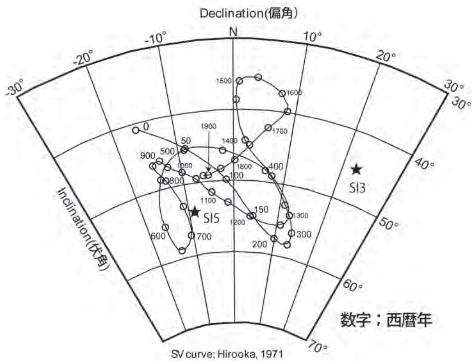
挿図2 焼土範囲(SI3及びSI5)の平均方向と考古地磁気の標準曲線との対比
