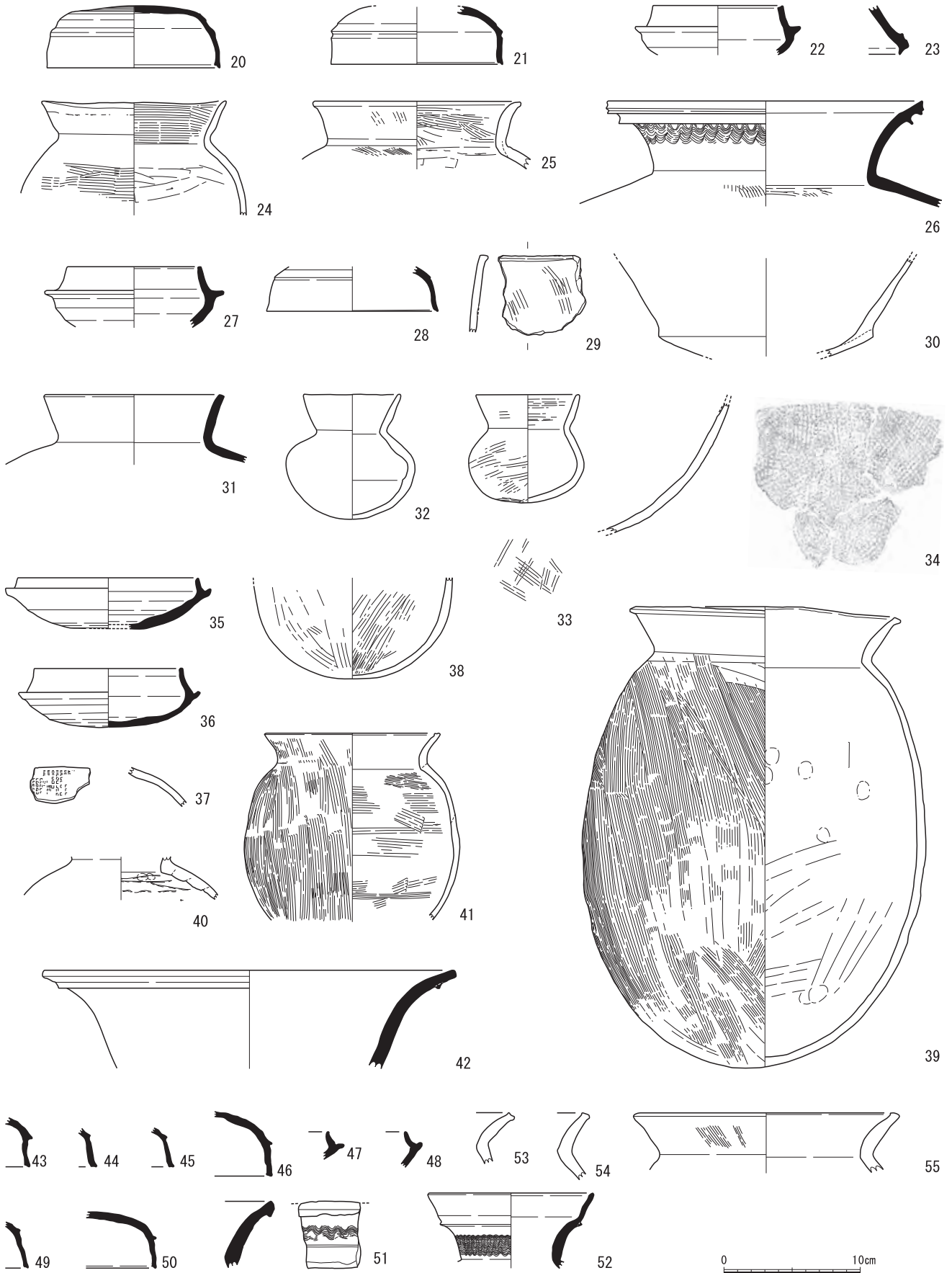
图21 出土遺物実測図2 S=1:4 (20~26 SI4 27~30 SI5 31~34 SI6 35~39 SK7 40 SK16 41 SK17 42 SK18 43~55 SD7)
