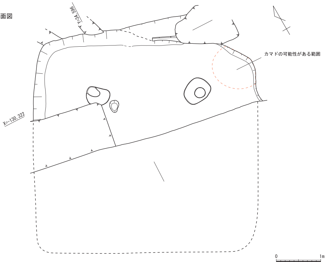
図6 SI1詳細図1 S=1 : 50
