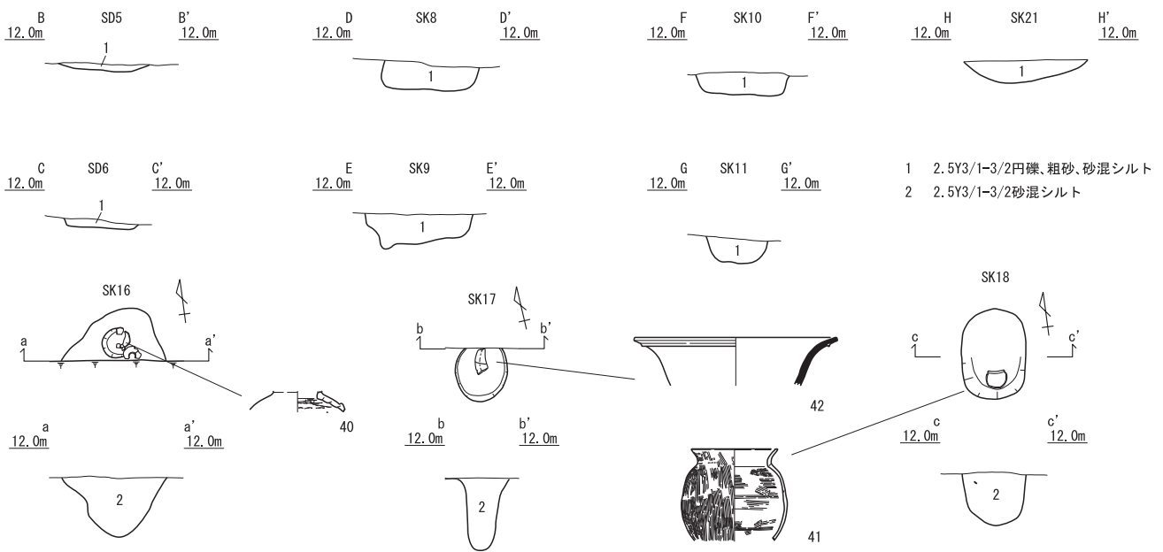
図18 SD・SK断面図及び詳細図（下層） S=1 : 50 ※SD5~SK11の平面図は、図4に掲載
