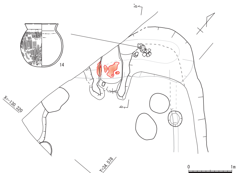
図8 SI2詳細図1 S=1 : 50
