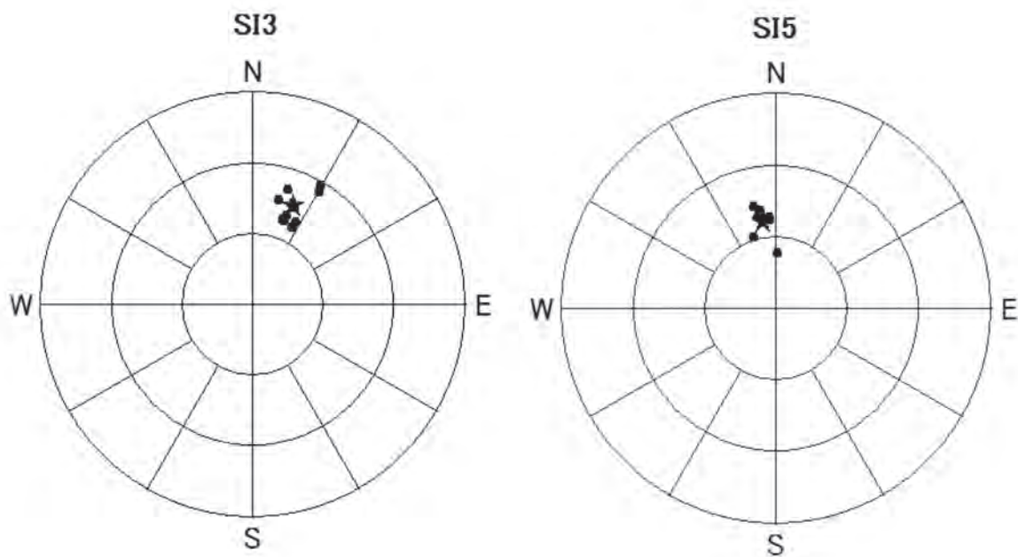
挿図1 焼土(SI3及びSI5)それぞれで採取した土壌試料の、交流消磁後の残留磁化方向(●)及び平均方向(★)
