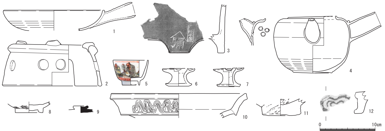
図5 遺物実測図 (S=1:4)
