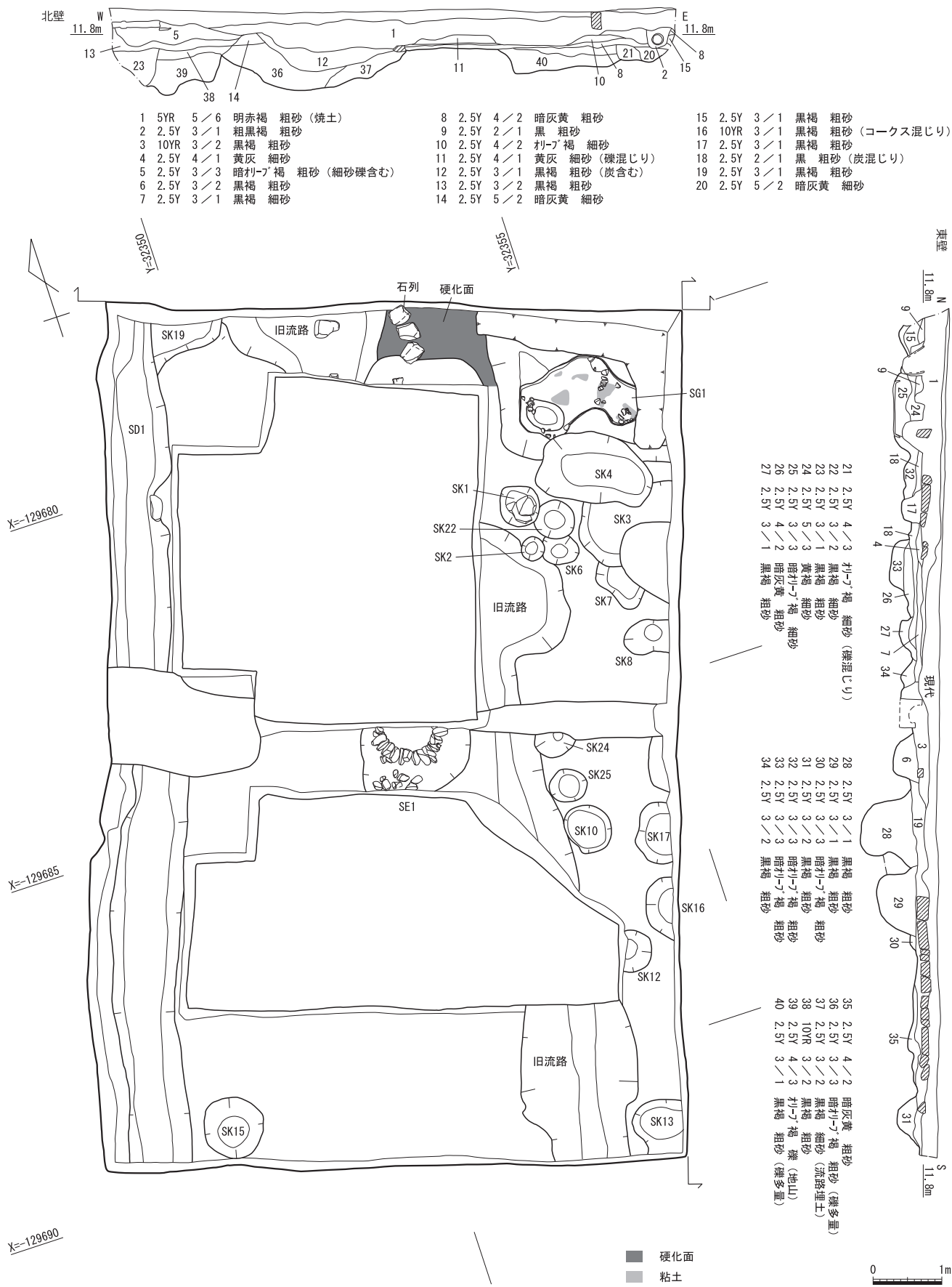
図3 第1・2面平面図・断面図 (S=1:80)
