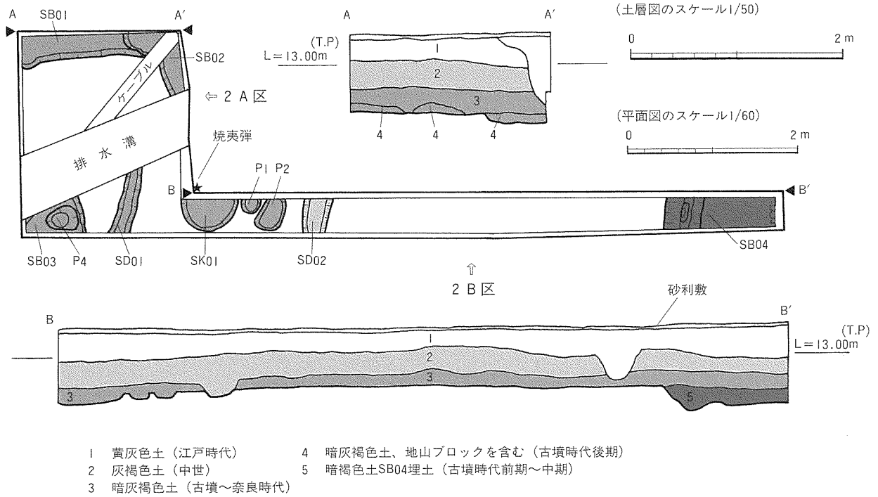
図6 2区 平面図および土層断面図
