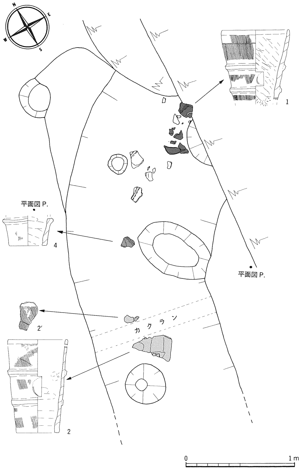
第 13 図 SD 17 埴輪出土状況
