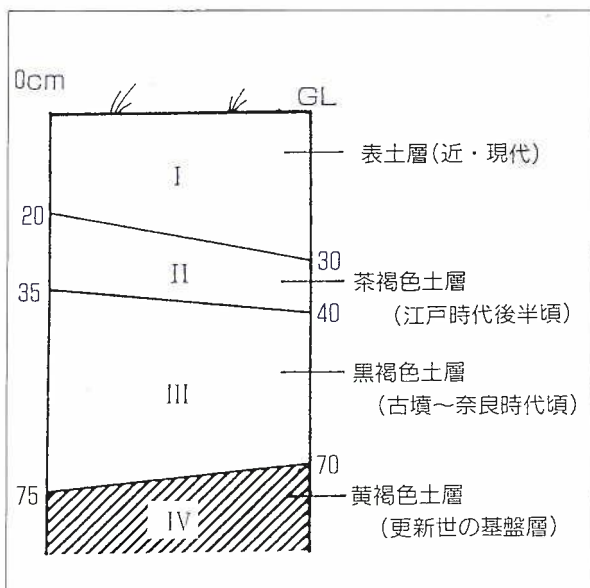
図3 土層模式図
