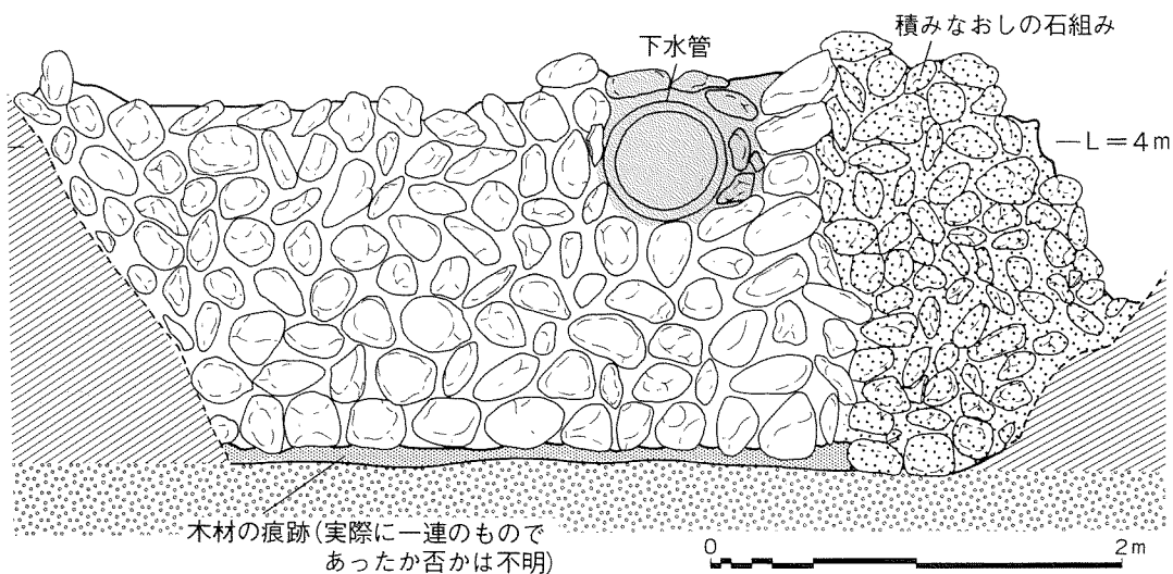
第5図 旧紫川石組み側面図 (1 : 40)
