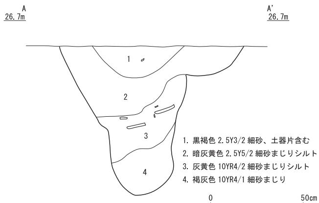
図3 SD2土層断面図 (S=1:20)
