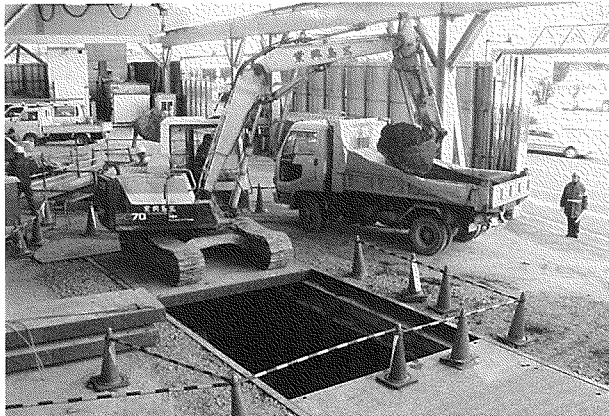
写真5 排土の搬出状況（東から）
