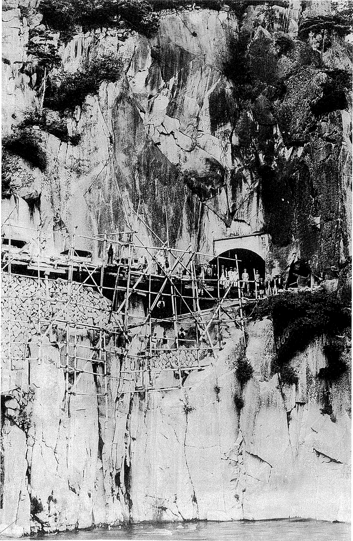
綾戸隧道(手前)と綾戸穴道(右奥) 昭和4年 生方稷衛氏 提供
