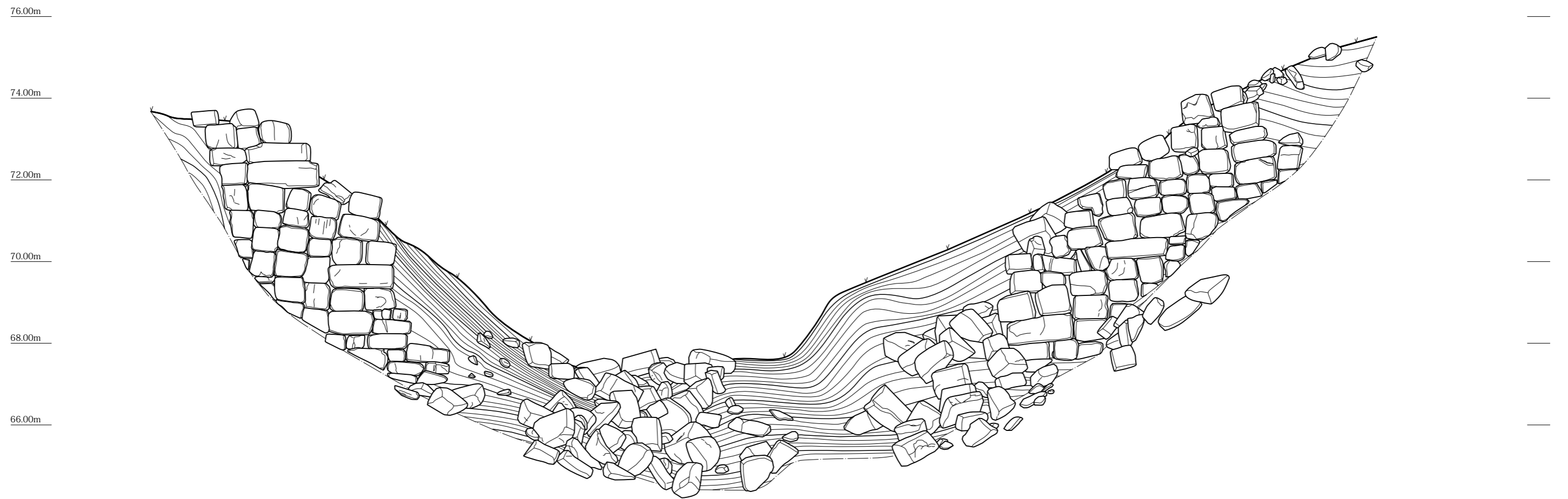
第 11 圖 西門跡前面石壘立面圖 (1/100)
