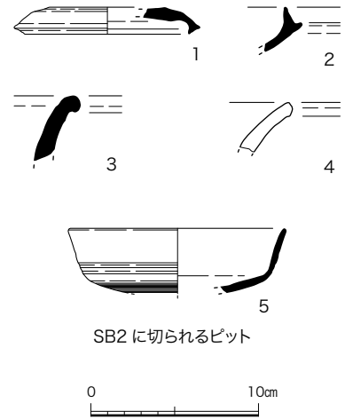
図9 SB2 出土遺物実測図 (1/4)
