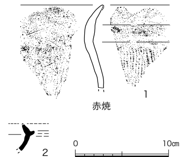
図30 SD8 出土遺物実測図(1/4)
