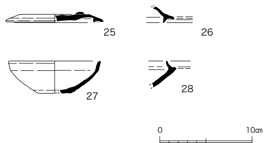
図 23 SE3 出土遺物実測図 (1/4)
