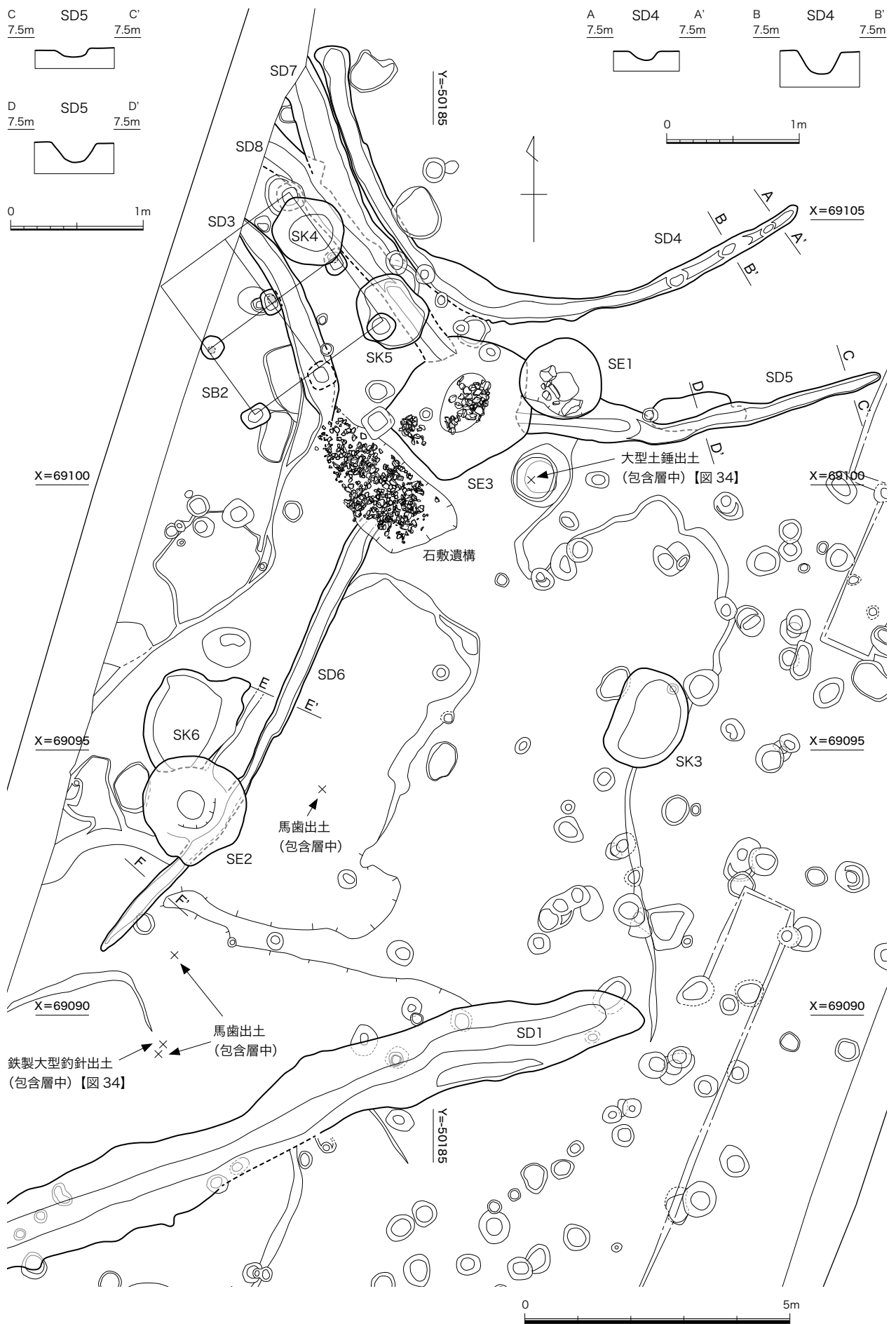
図 18 石敷遺構周辺平面図 (1/100)、SD4、SD5 断面図 (1/40)
