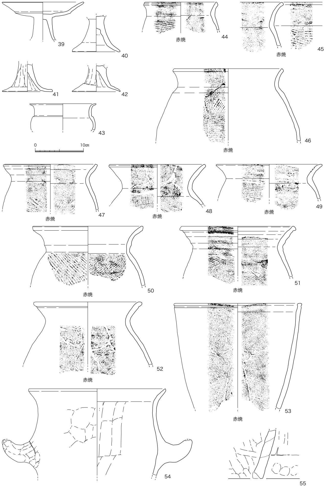
図33 包含層出土遺物実測図(1/4)
