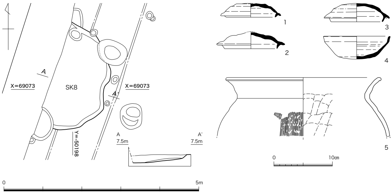
図17 SK8 平面図、断面図 (1/60)、出土遺物実測図 (1/4)
