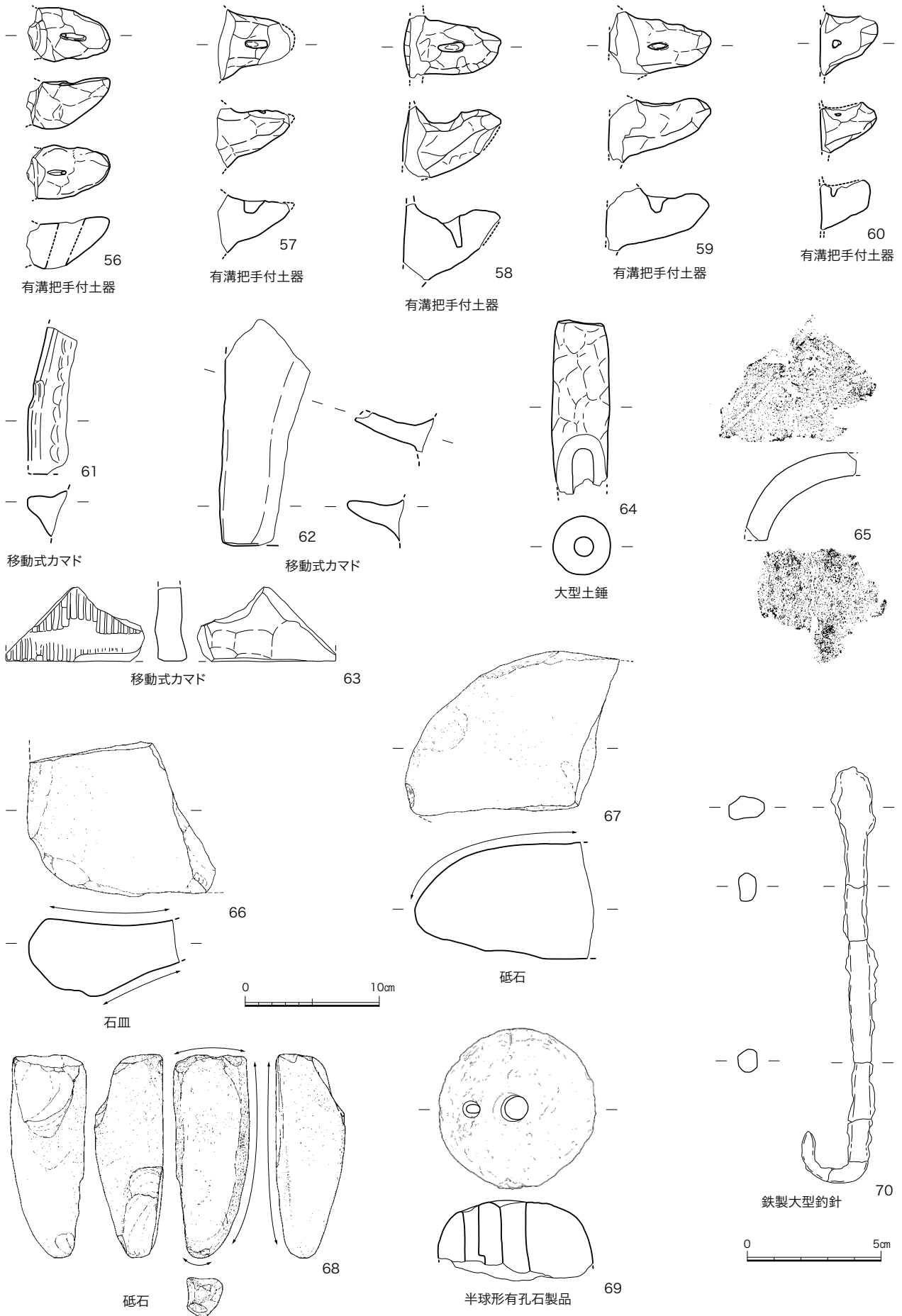
図 34 包含層出土遺物実測図 (1/4、鉄製品 1/2)
