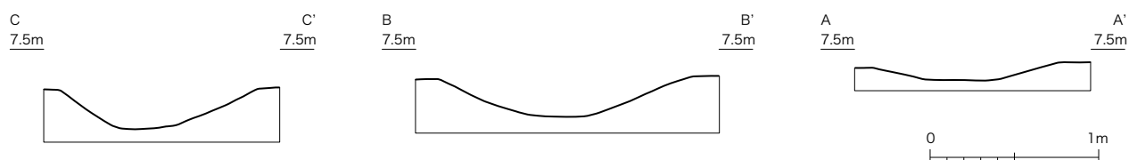
図 26 SD1 平面図 (1/100)、断面図 (1/40)
