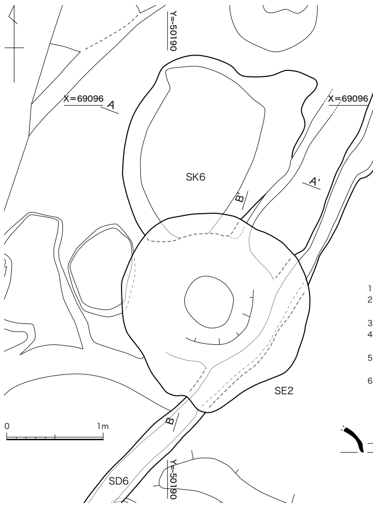
図14 SK6、SE2平面図、断面図(1/40)
