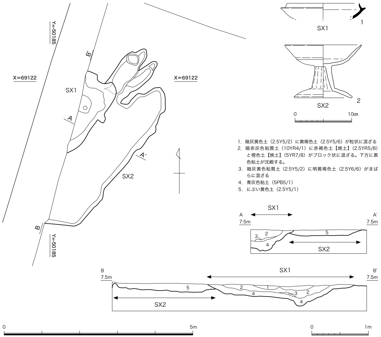
図 31 SX1、SX2 平面図 (1/60)、断面図 (1/40)、出土遺物実測図 (1/4)
