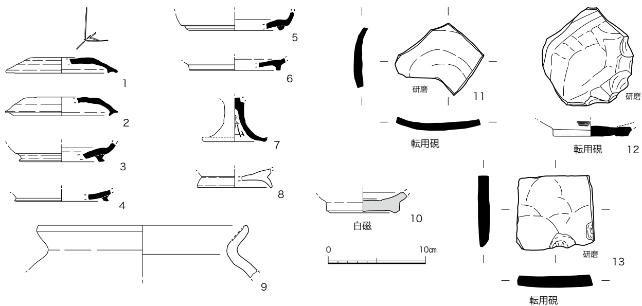
図 27 SD1 出土遺物実測図 (1/4)
