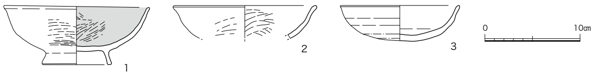
図 11 SK2 平面図、断面図 (1/40)、出土遺物実測図 (1/4)
