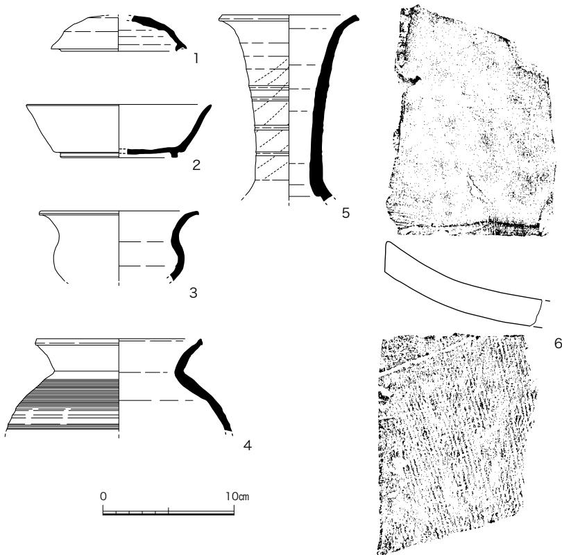
図20 SE1 出土遺物実測図 (1/4)
