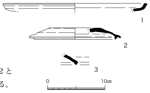
図16 SE2出土遺物実測図(1/4)
