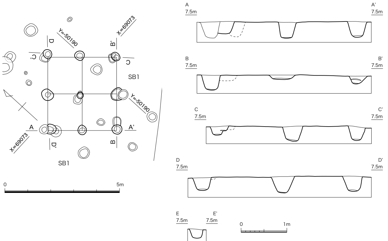
図6 SB1 平面図 (1/100)、断面図 (1/50)
