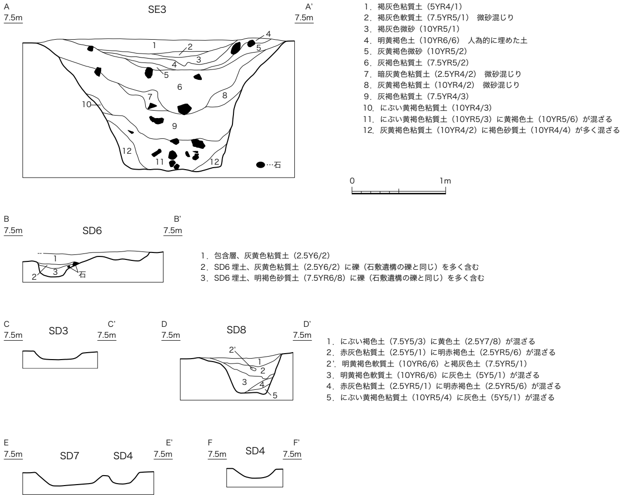
図22 SE3、SD3、SD4、SD6、SD7、SD8断面図 (1/40)
