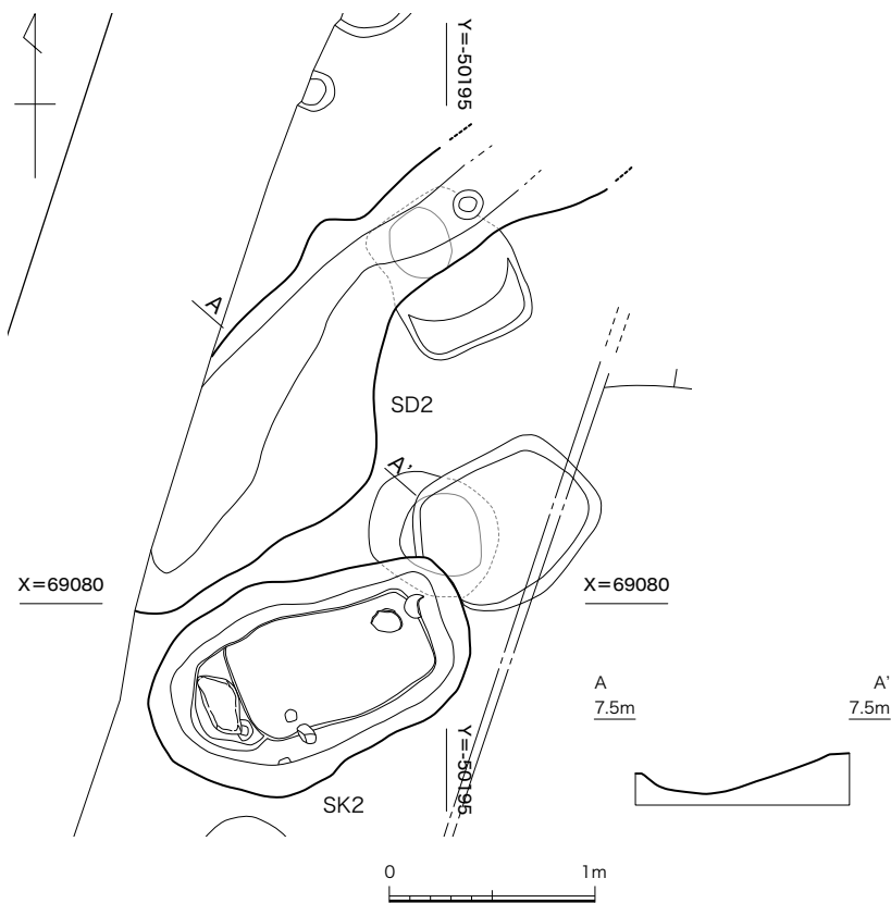
図28 SD2 平面図、断面図(1/40)
