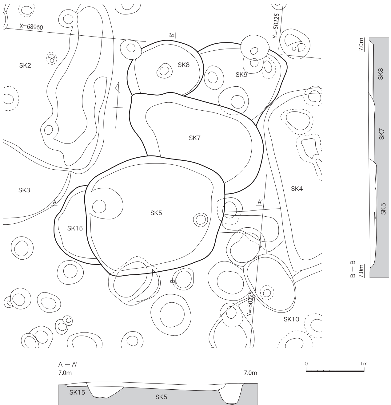
図11 SK5、7、8、9、15平面図、断面図(1/40)
