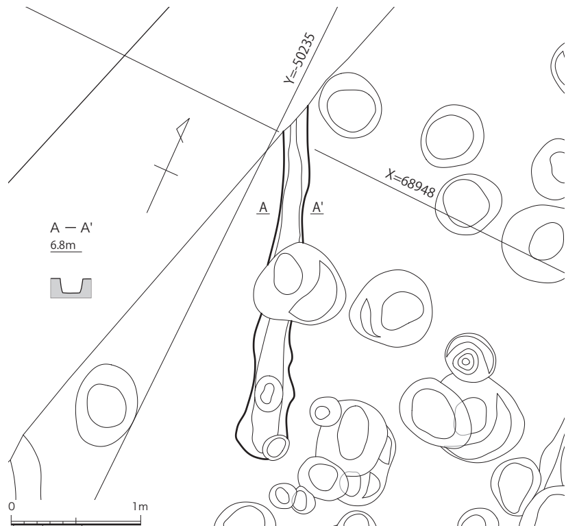
図 24 SD3 平面図、断面図(1/40)
