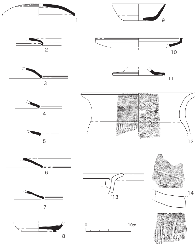
図12 SK5 出土遺物実測図 (1/4)
