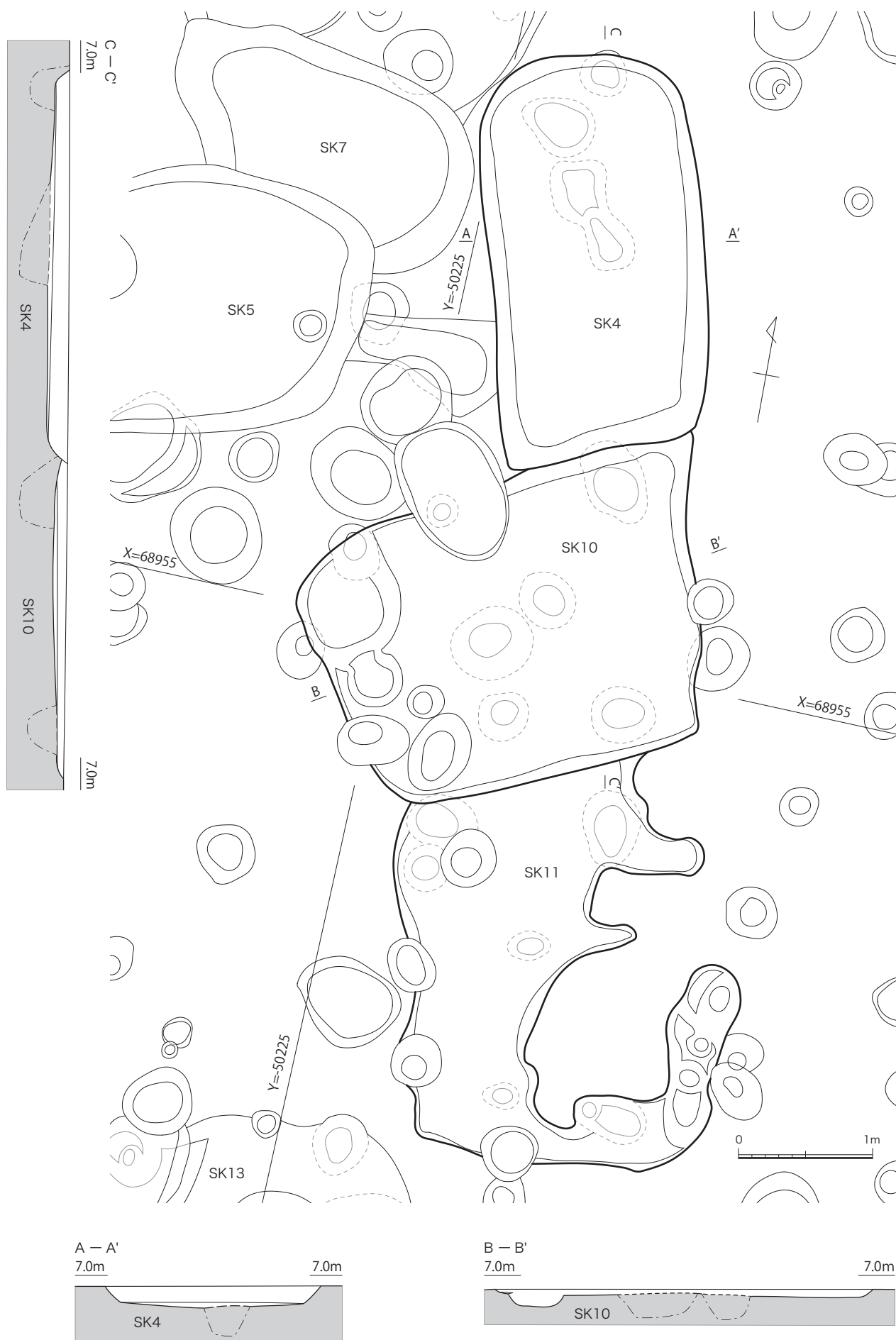
图9 SK4、10、11 平面图、断面图(1/40)
