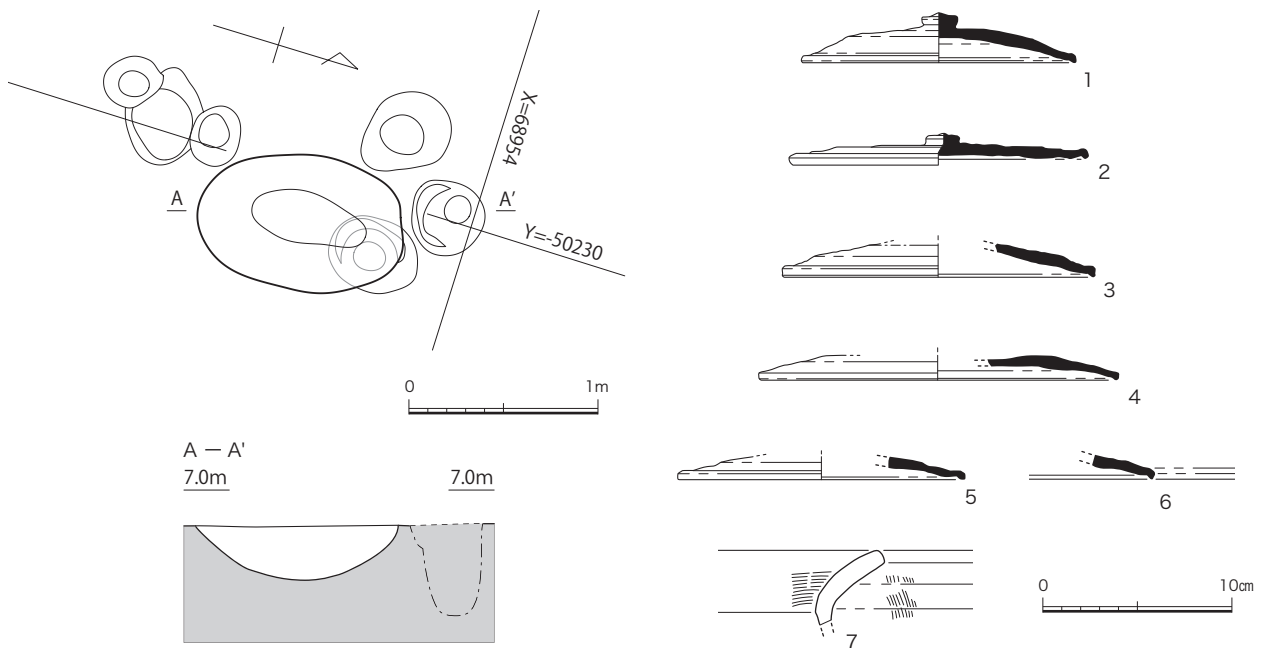
図13 SK6平面図、断面図(1/40)、出土遺物実測図(1/4)
