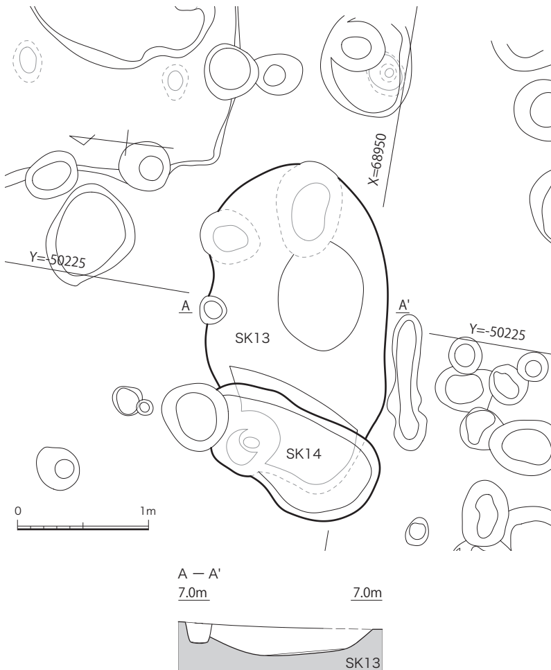
図18 SK13、SK14平面図、断面図(1/40)
