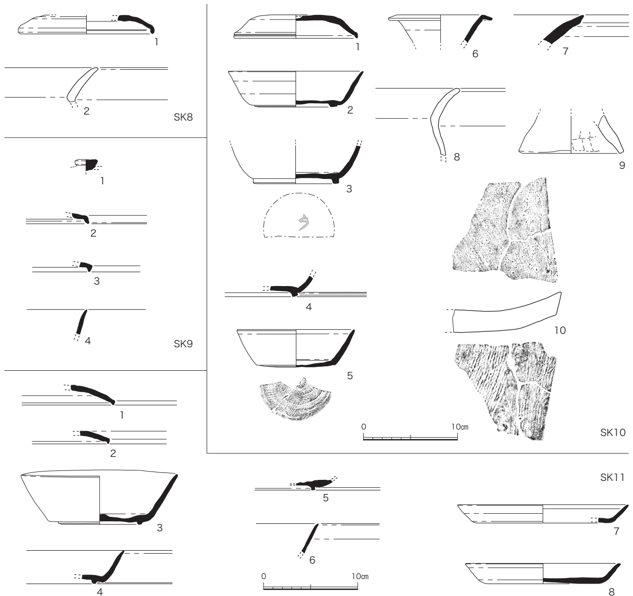
図 15 SK8、9、10、11 出土遺物実測図(1/4)
