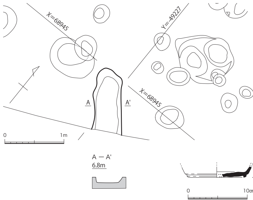
図22 SD1 平面図、断面図 (1/40)、出土遺物実測図 (1/4)
