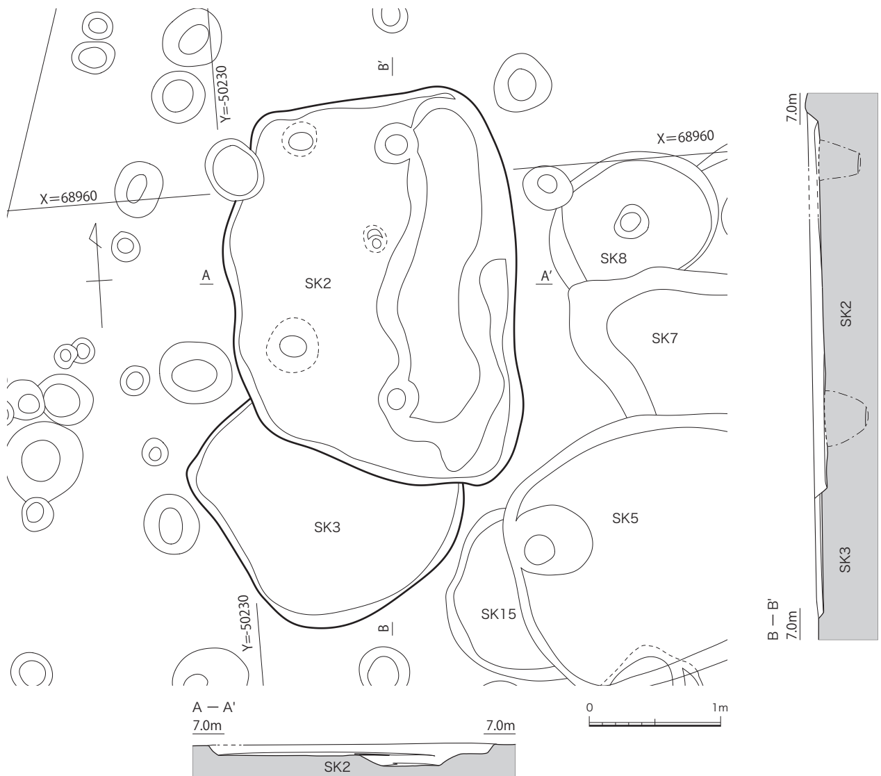
図7 SK2,3平面図、断面図(1/40)
