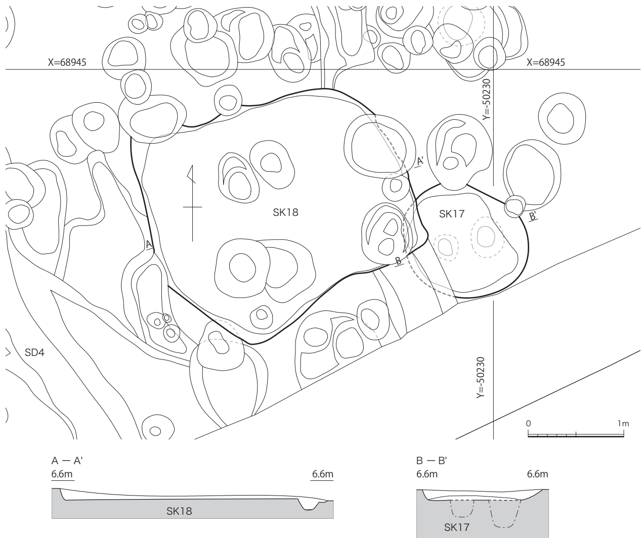
図20 SK17、SK18平面図、断面図(1/40)
