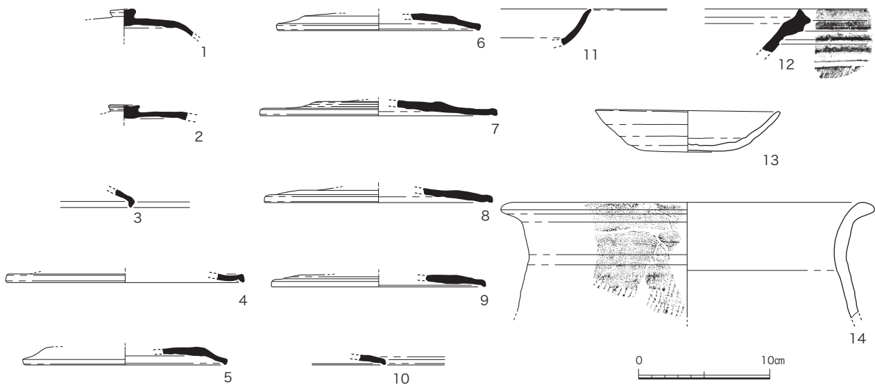
図8 SK2 出土遺物実測図(1/4)
