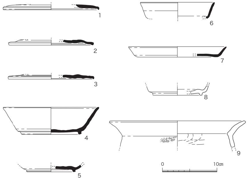
図14 SK7 出土遺物実測図(1/4)
