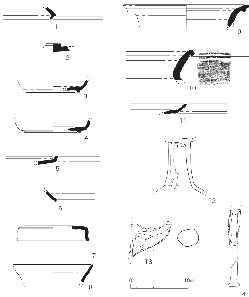
図 26 SD4 出土遺物実測図 (1/4)
