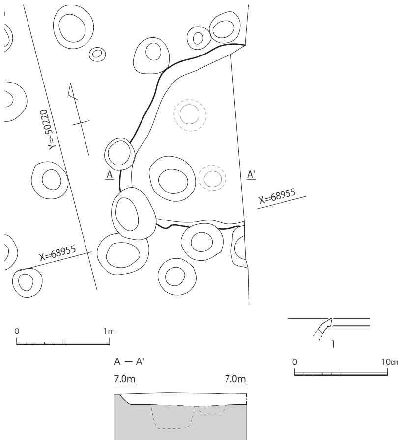
図6 SK1 平面図、断面図 (1/40)、出土遺物実測図 (1/4)
