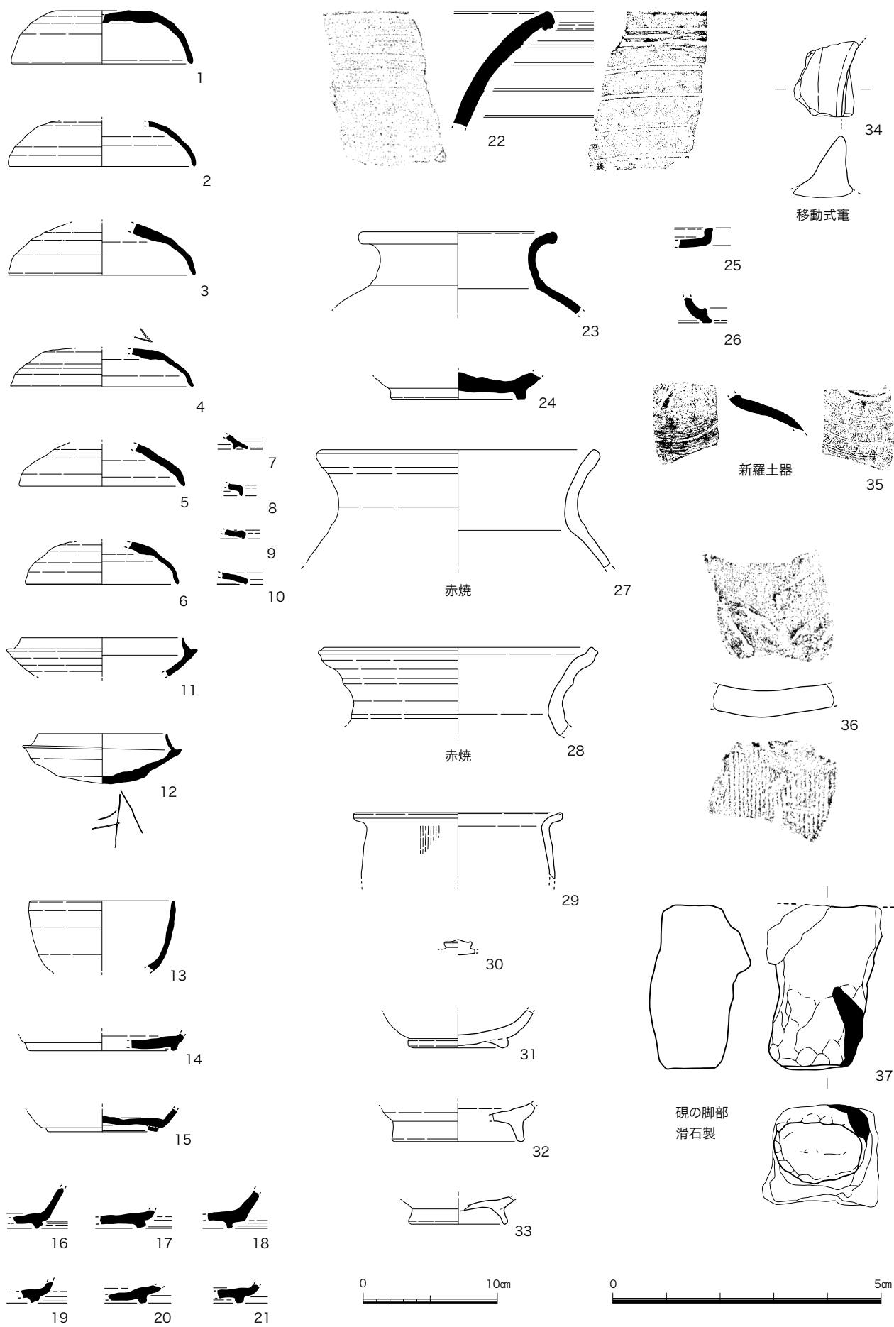
図 26 包含層出土遺物実測図 (1/4、石製品 1/1)
