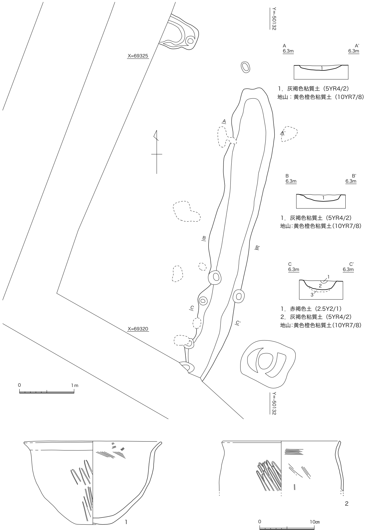
図3 A区 方形周溝墓平面図、断面図 (1/40)、出土遺物実測図 (1/4)
