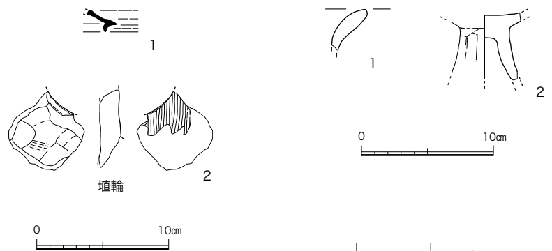
図22 SK-12 出土遺物実測図 (1/4)
