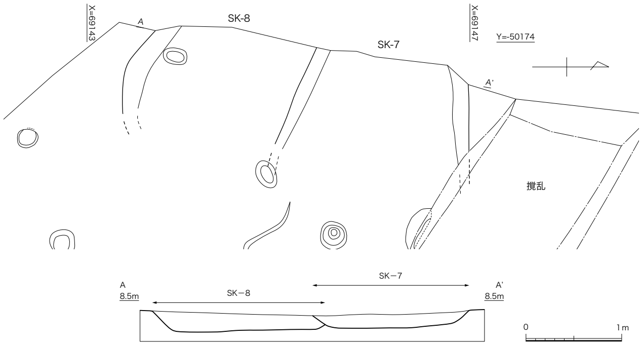
图 14 SK-7、8 平面図、断面図 (1/40)
