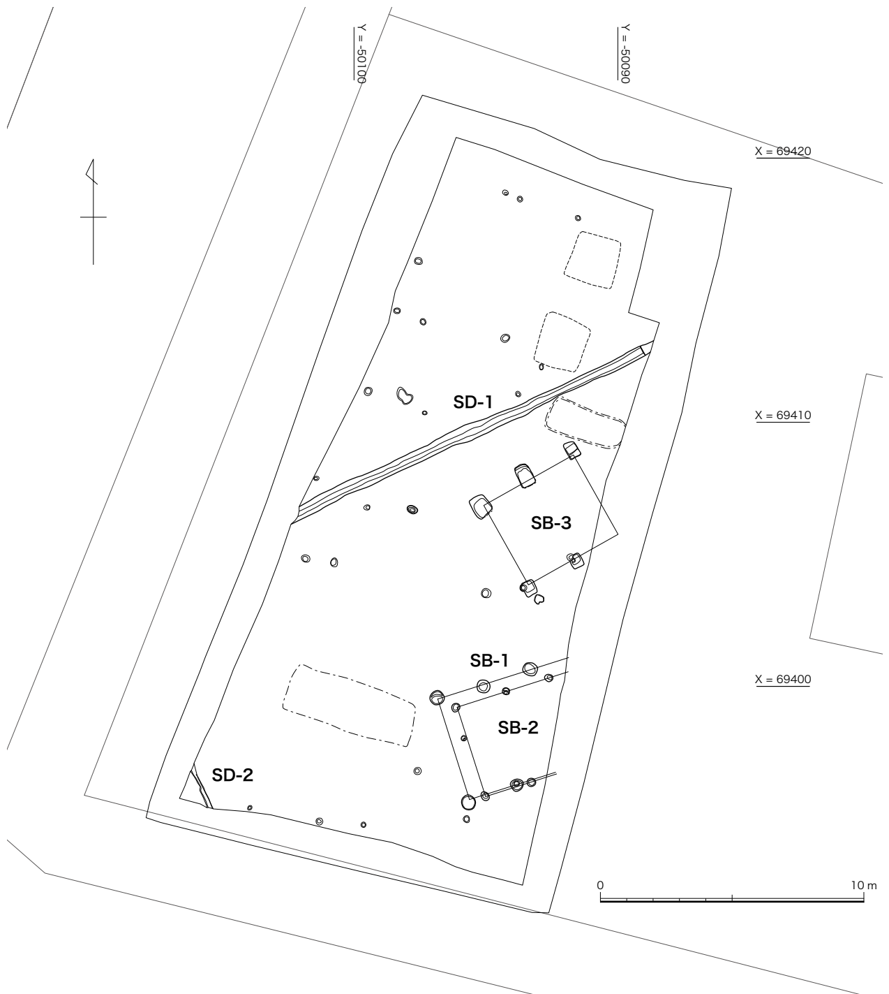
図2 内橋カラヤ遺跡第3地点平面図(1/200)
