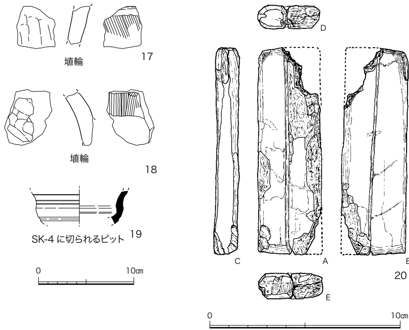
図12 SK-4 出土遺物実測図 (1/4、石器 1/2)
