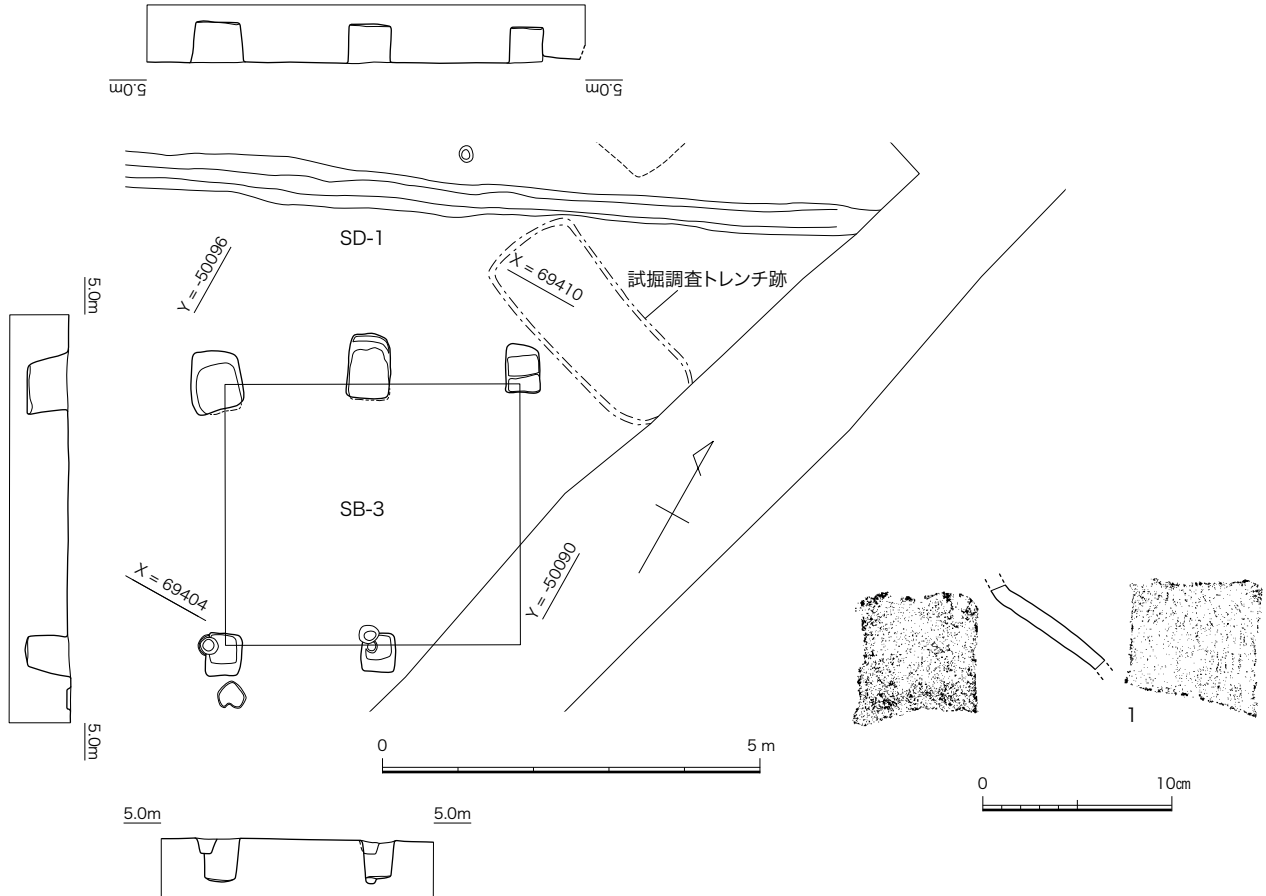
図6 SB-3 平面図、断面図 (1/100)、出土遺物実測図 (1/4)
