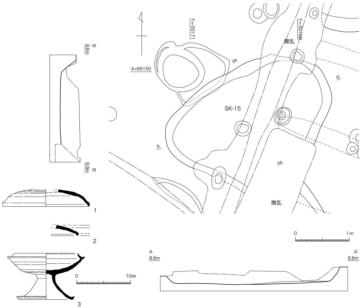
図24 SK-15平面図、断面図(1/40)、出土遺物実測図(1/4)
