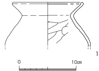
図5 SB-2 出土遺物実測図 (1/4)
