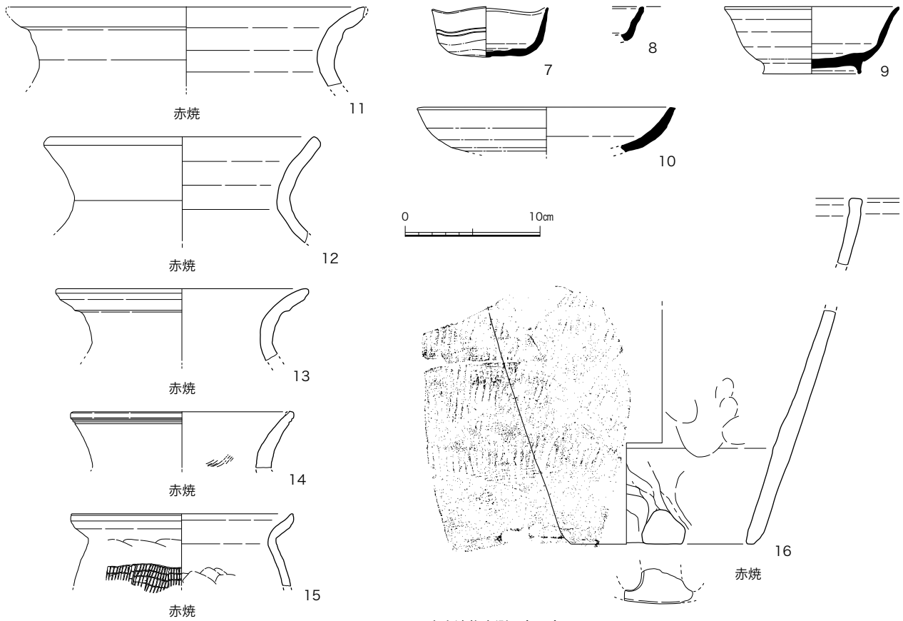
图11 SK-4 出土遺物実測图(1/4)
