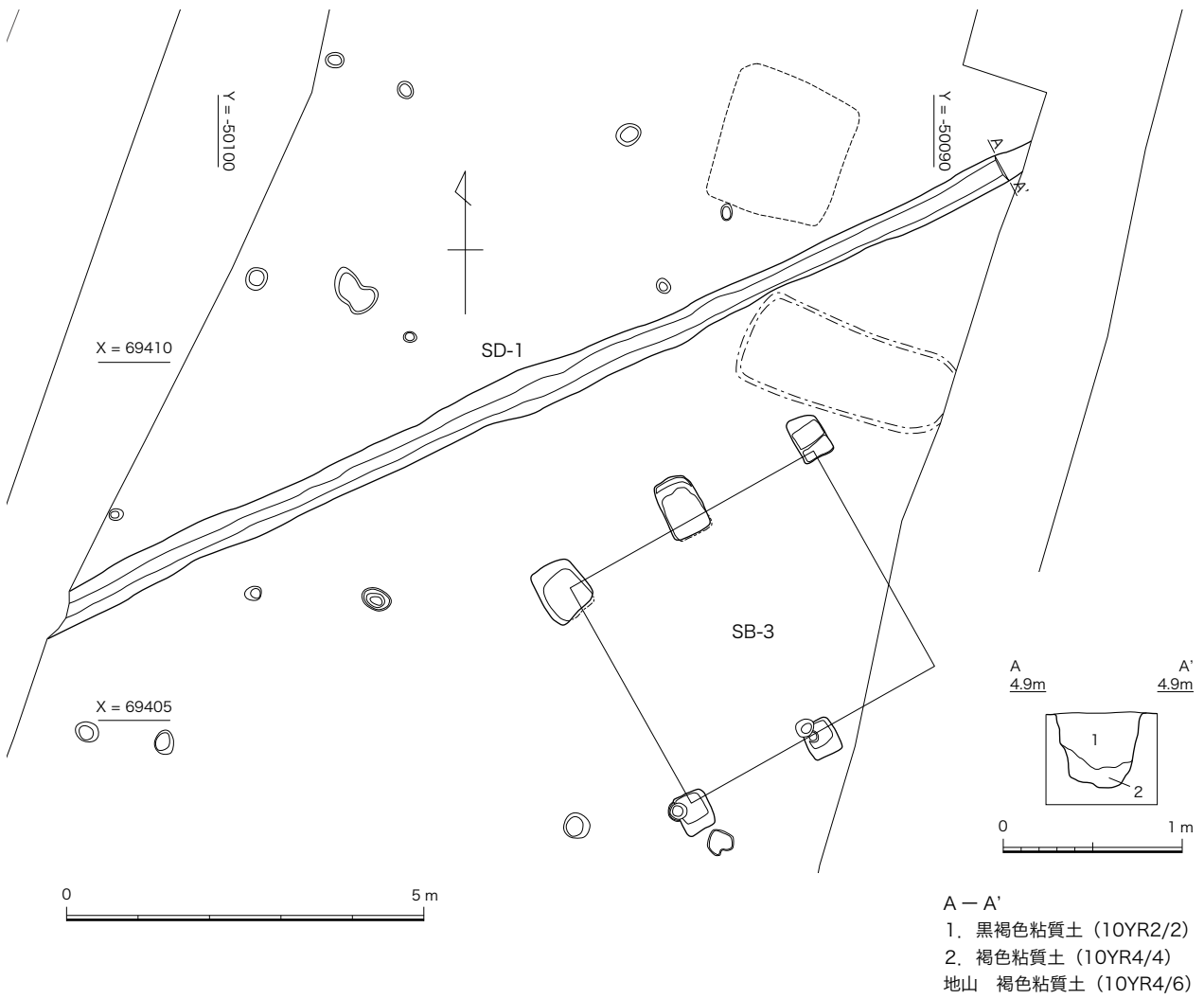
図8 SD-1 平面図 (1/100)、土層断面図 (1/20)
