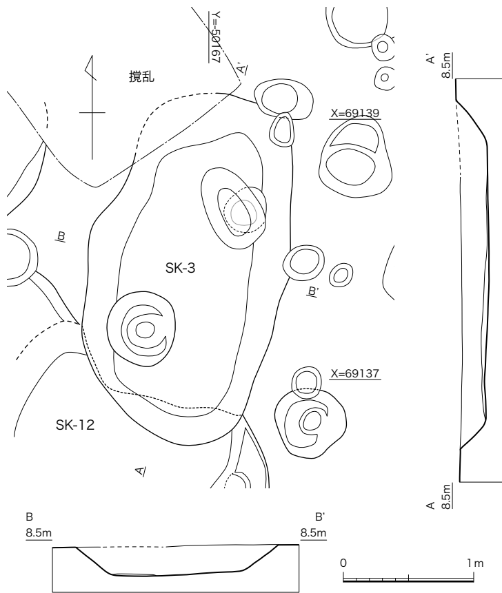
図8 SK-3平面図(1/40)
