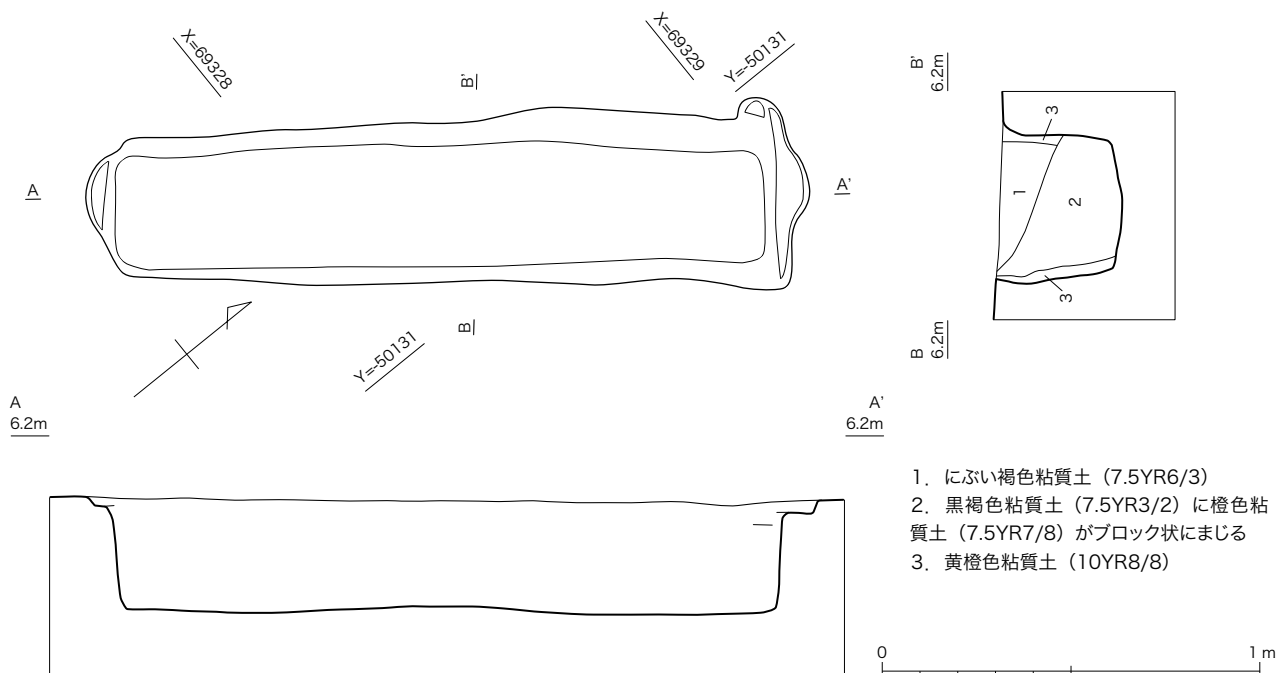
図4 A 区 木棺墓平面図、断面図 (1/20)
