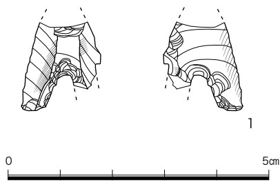
図5 A区 木棺墓出土遺物実測図(1/1)
