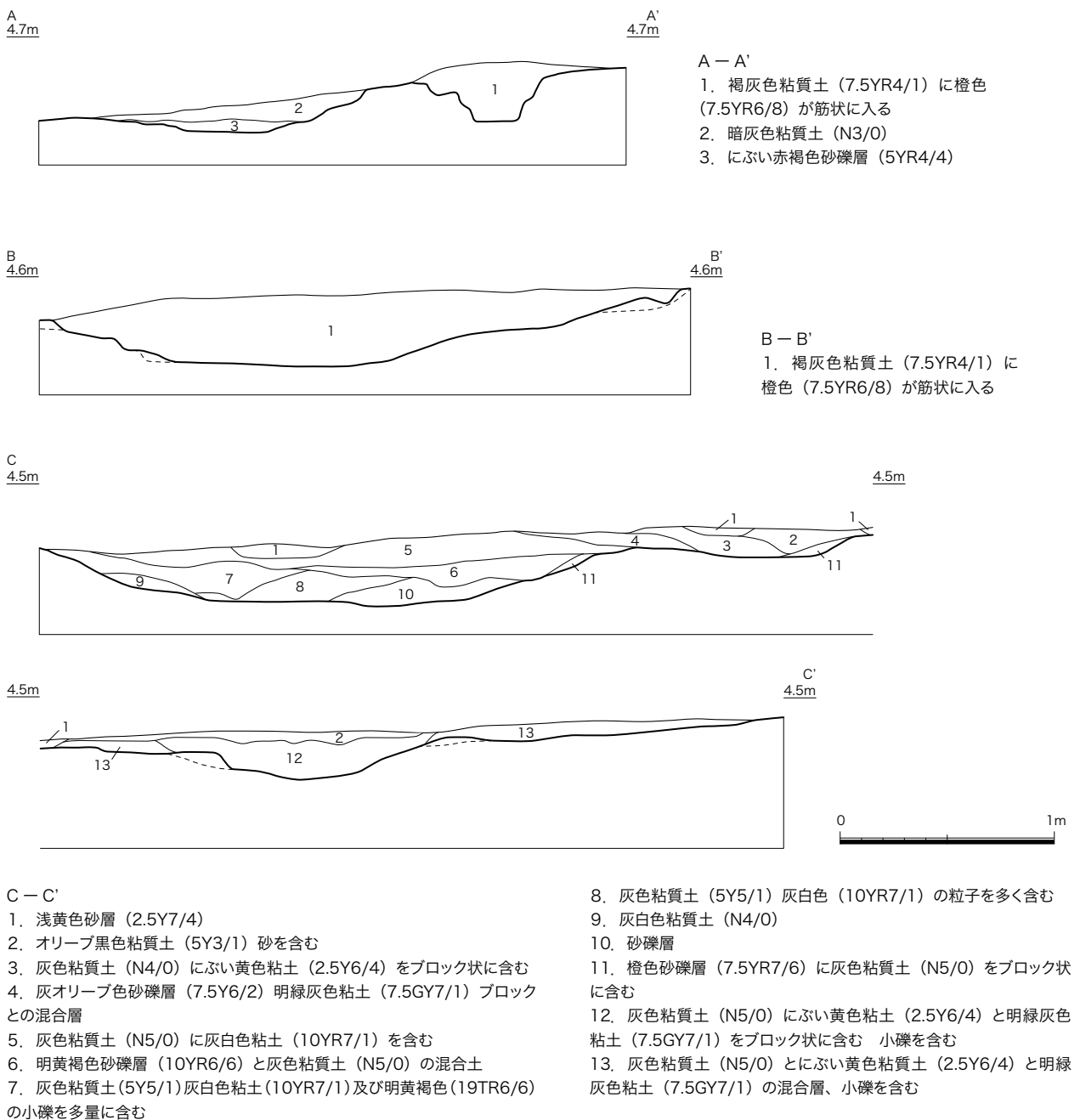
図9 B区 第1号～第5号溝状遺構土層図(1/30)
