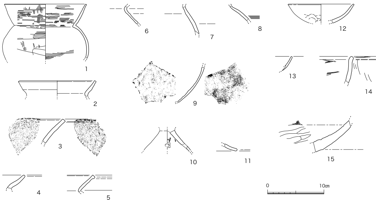
図9 SD-1 出土遺物実測図 (1/4)
