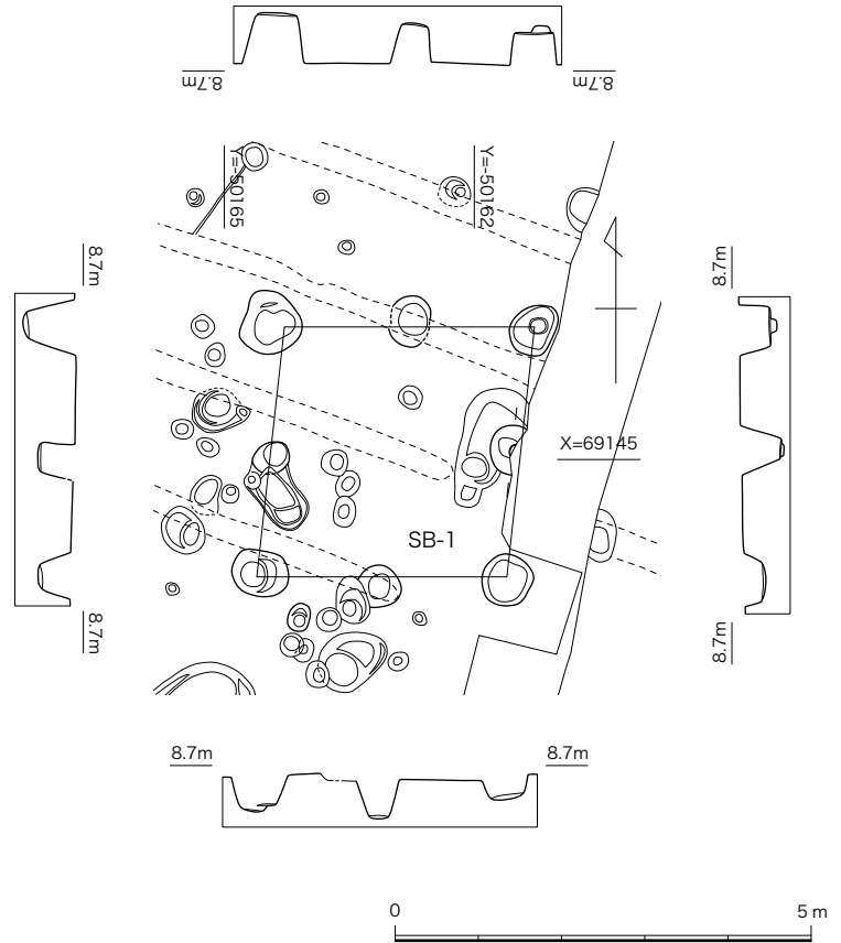
図4 SB-1 平面図、断面図 (1/100)
