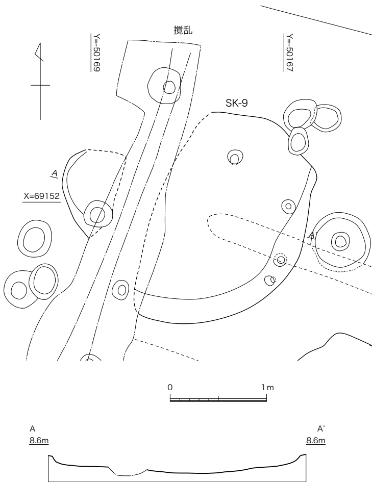
图 16 SK-9 平面図、断面図 (1/40)
