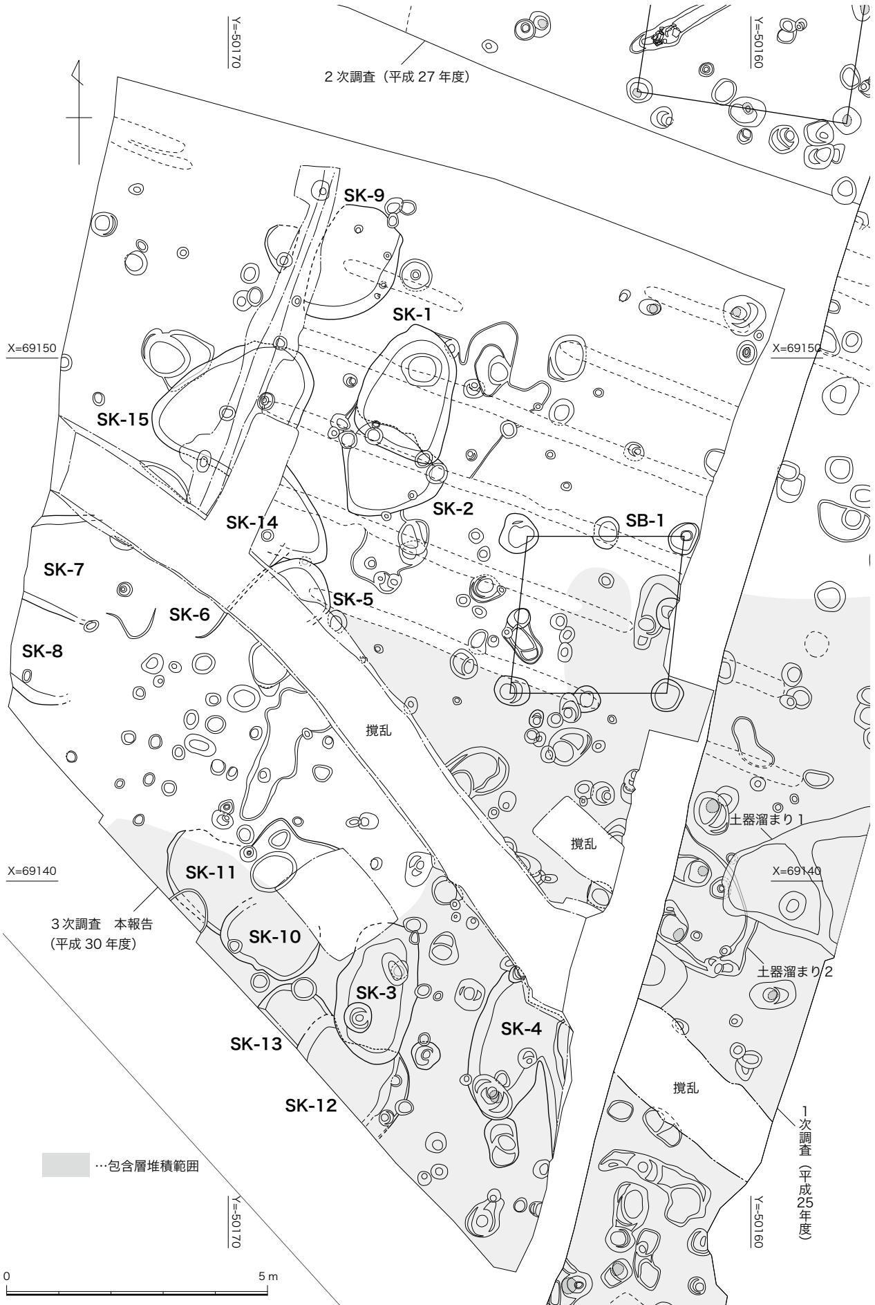
図3 内橋鏡遺跡3次平面図(1/100)
