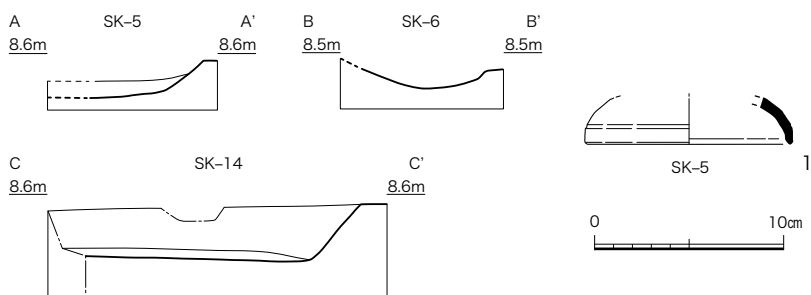
図13 SK-5、6、14 平面図、断面図 (1/40)、SK-5 出土遺物実測図 (1/4)
