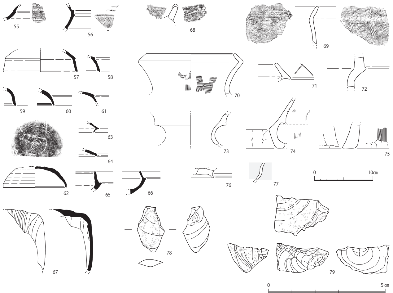
第12図 ピット出土遺物実測図 (1/4、1/1)
