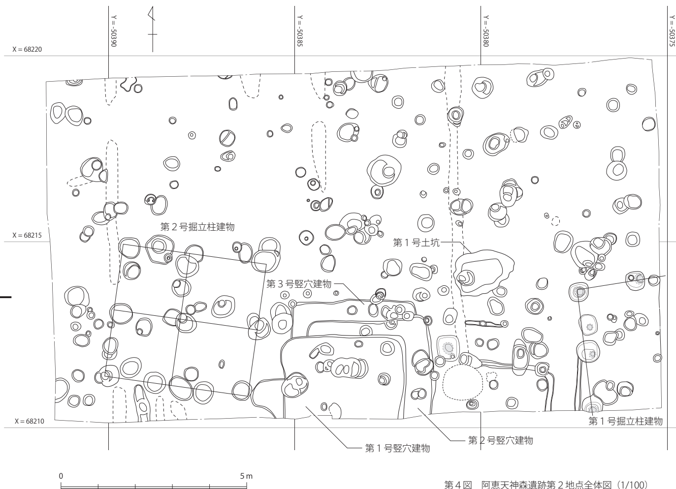
第4図 阿恵天神森遺跡第2地点全体図 (1/100)
