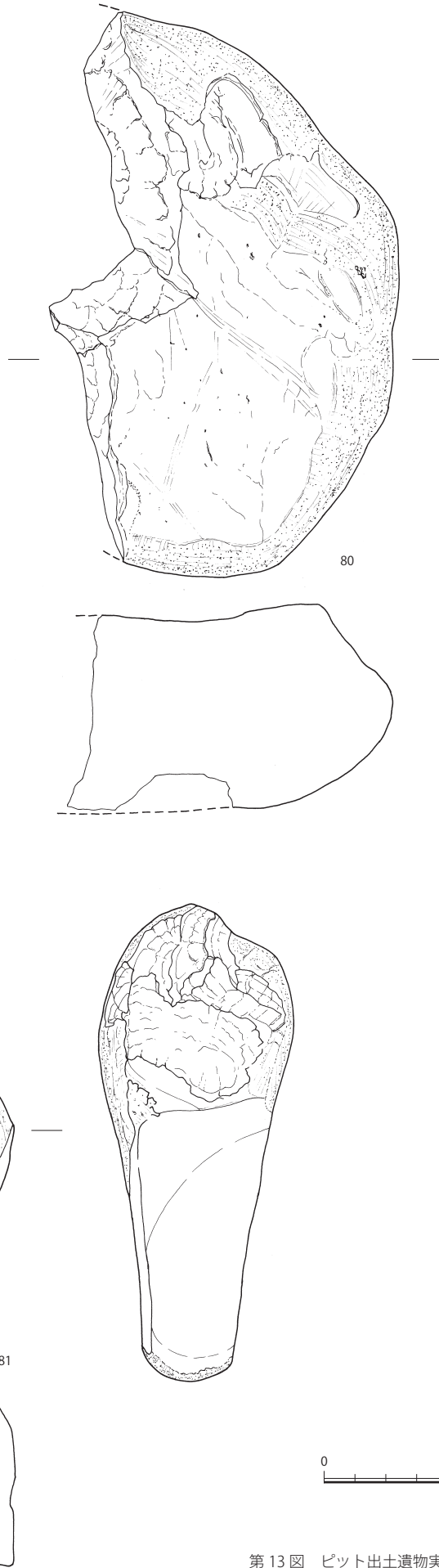
第13図 ピット出土遺物実測図 (1/2)
