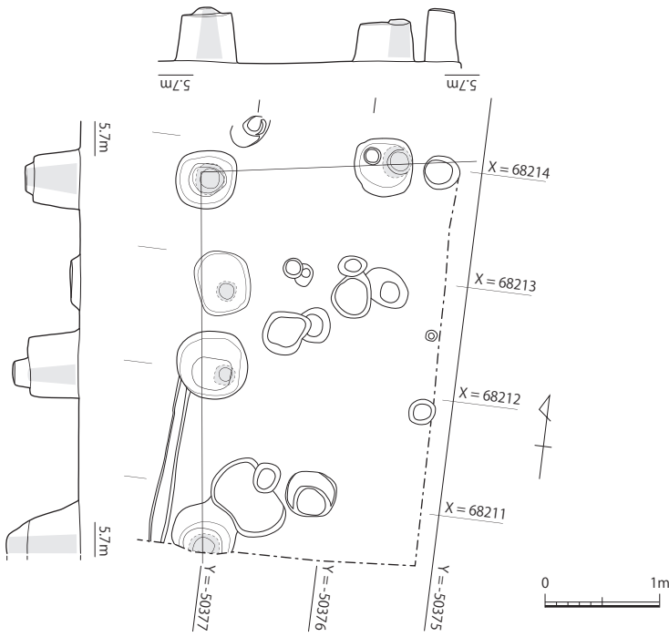
第7図 第1号掘立柱建物実測図(1/60)
