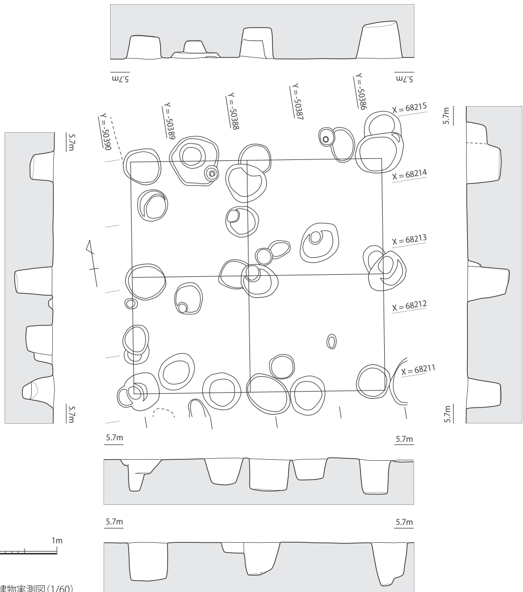
第8図 第2号掘立柱建物実測図(1/60)
