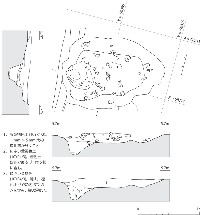
第10図 第1号土坑実測図(1/30)
