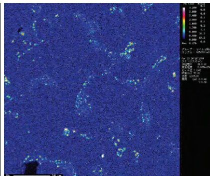
C-7 鉛 (Pb) X線像
