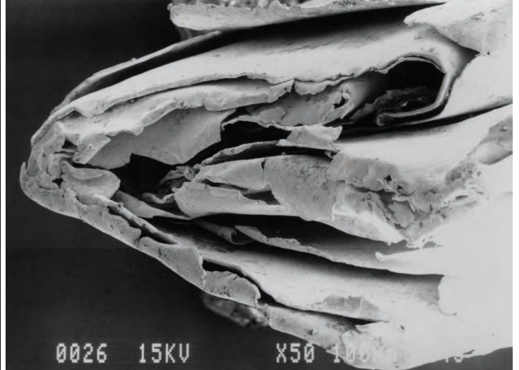
C-2-2 折り重なり部（電子顕微鏡観察）
