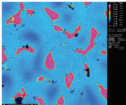
C-7 アンチモン (Sb) X線像
