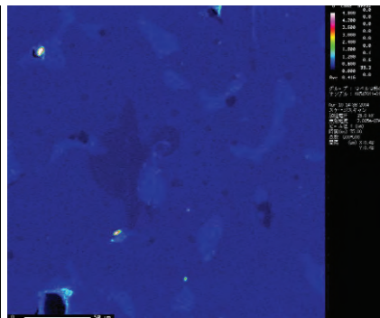
C-7 酸素 (O) X線像
