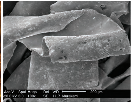
C-1-3 金糸部分の拡大（電子顕微鏡観察）
