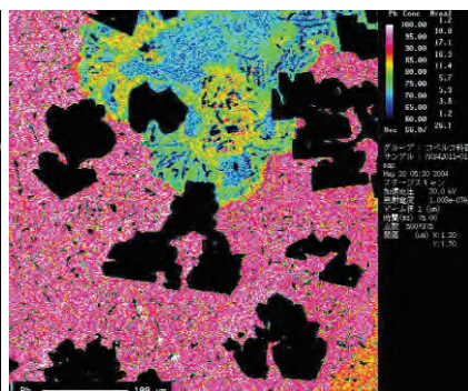
C-8 鉛 (Pb) X線像
