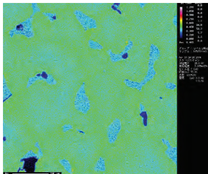
C-7 ヒ素 (As) X線像
