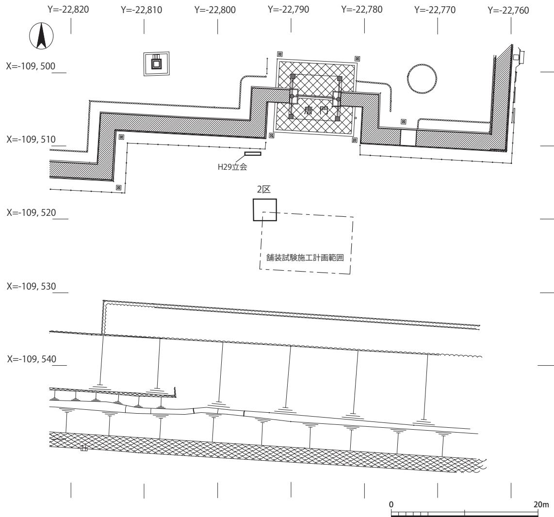
図9 2区配置図（1：500）
