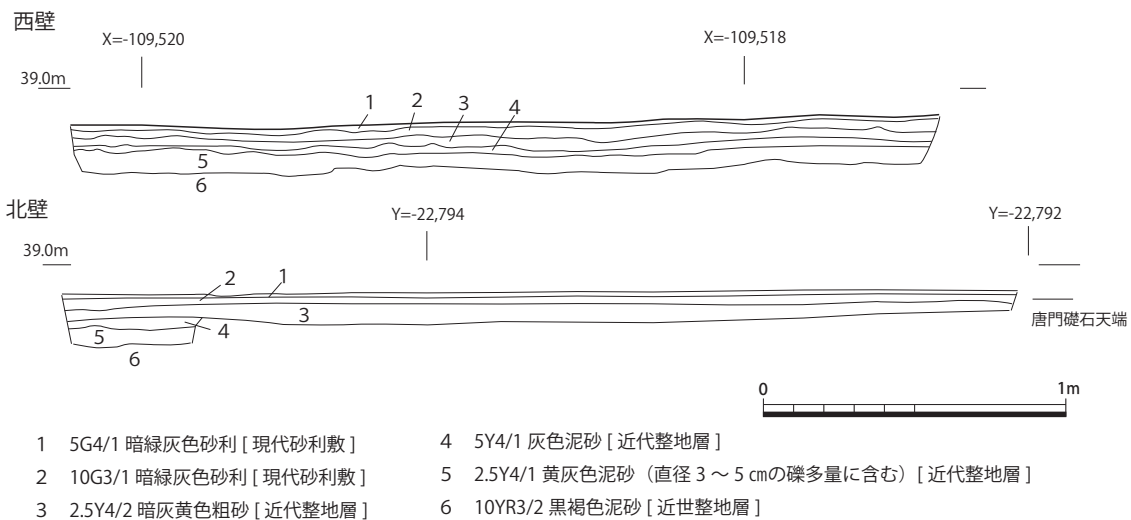
図11 2区段面図 (1:25)
