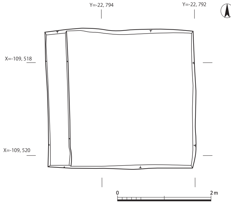
図10 2区平面図 (1:50)
