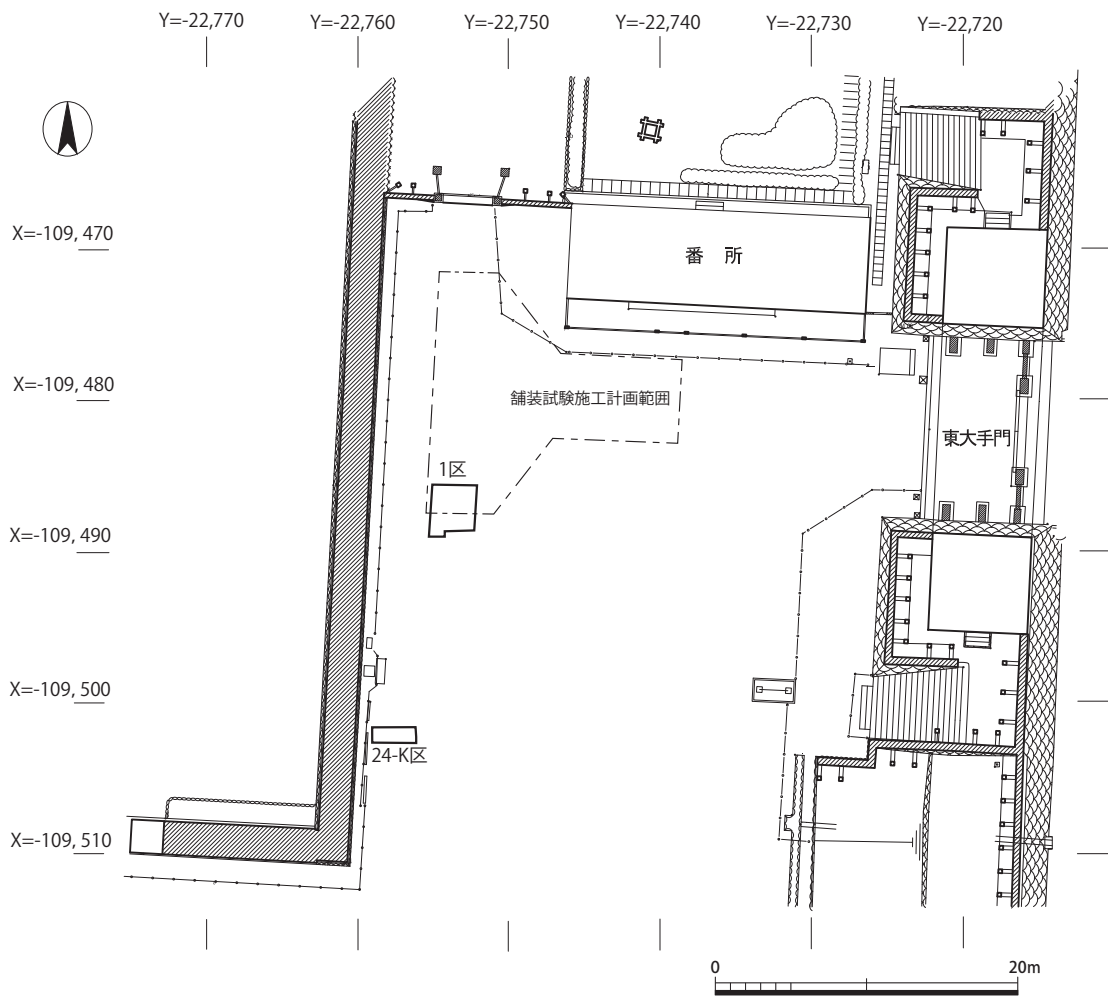
図6 1区配置図 (1 : 500)
