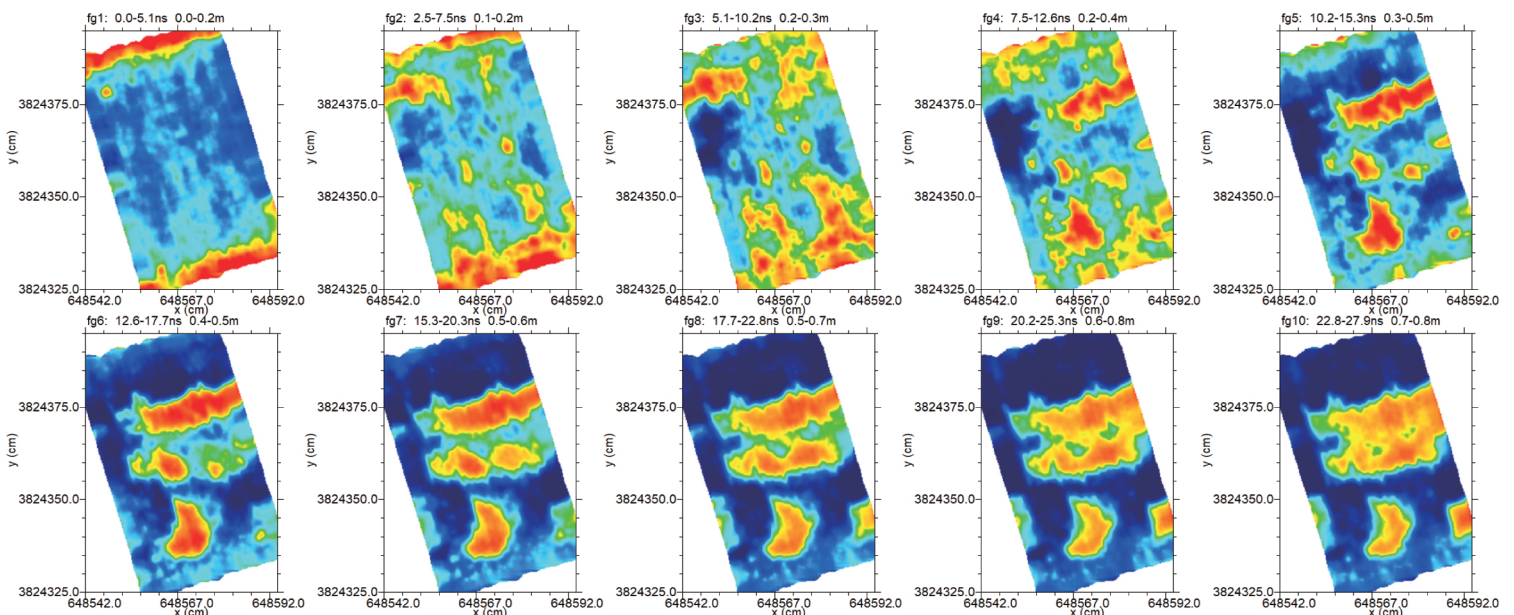
第12図 地中レーダー探査の結果
