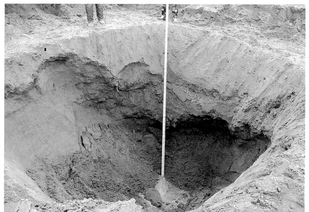
写真39 58T西壁土層堆積状況
