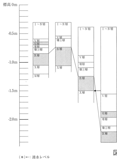
土層柱状図 ②
