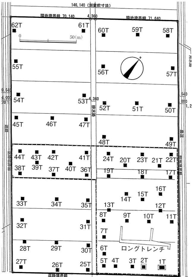
図3 調査坑配置図 (S=1/2,000)
