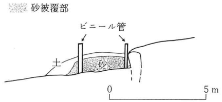
北西の久保3号古墳埋土保存模式図
