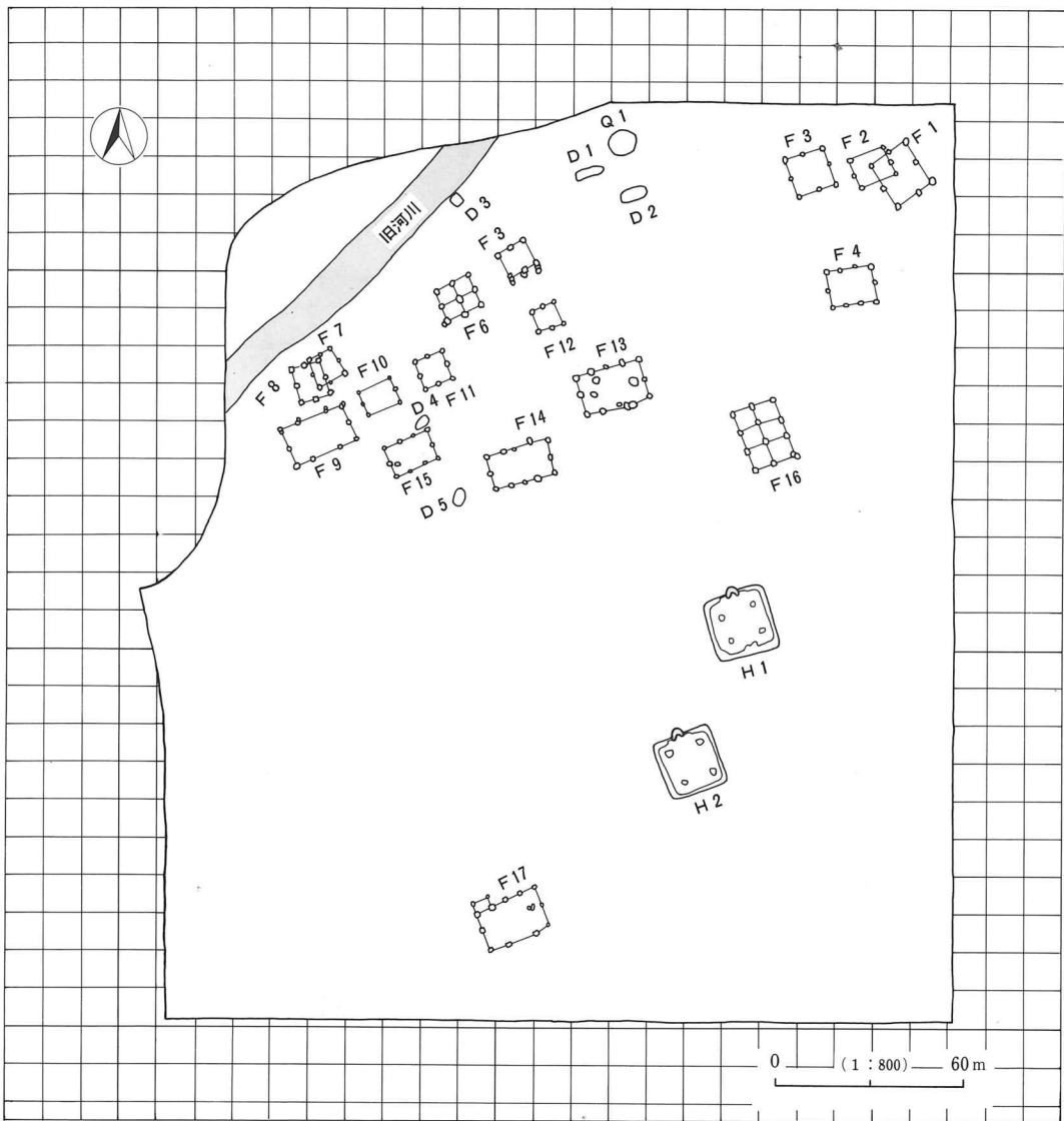
西曾根遺跡遺構全体図
