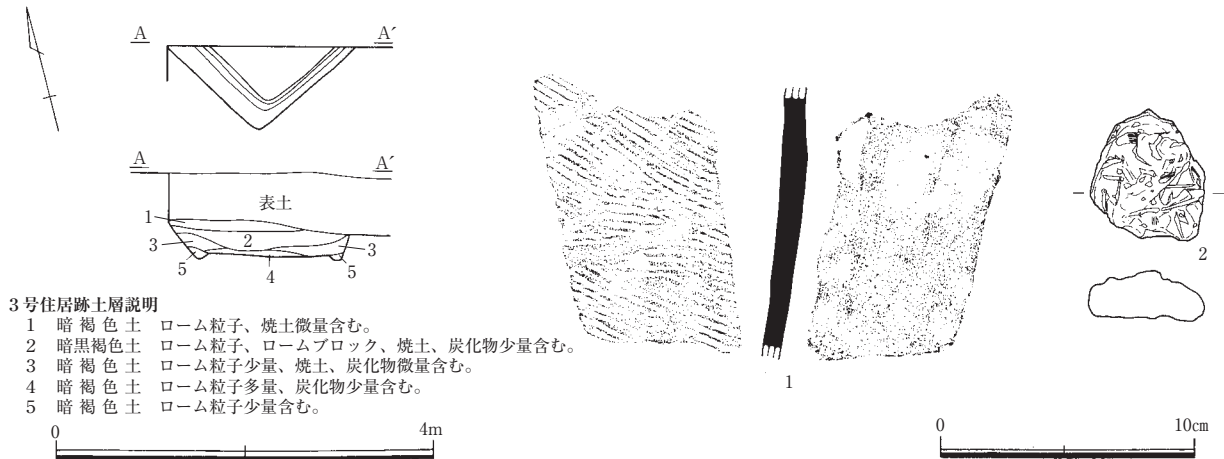
第14図 東海道遺跡3号住居跡及び出土遺物
