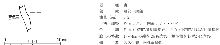
図5 出土遺物実測図 (S=1/4)
