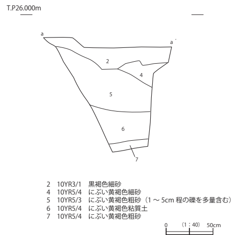
図 18 ④ブロック北側断割土層断面図 (1 : 40)
