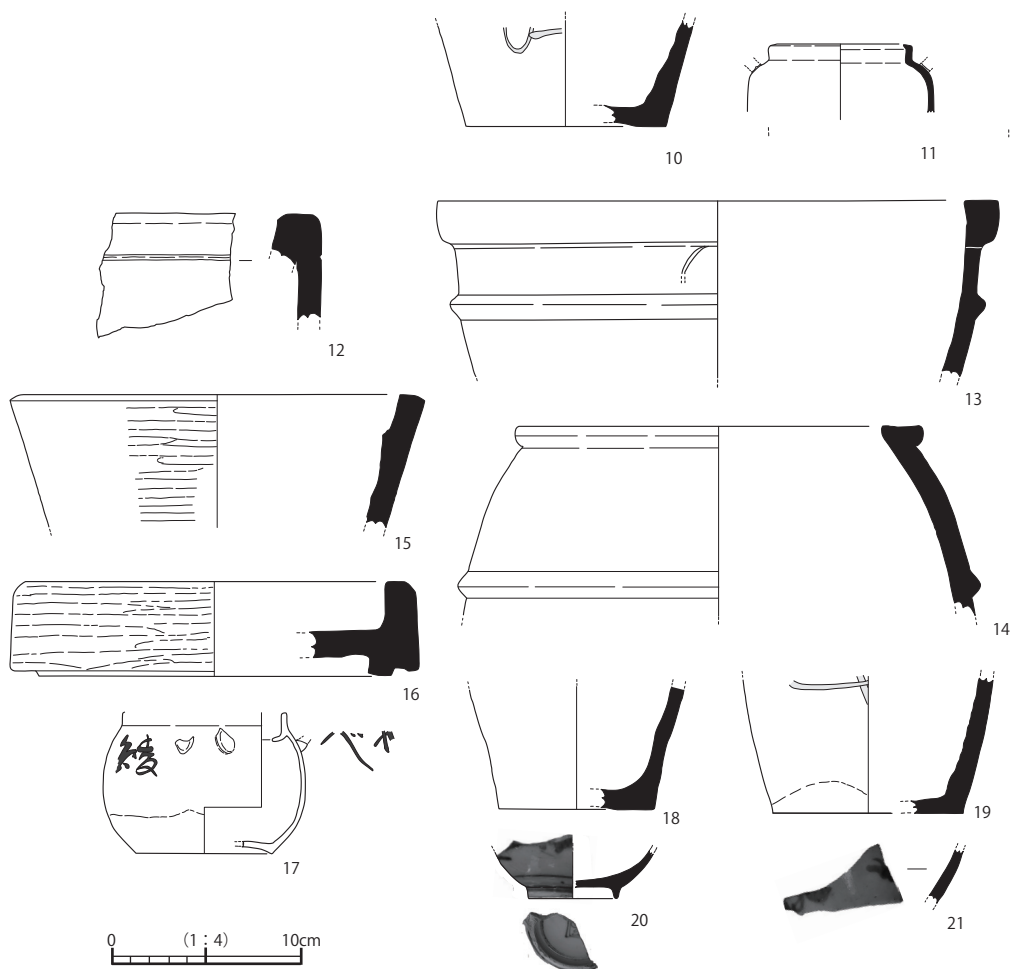
図22 ④ブロック出土器 (1:4)
