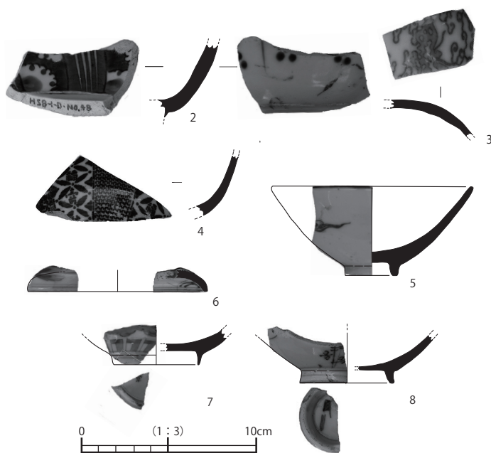
図20 ②ブロック出土土器 (1:3)
