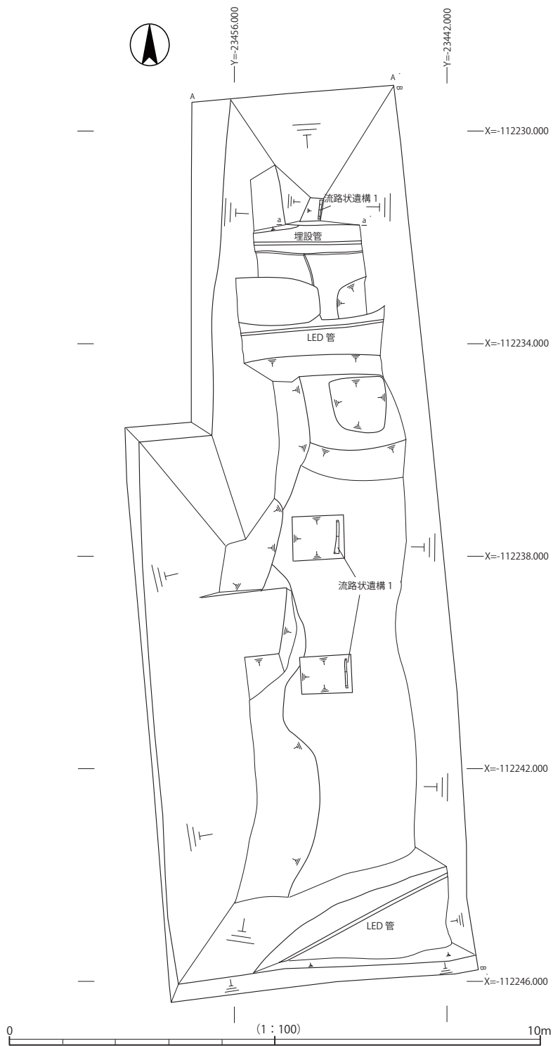
図 17 ④ブロック平面図 (1 : 100)
