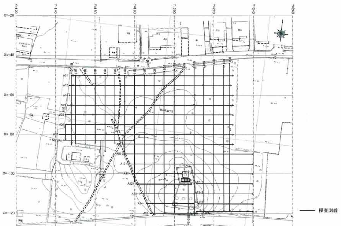
測線配置図
