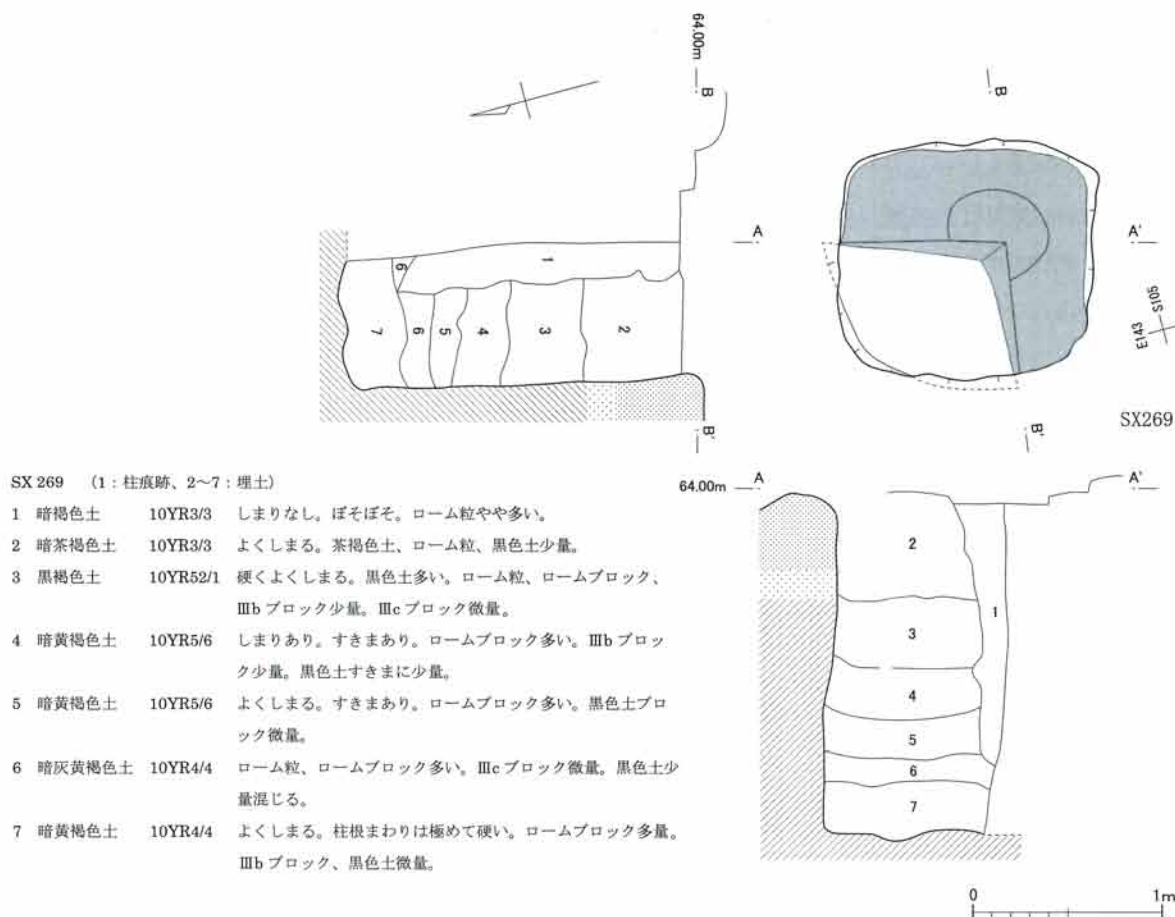
第9図 SX269一本柱跡平面・断面図
