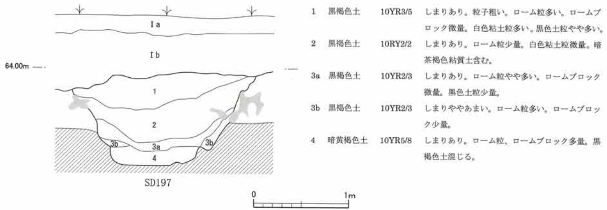
第14図 第578次調査No. 1地点 昭和33年度中央旧トレンチ SD197溝跡南北断面図
