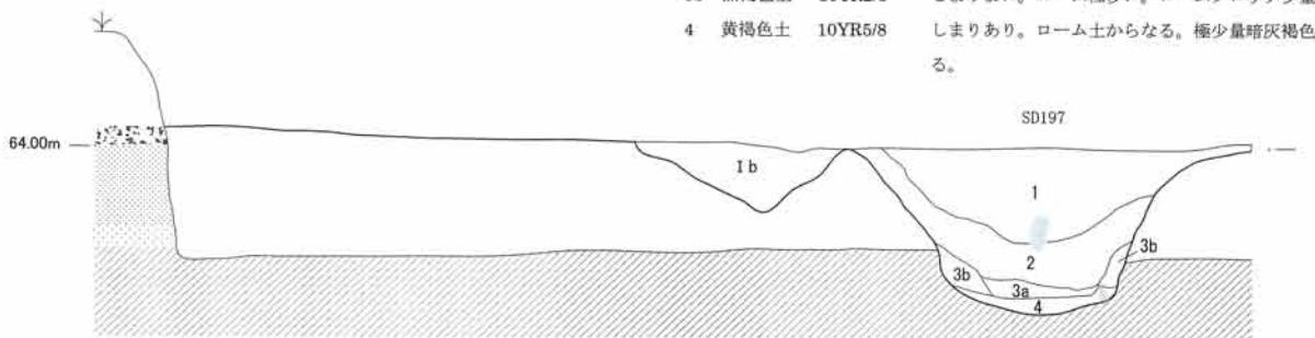
第11図 第570次調査No.6地点 昭和33年度旧トレンチ 南北断面図
