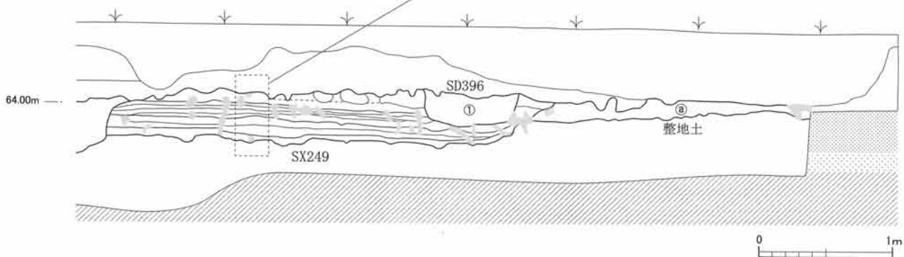
第15図 第578次調査No. 1地点 昭和33年度中央旧トレンチ SX249築地塀跡南北断面図
