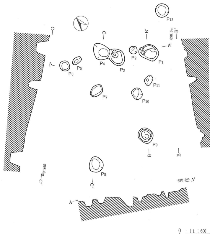
第31図 F2号掘立柱建物址実測図
