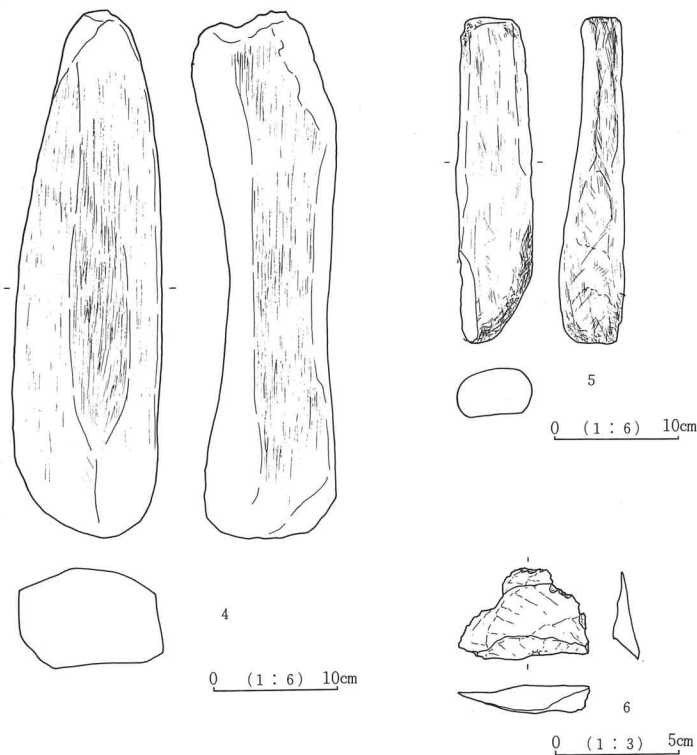
第16図 H2号住居址出土遺物実測図
