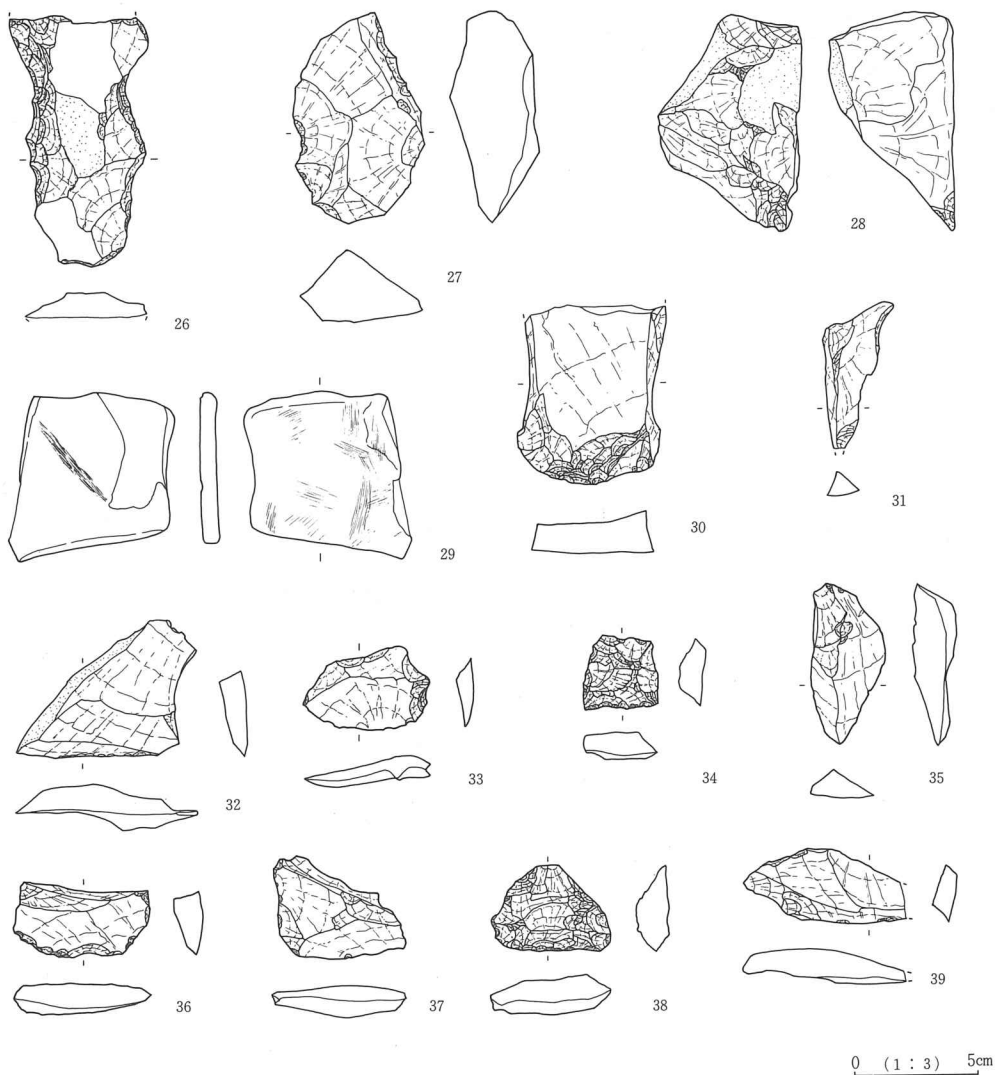
第46图 A区集中分布地区出土縄文時代遺物実測図
