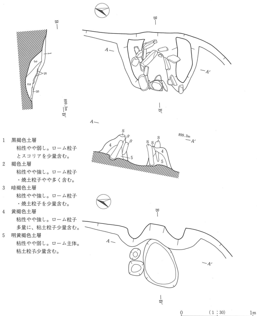
第14図 H2号住居址カマド実測図
