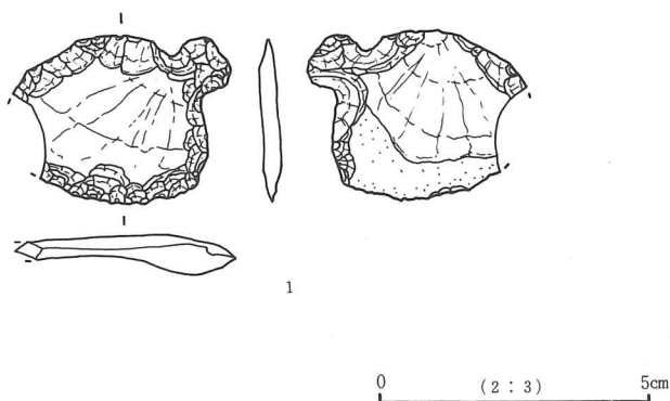
第40図 第3号土坑出土石器実測図
