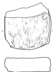
第53図 グリッドおよび表採遺物実測図
