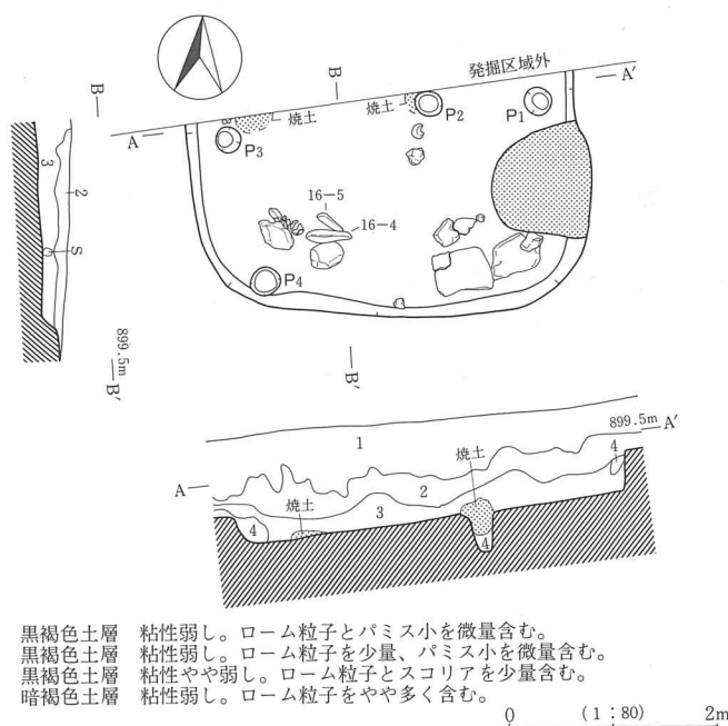
第13図 H2号住居址実測図
