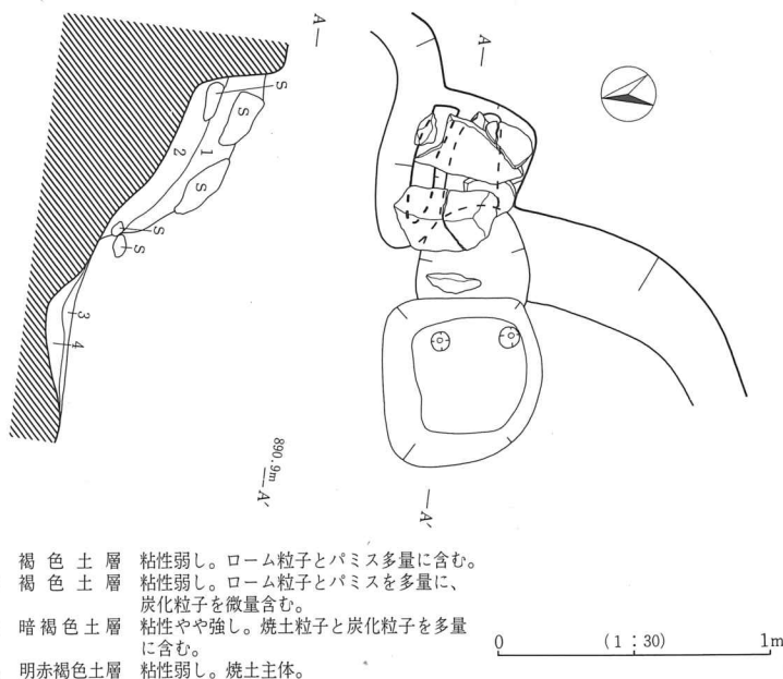
第7図 H1号住居址2号カマド実測図
