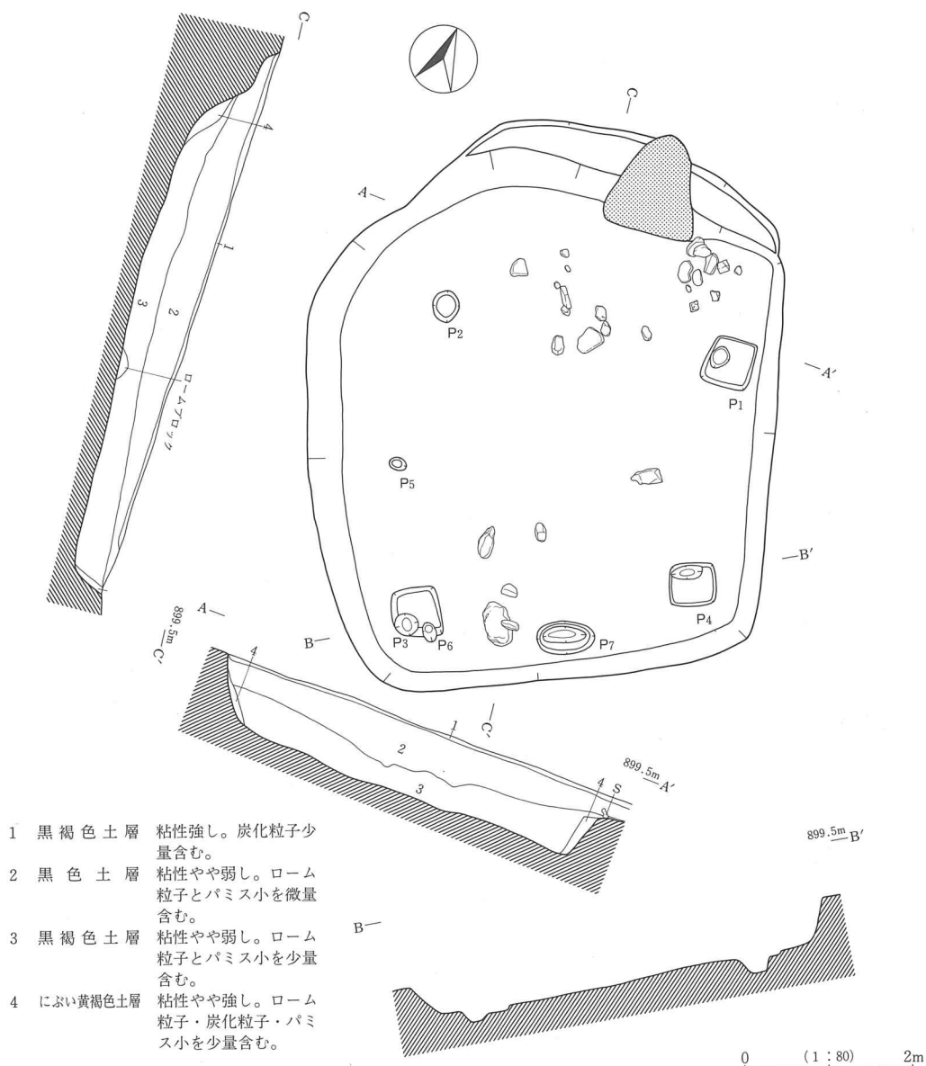
第18図 H3号住居址実測図
