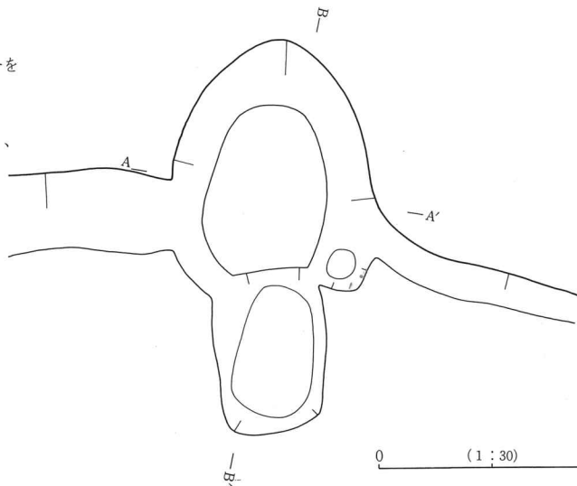
第19図 H3号住居址カマド実測図
