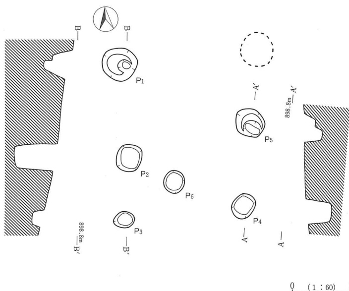
第29図 F1号掘立柱建物址実測図
