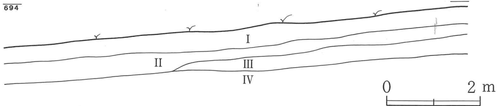
第5図 第2トレンチ実測図 (1/80)
