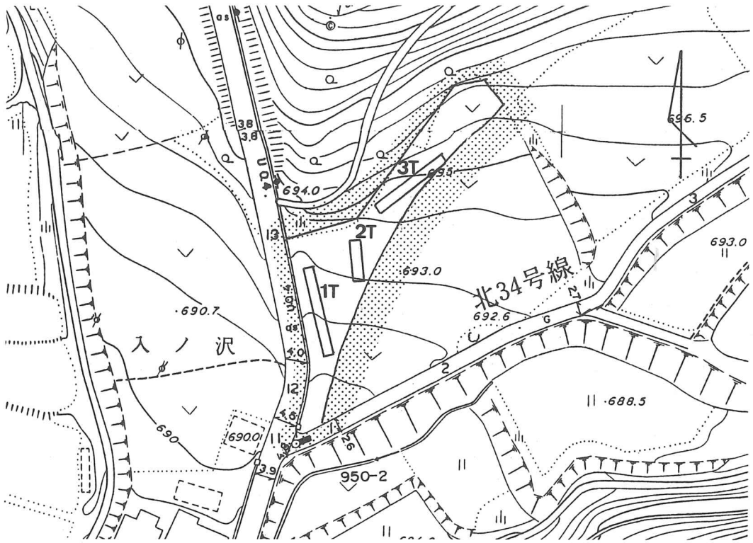
第2図 トレンチ配置図 (1/1,000)
