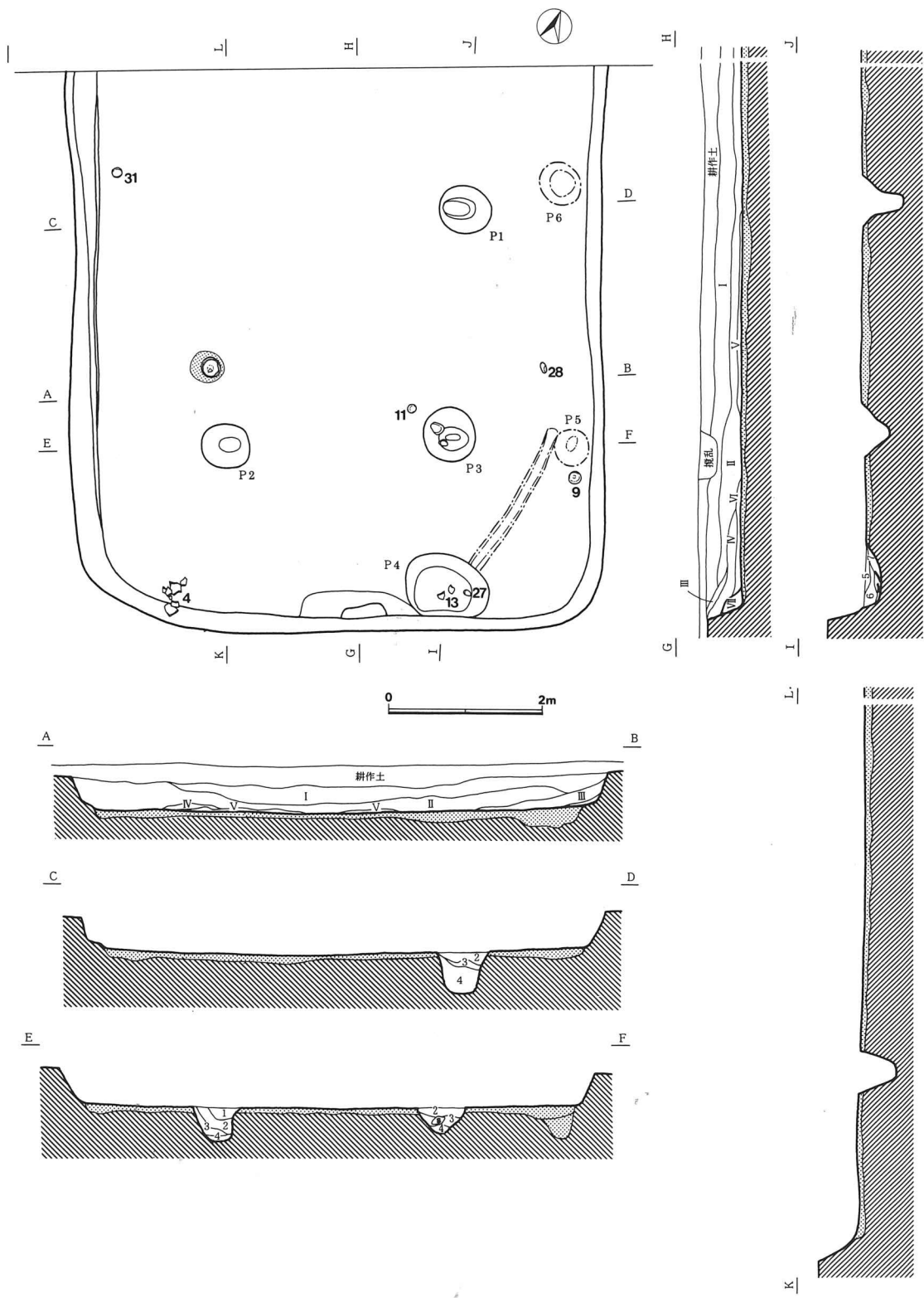
第9图 Y-1号住居址 (1:80)
