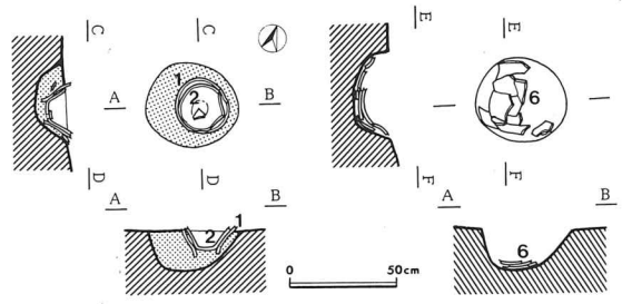
第10図 Y-1号住居址炉 (1:40)
