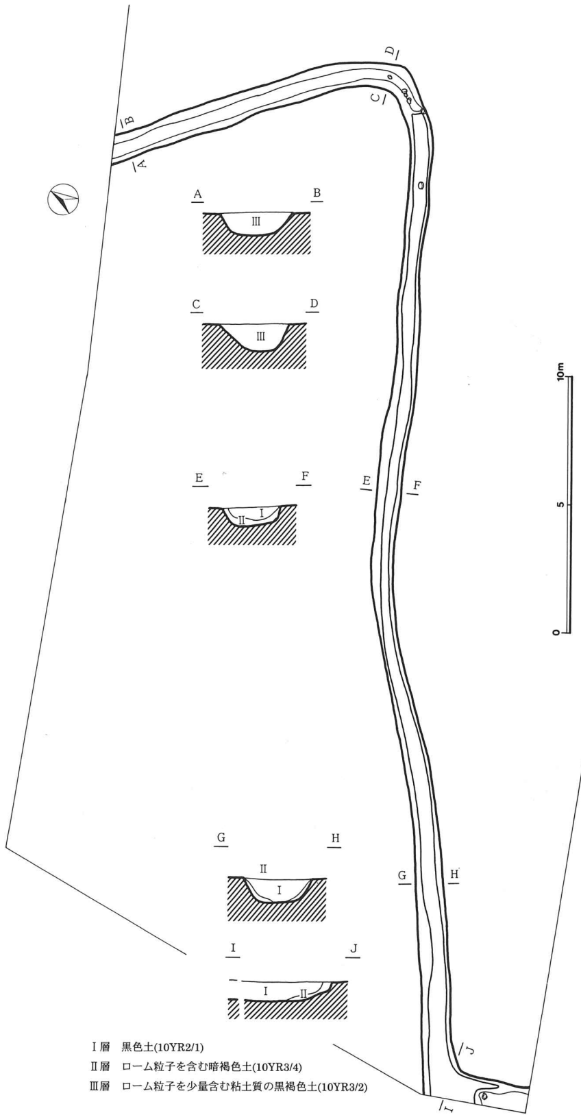
第22図 M-2号溝状遺構 (1:200)
