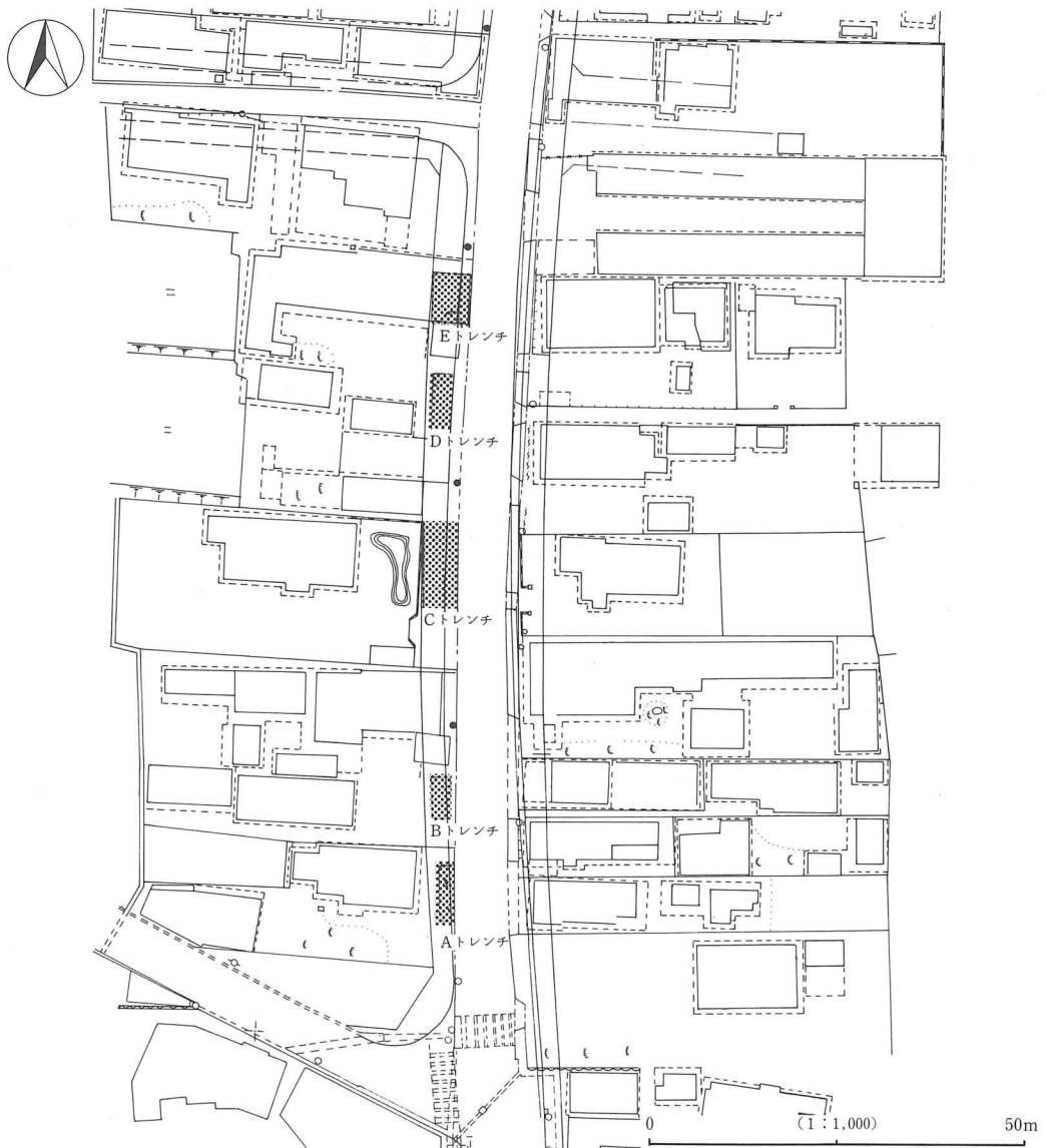
第1図 新町遺跡地形及び調査区設定図
