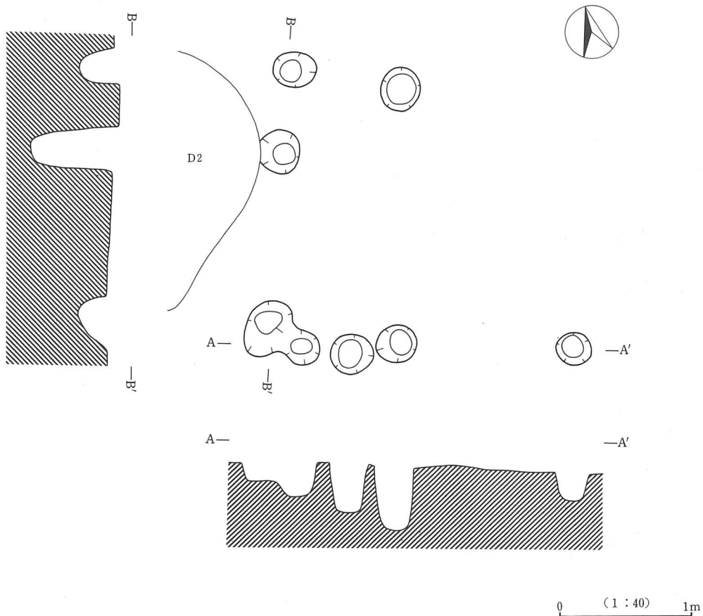
第7図 F2号掘立柱建物址実測図
