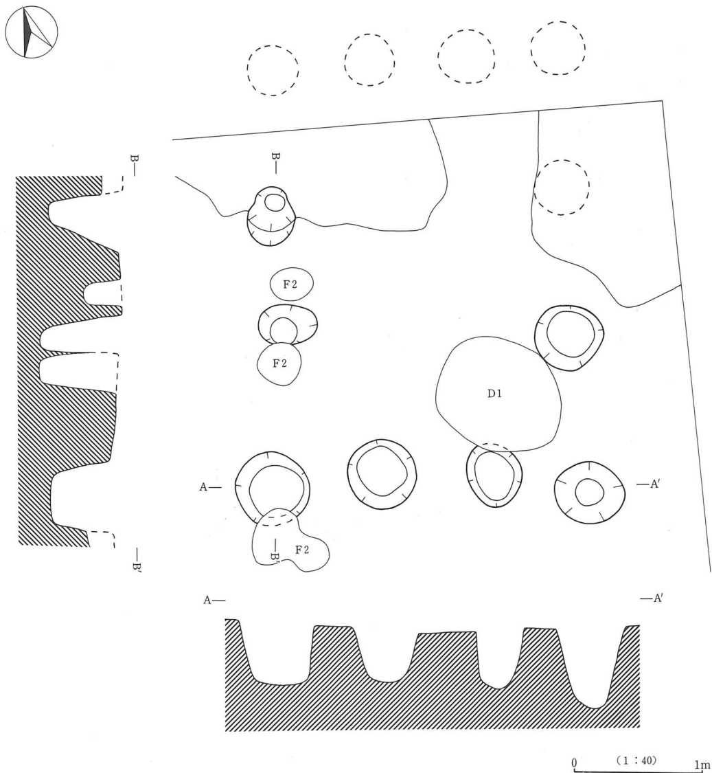
第6図 F1号掘立柱建物址実測図
