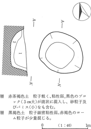
第4図 D1号土坑実測図
