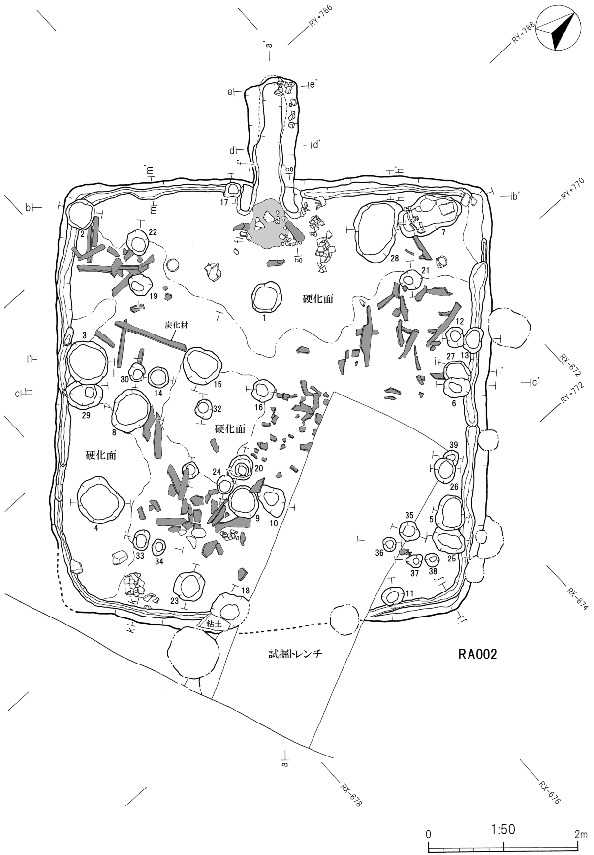
第26図 RA002竪穴建物跡(1)
