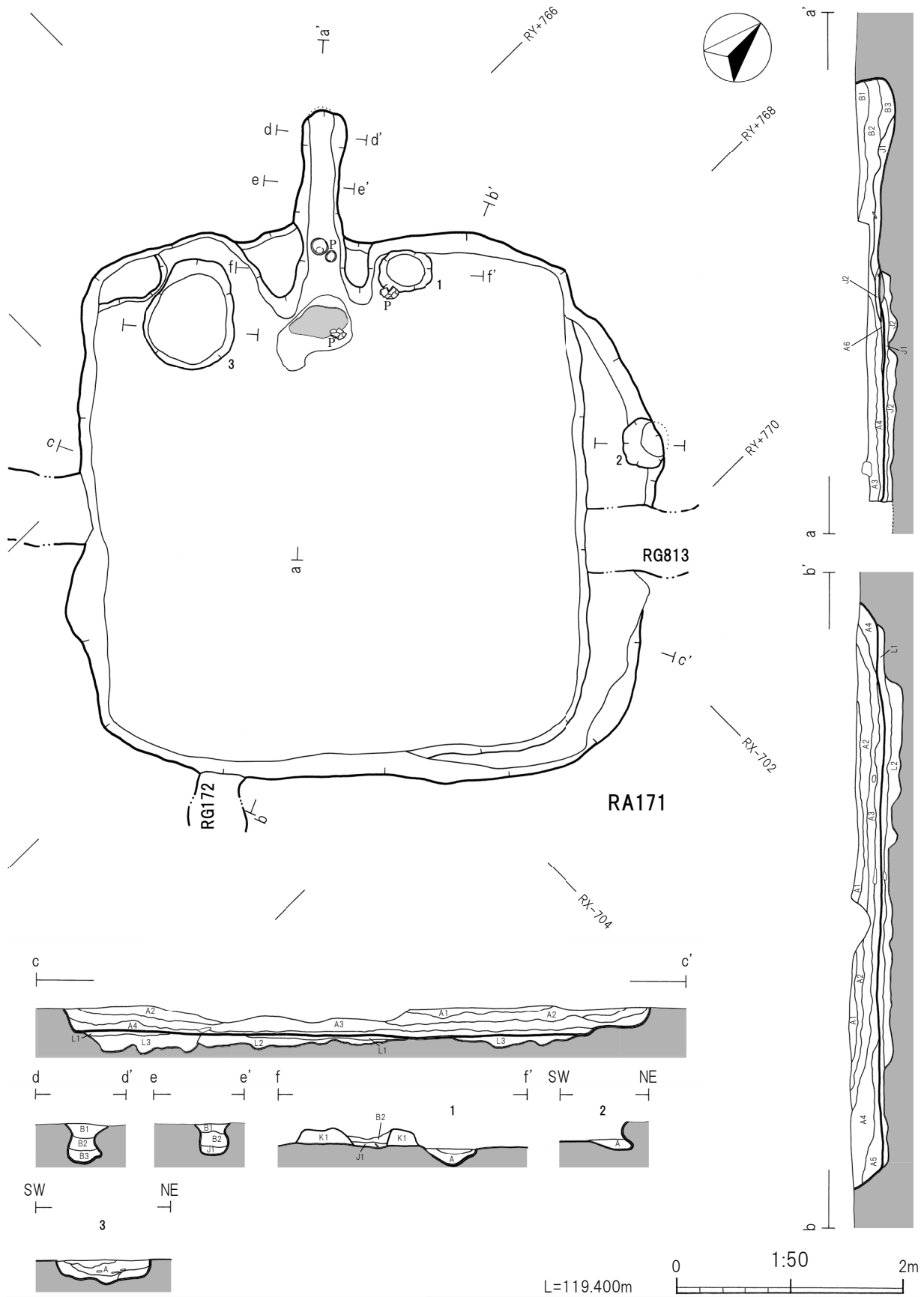
第57図 RA171豎穴建物跡
