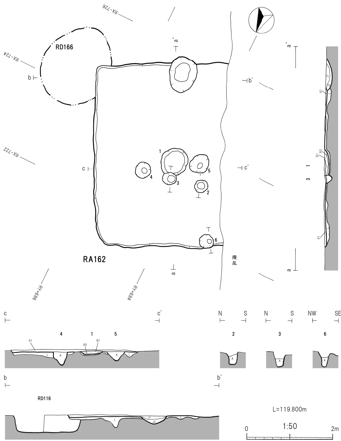
第52図 RA162竪穴建物跡
