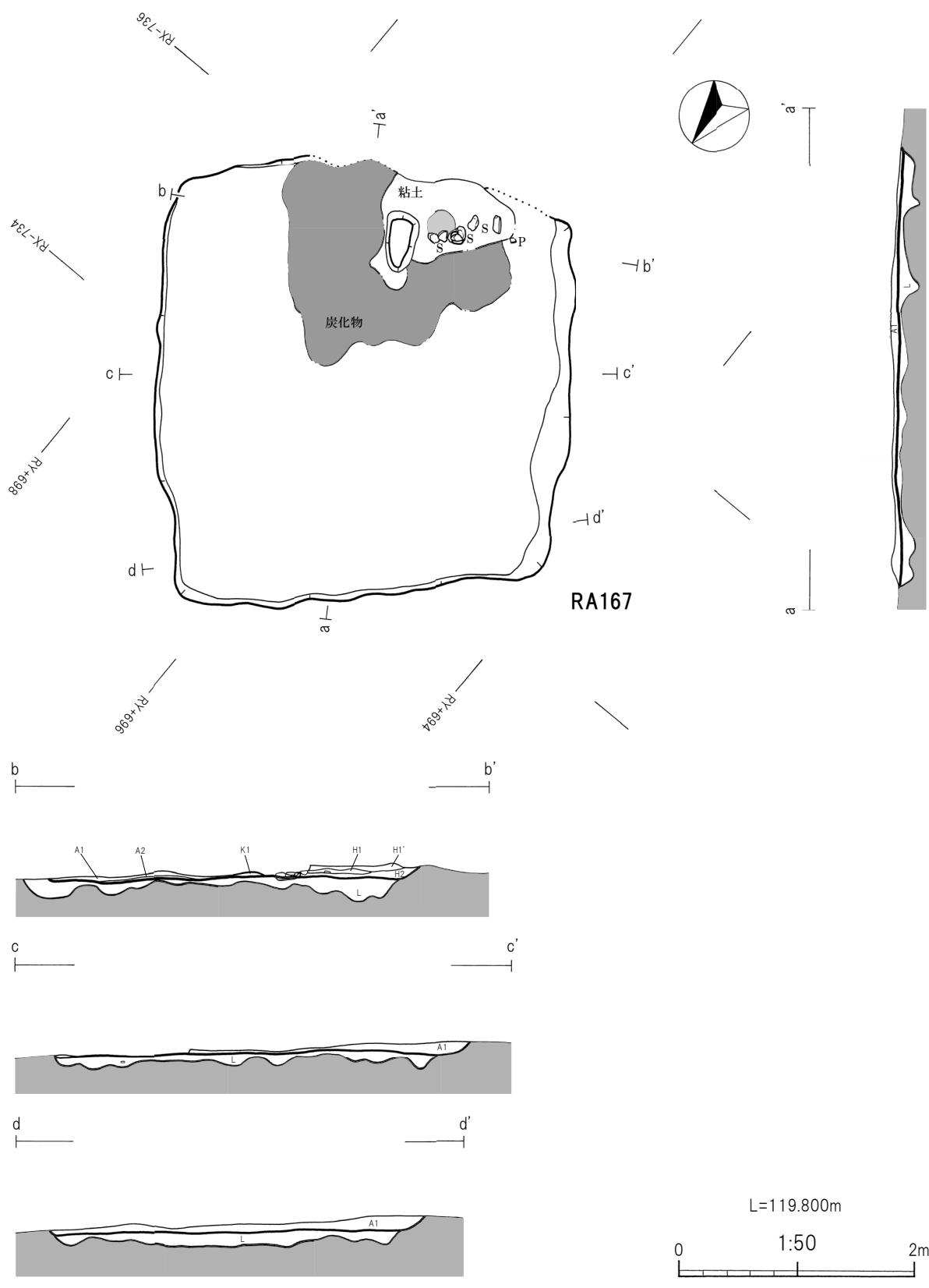
第55図 RA167竪穴建物跡
