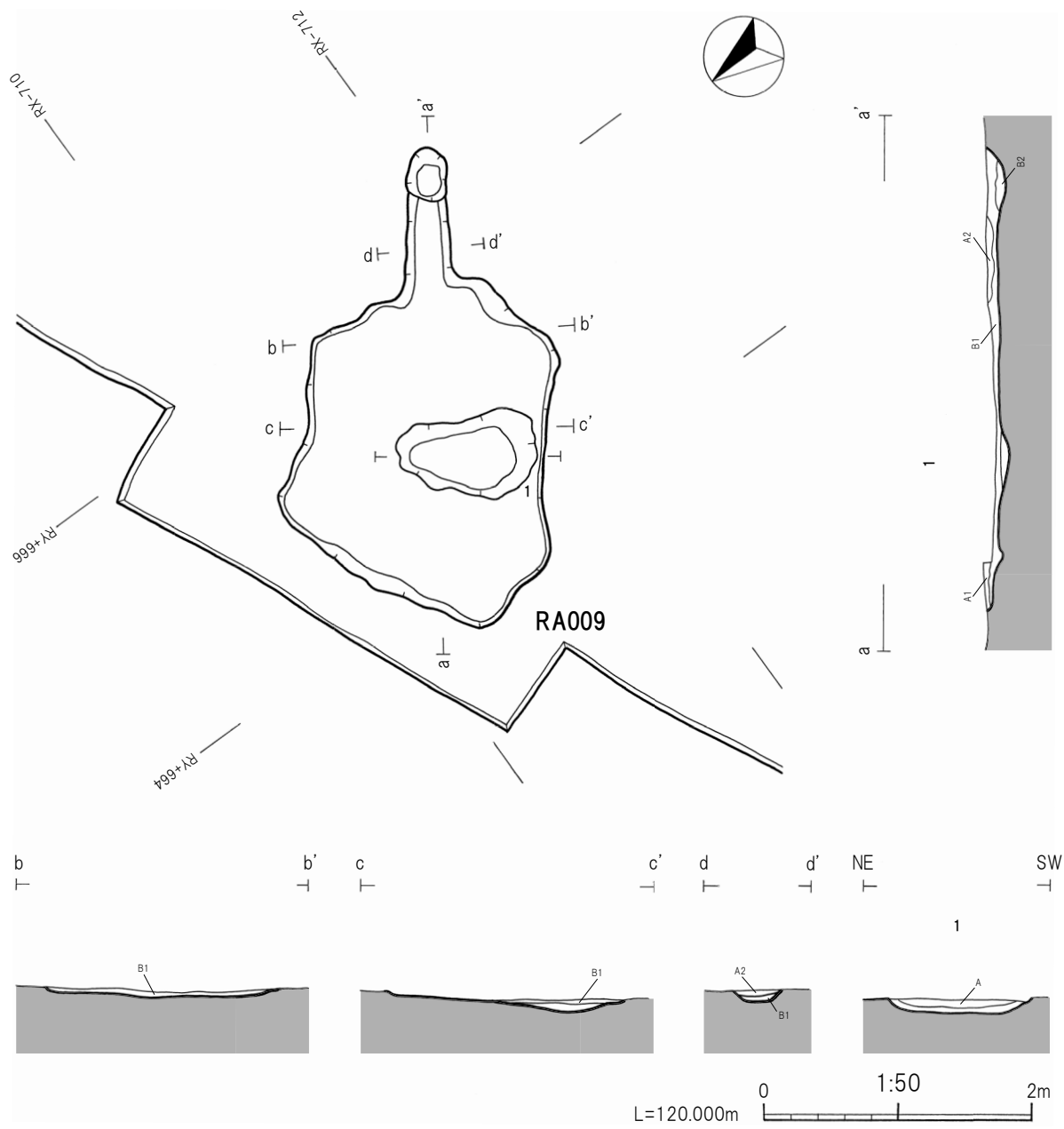
第34図 RA009竪穴建物跡
