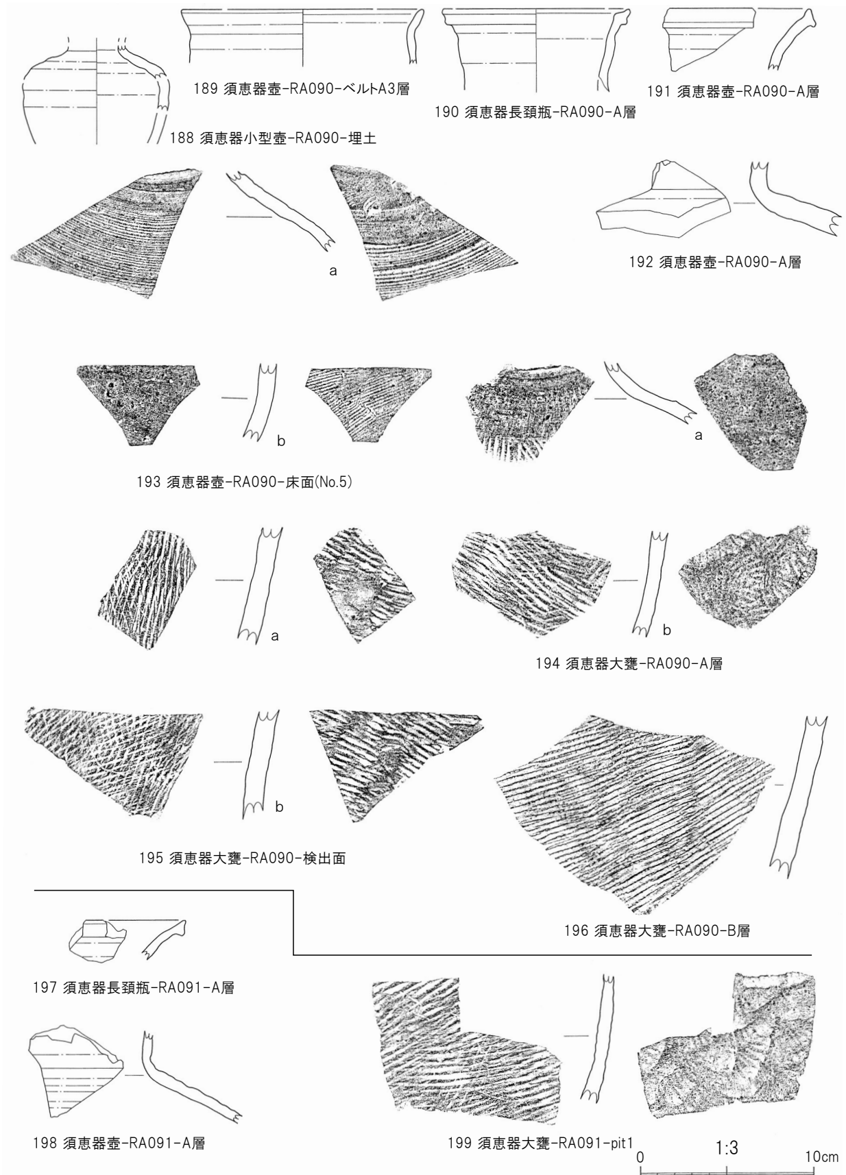
第88図 RA090出土土器(2), RA091出土土器
