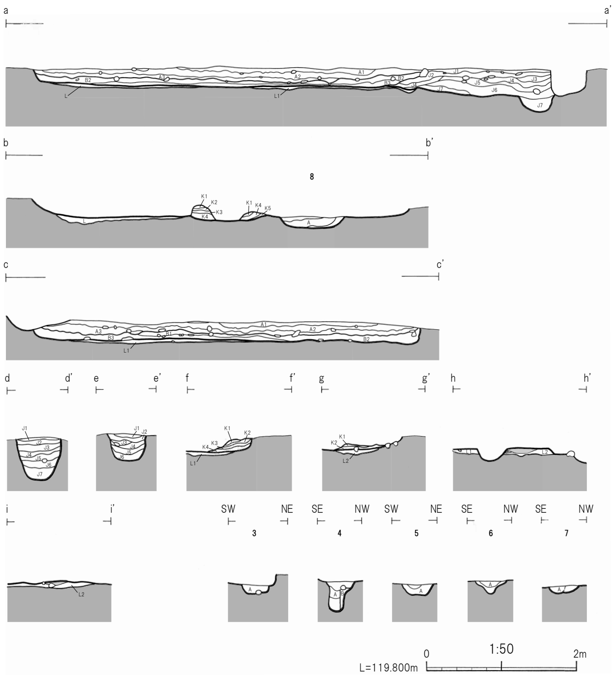
第32図 RA005竪穴建物跡(2)
