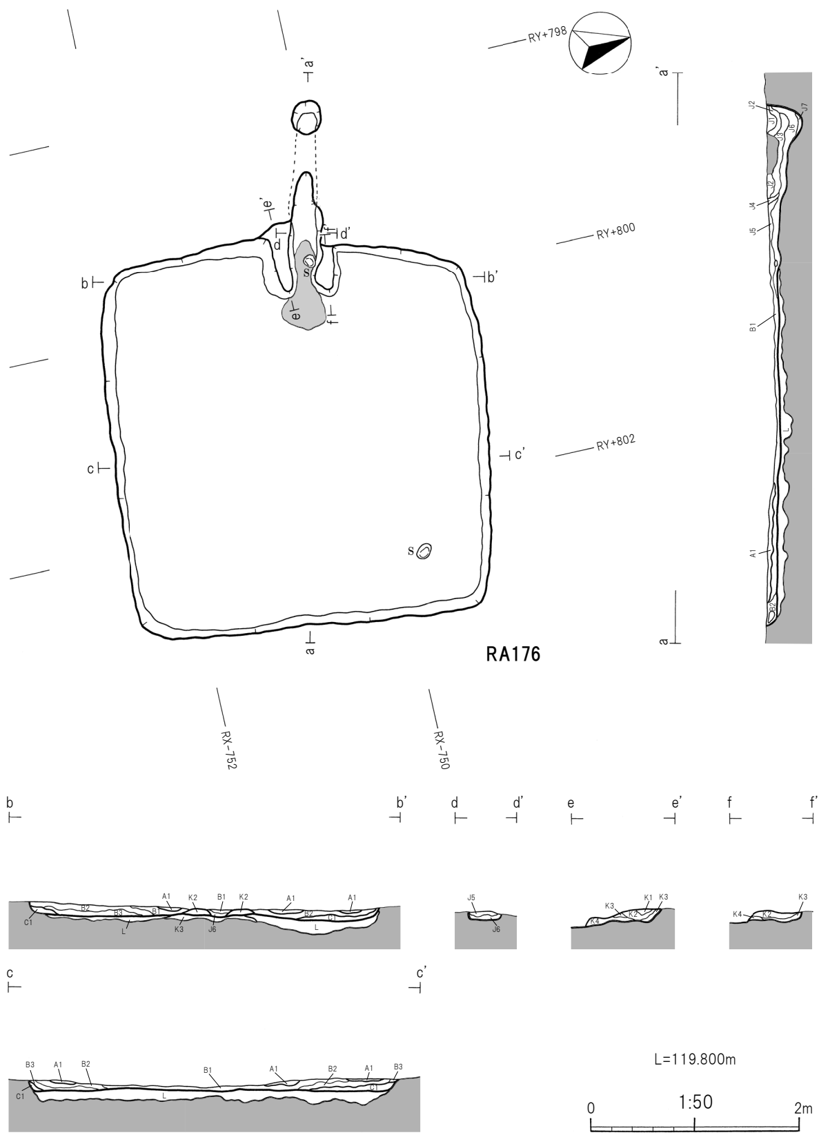
第61図 RA176竪穴建物跡
