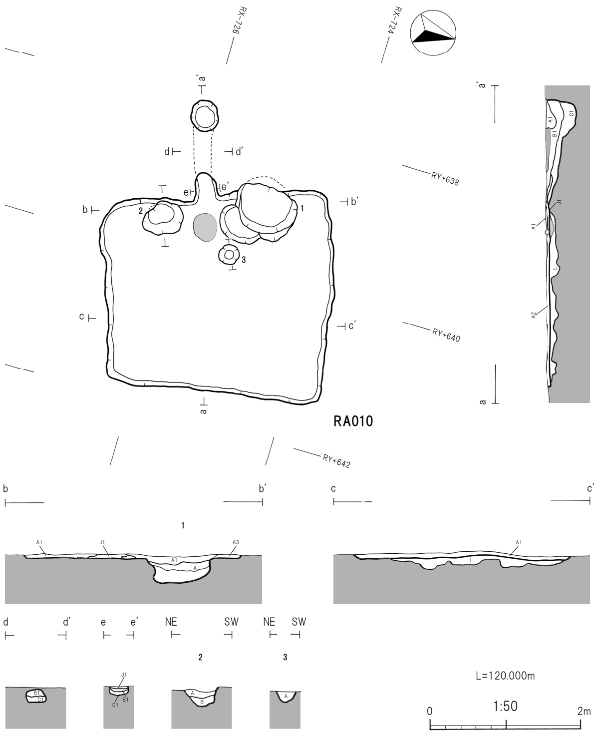
第35图 RA010竖穴建物跡
