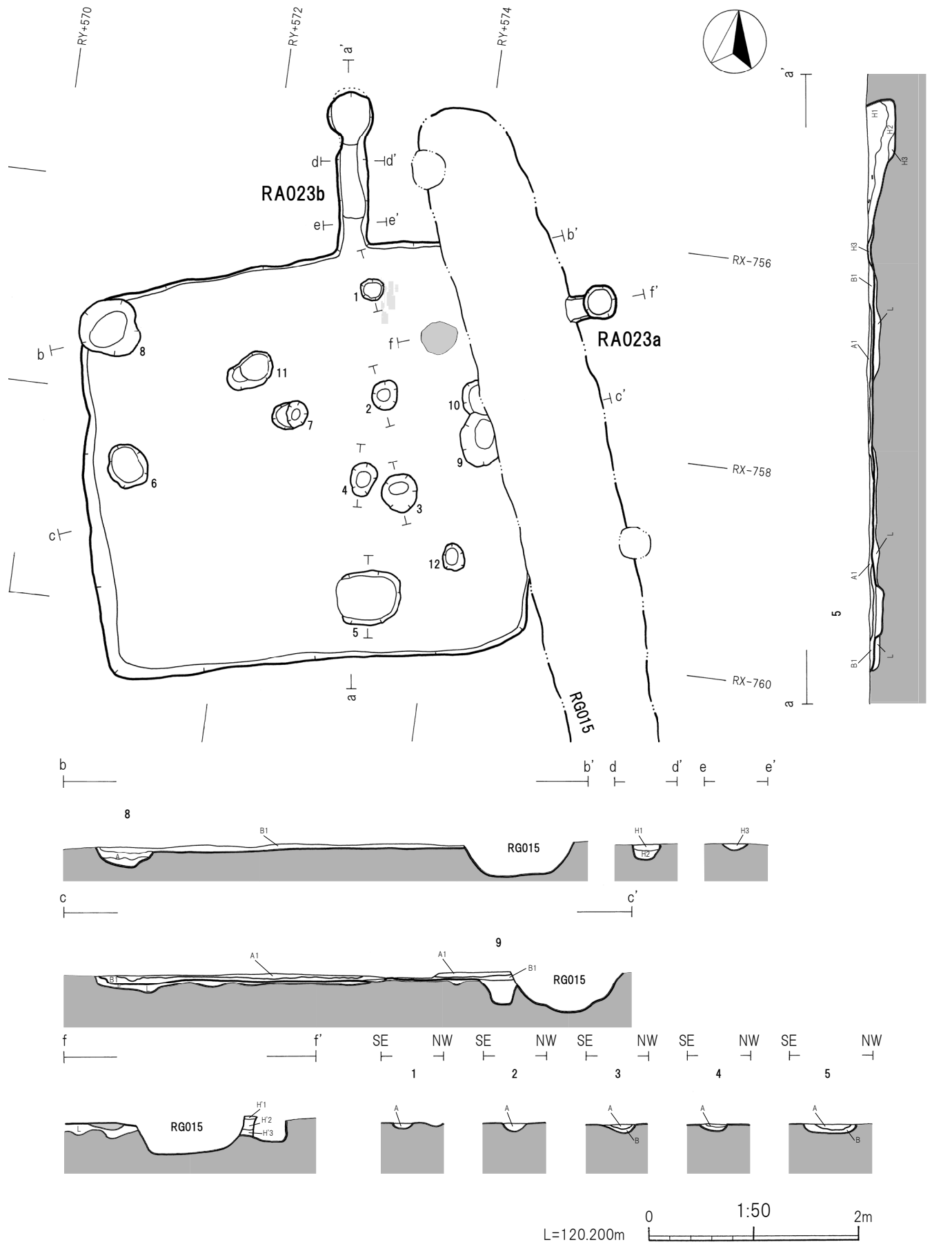
第48図 RA023竖穴建物跡
