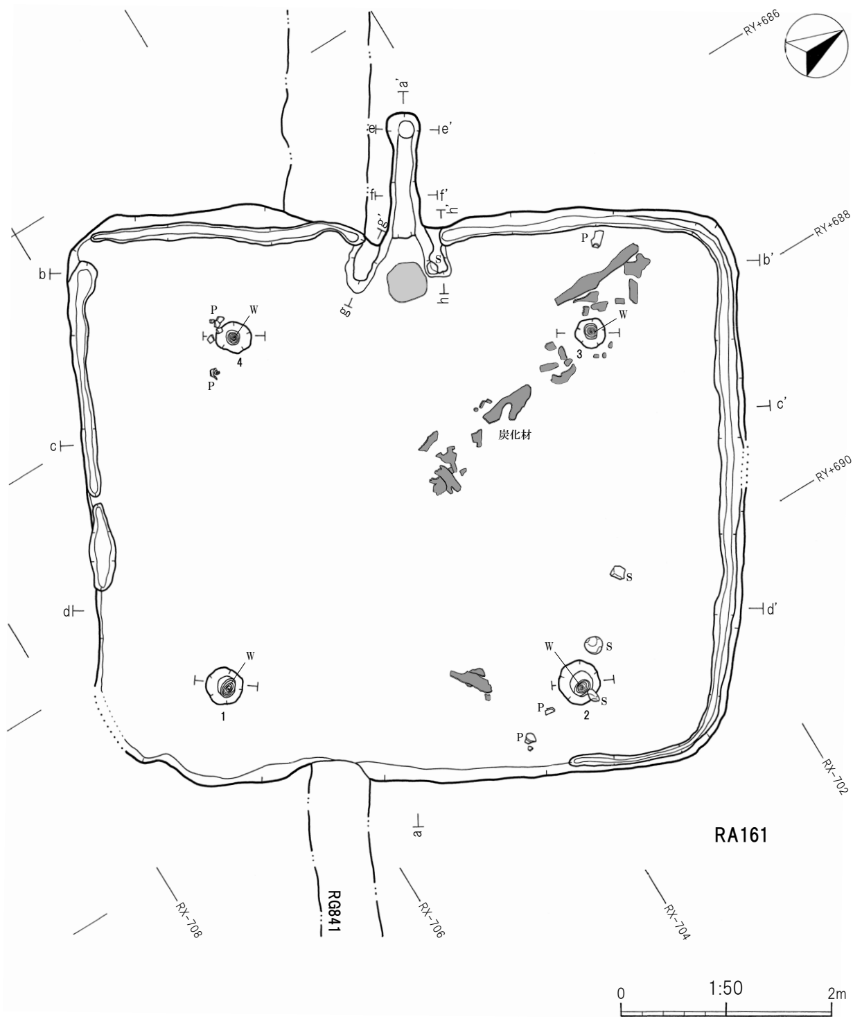
第50図 RA161竪穴建物跡(1)
