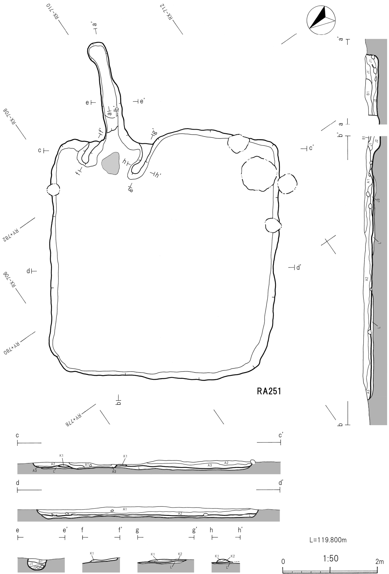
第62図 RA251竖穴建物跡
