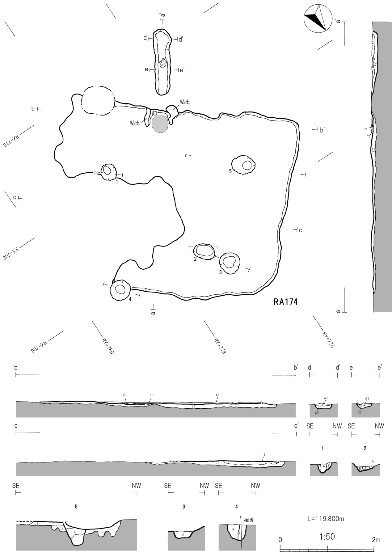
第59図 RA174竪穴建物跡
