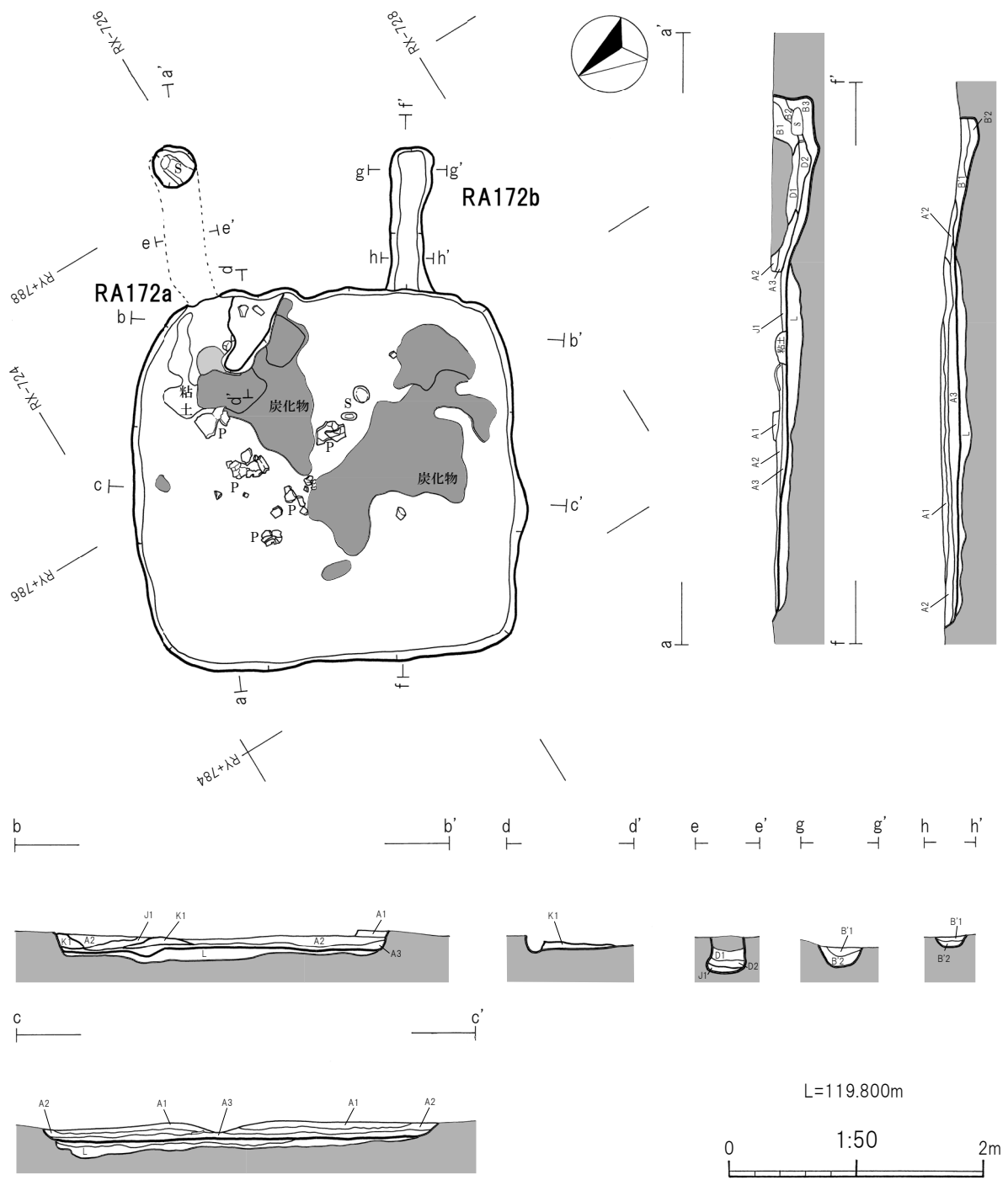
第58図 RA172竖穴建物跡
