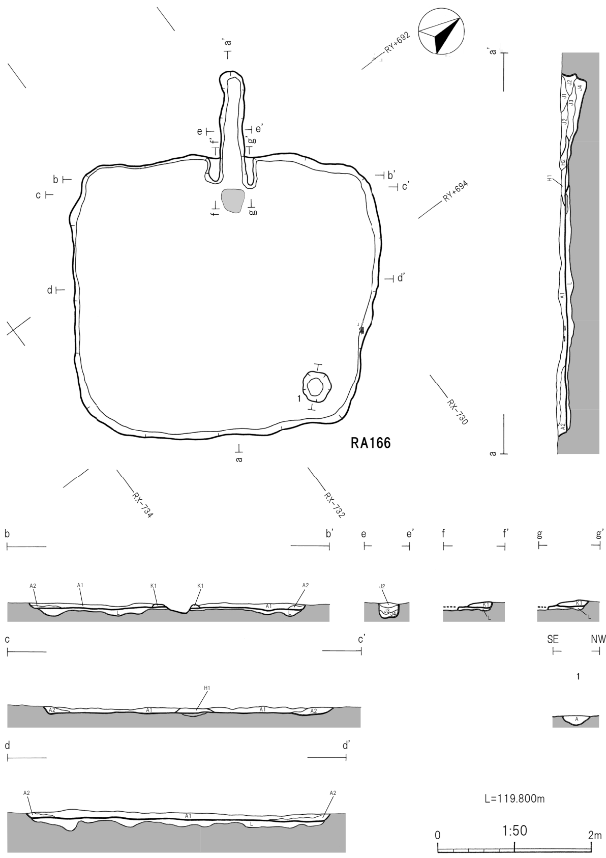
第54図 RA166竪穴建物跡
