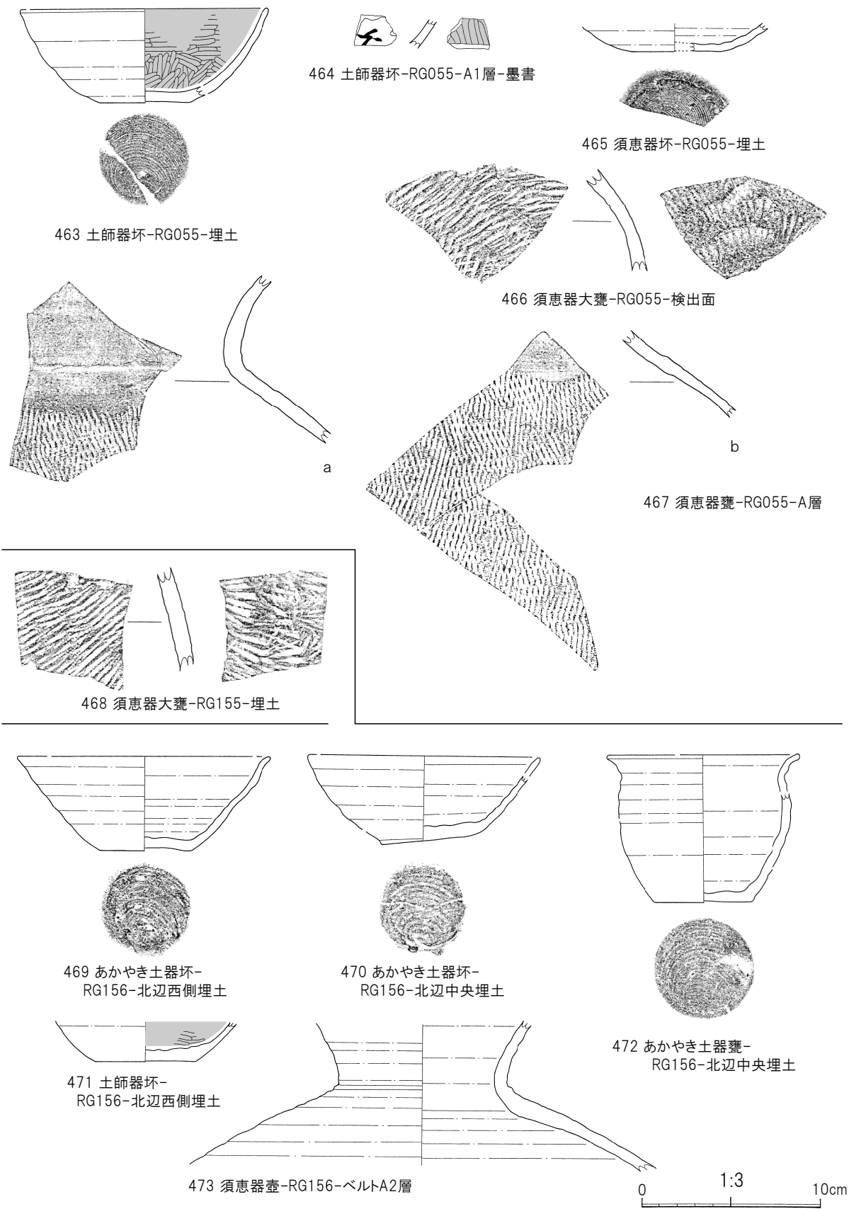
第118図 RG055・155・156出土土器
