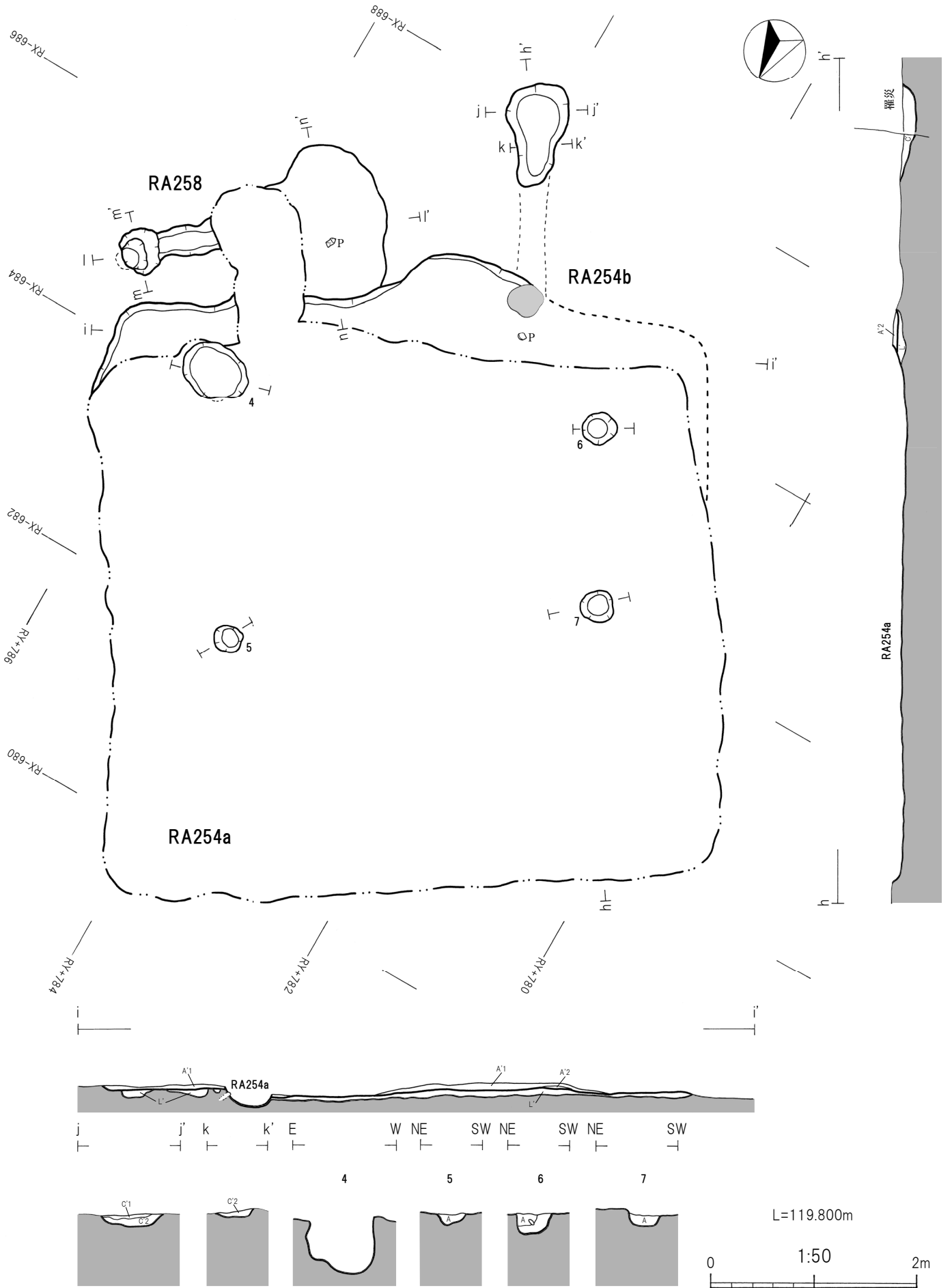
第67図 RA254・258竪穴建物跡(2)
