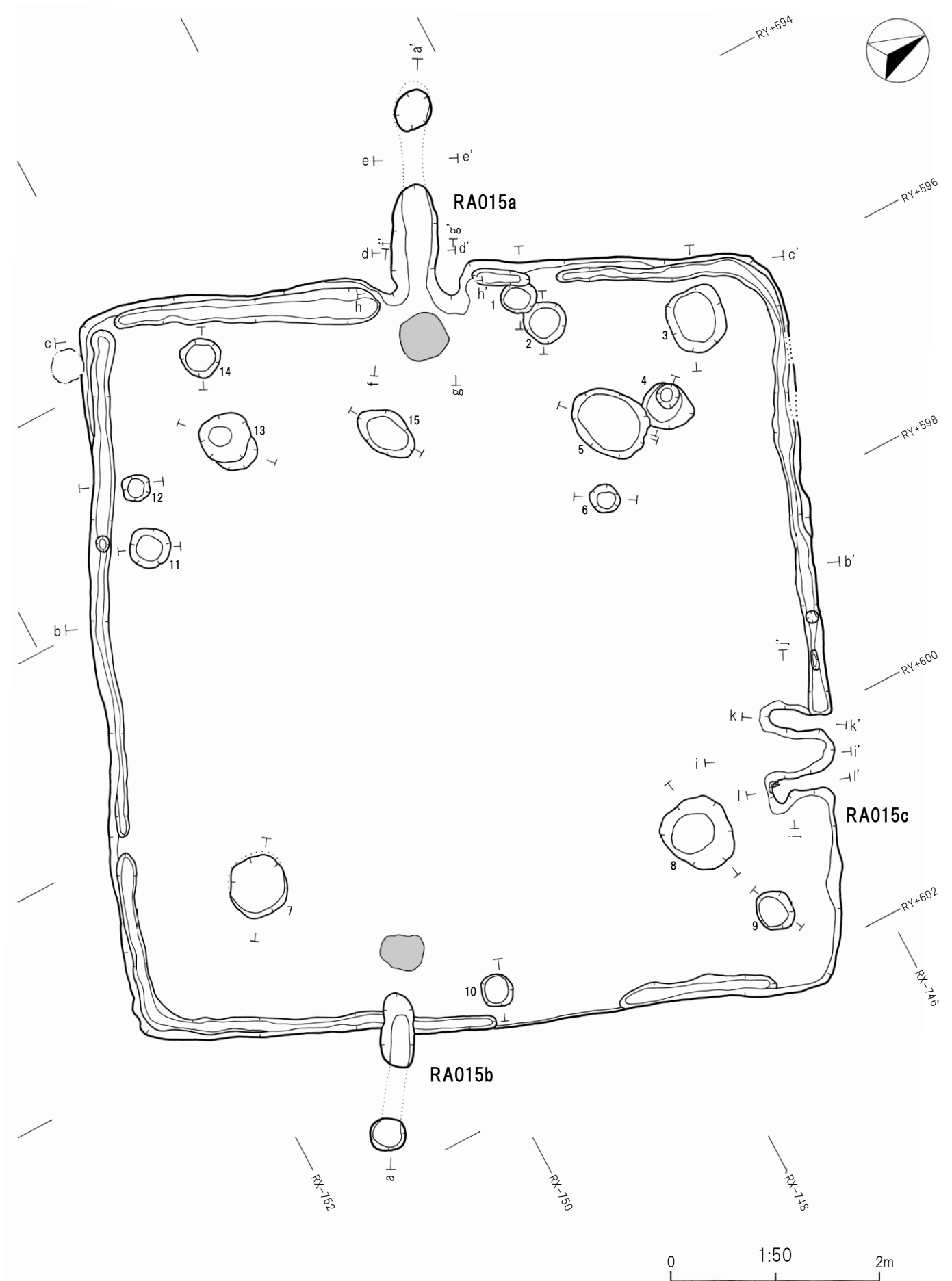
第41图 RA015竖穴建物跡(1)
