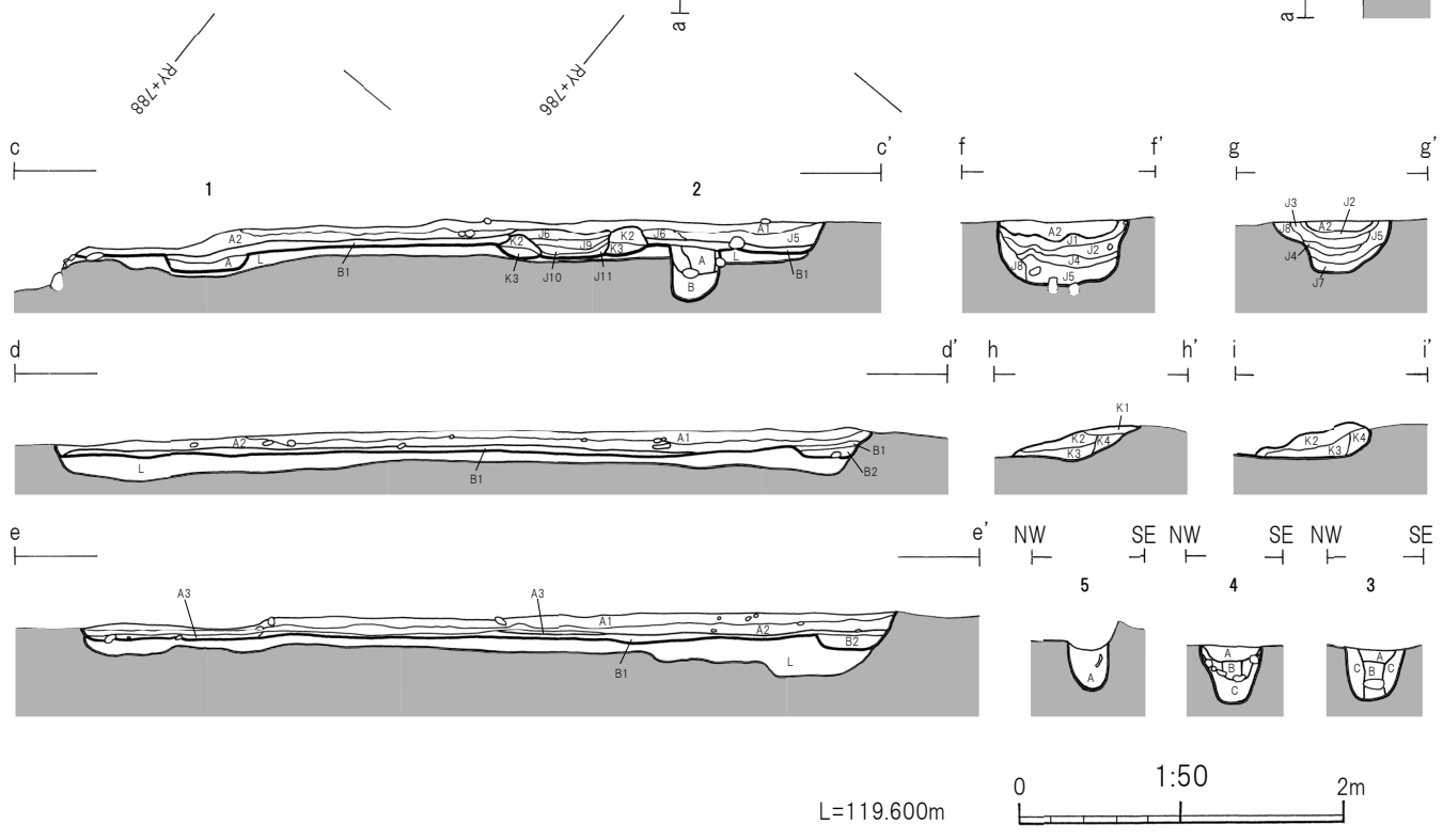
第64図 RA253竪穴建物跡
