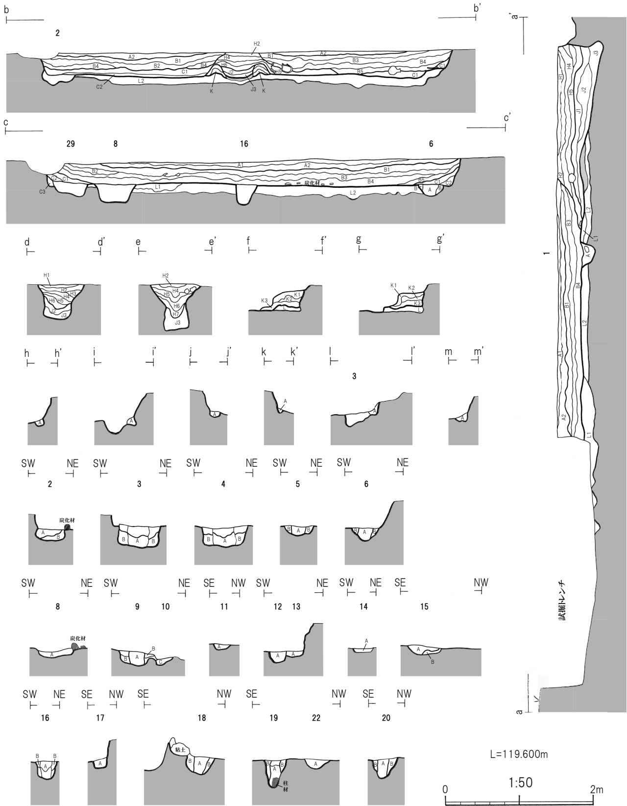
第27図 RA002竪穴建物跡(2)
