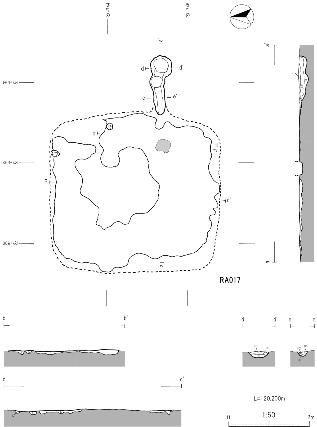
第43図 RA017竪穴建物跡
