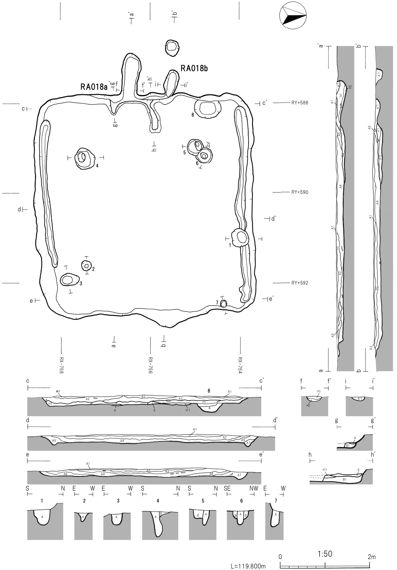
第44図 RA018竖穴建物跡(1)
