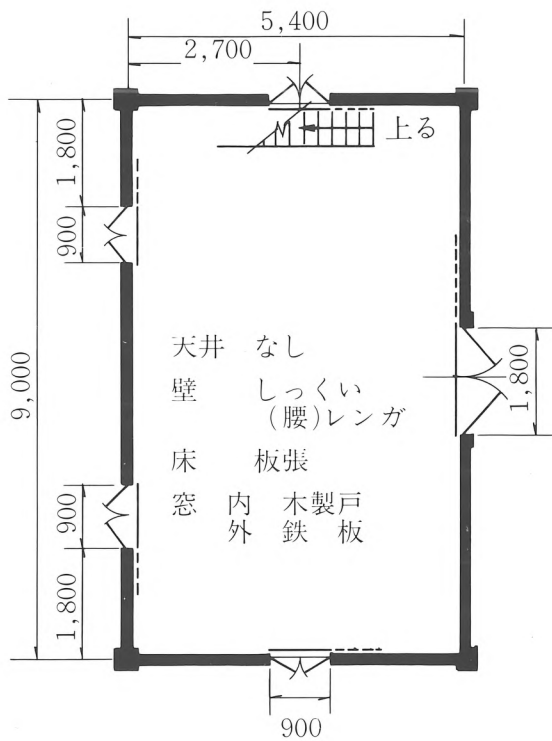
1階平面図
