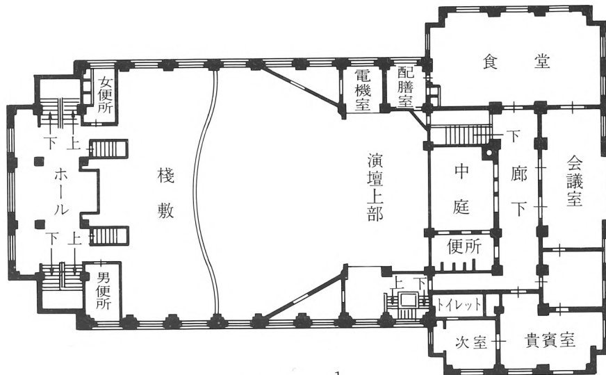
3階平面図 \frac{1}{400}
