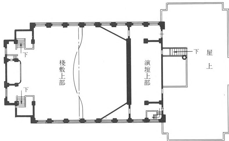
4階平面図 \frac{1}{400}
