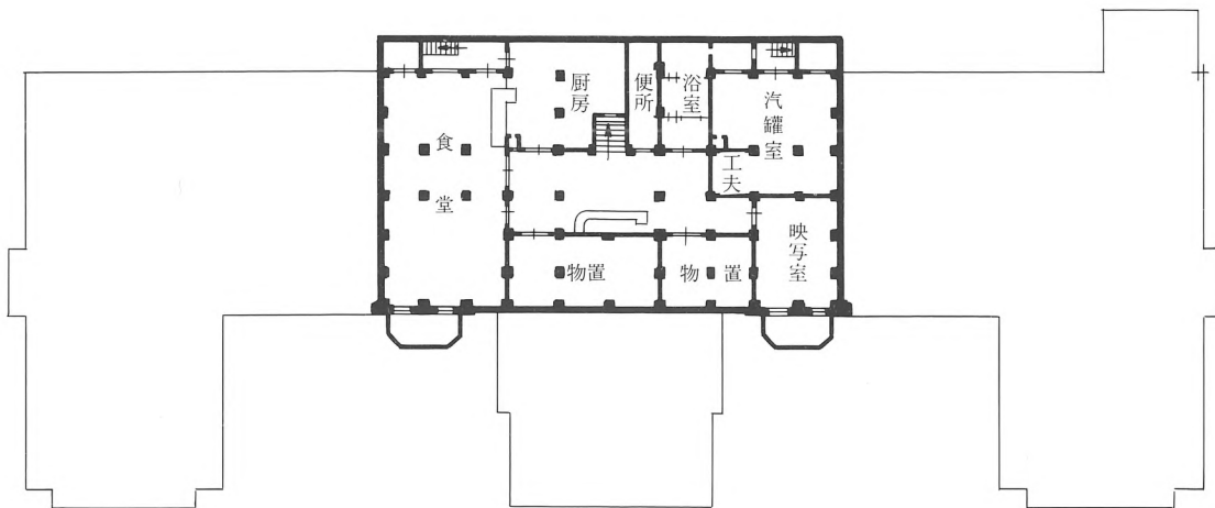
地階平面図(当初の部屋配置、以下同様)
