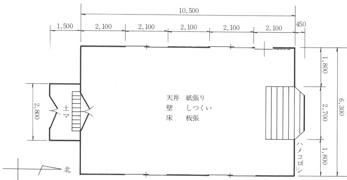
平面図
