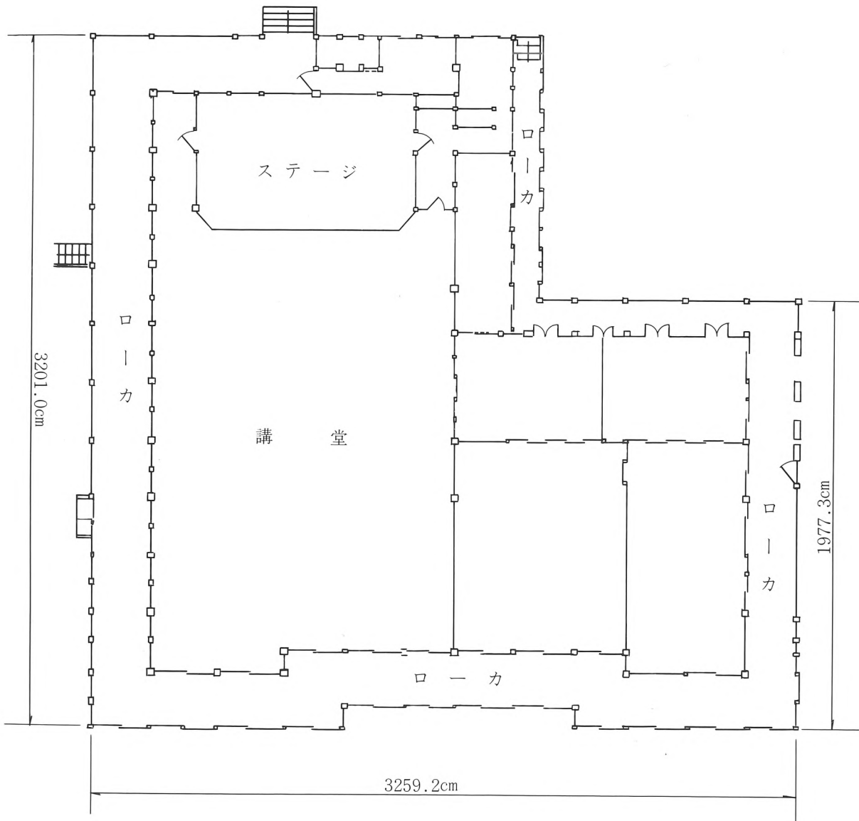
ブリュナー館（現状平面図）
