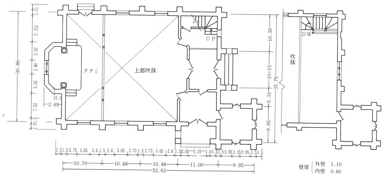
2階平面図
