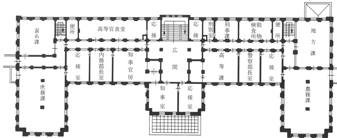
2階平面図
