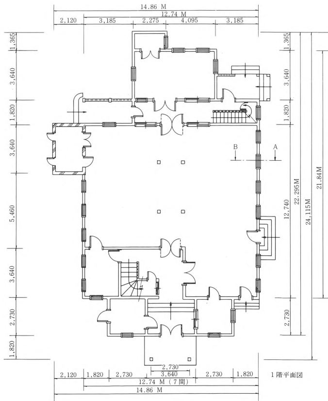
1階平面図
