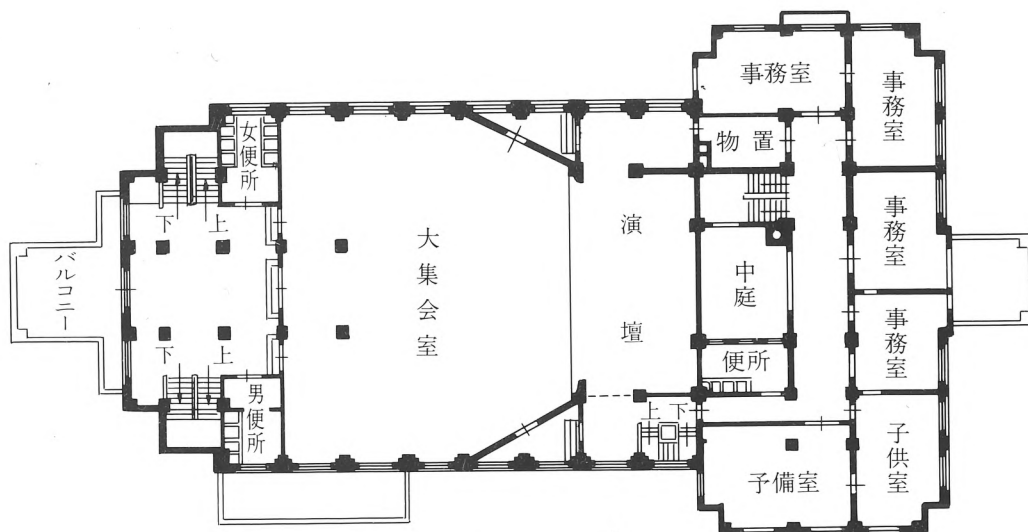
2階平面図 \frac{1}{400}
