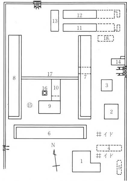
当初富岡製糸場建造物配置図
