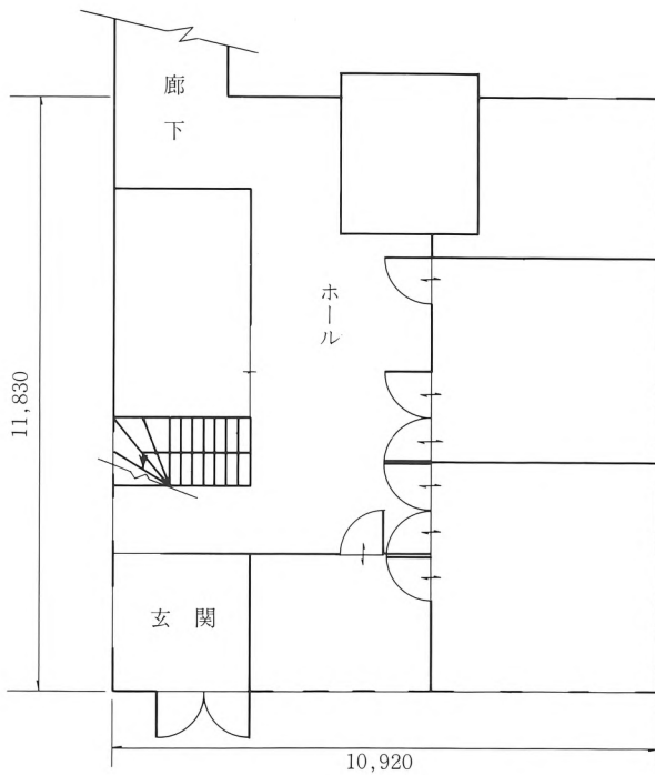
1階平面図
