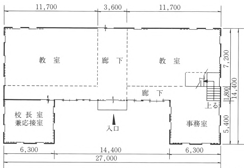
1階平面図 (推定、当初部屋配置)
