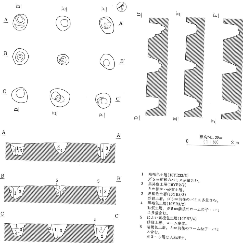
第8図 第232号掘立柱建物址実測図
