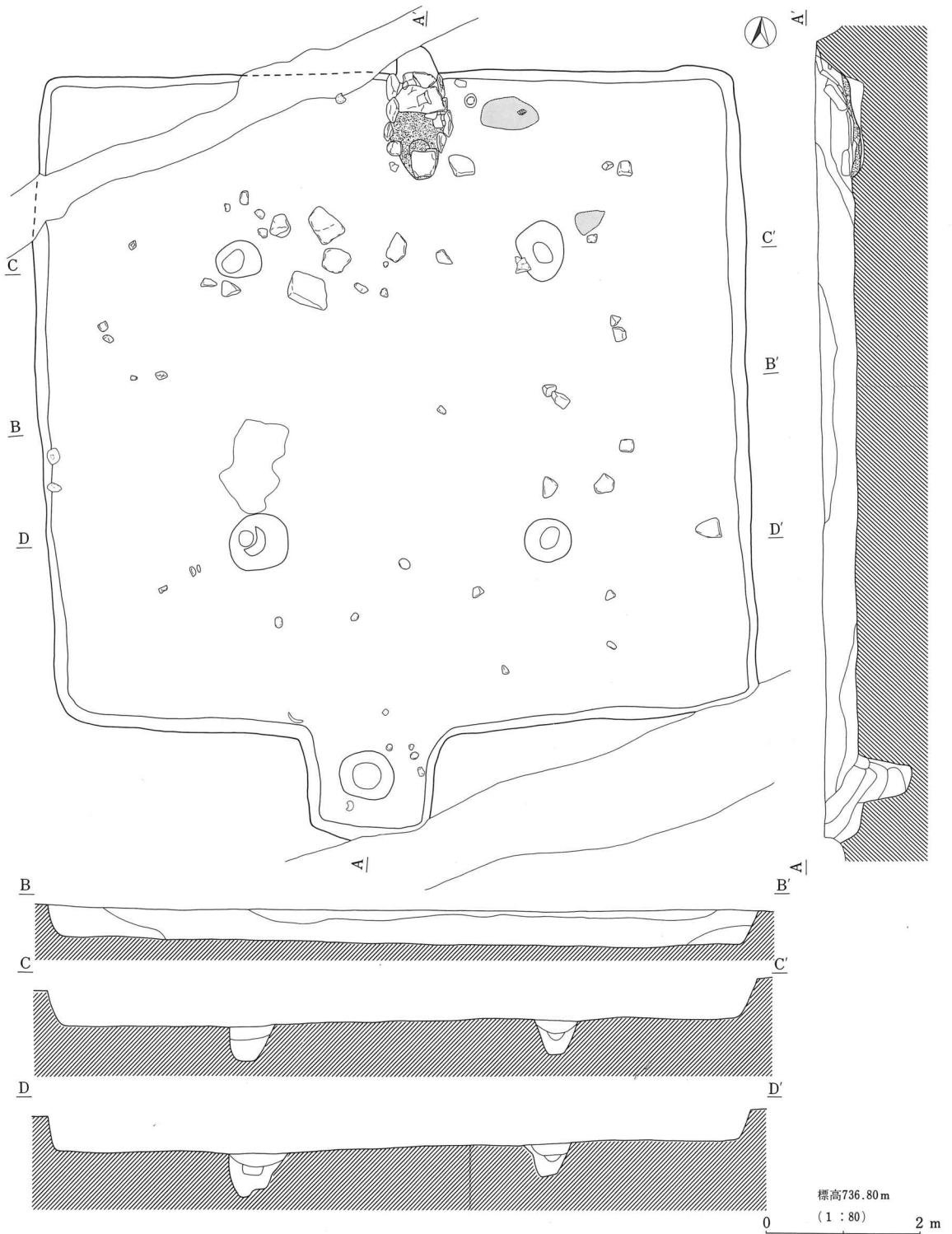
第6图 第162号住居址实测图
