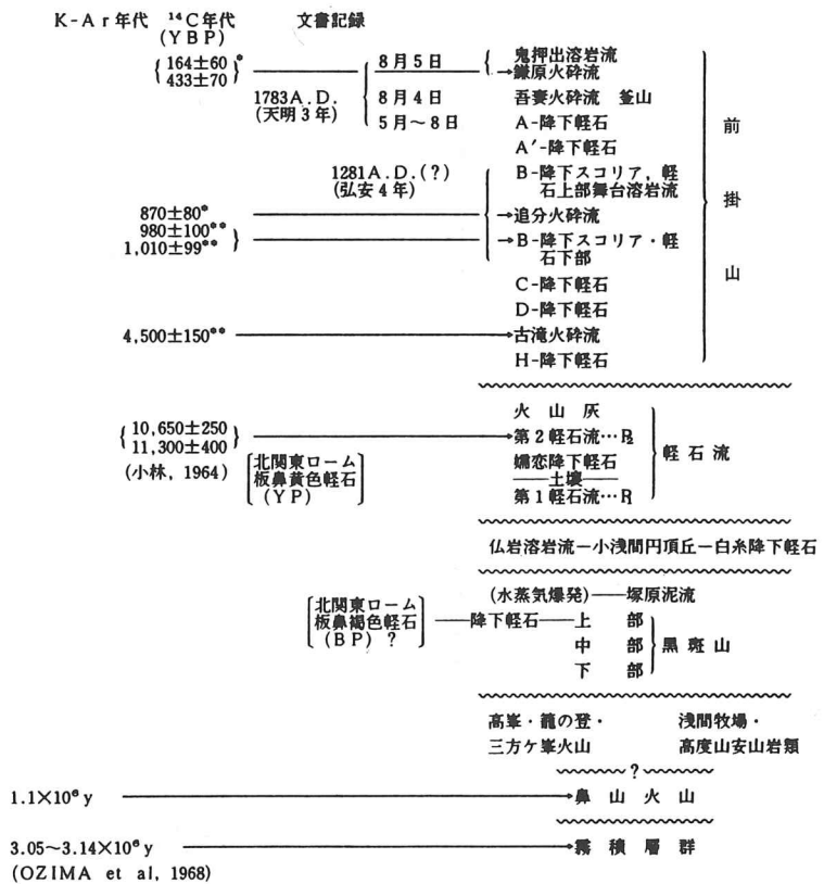
第2表 浅間火山を中心とした編年 (荒牧重雄著『浅間火山の地質』による。一部加除)
