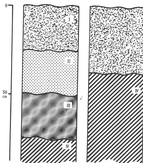
第5図 聖原遺跡I基本層序模式図
