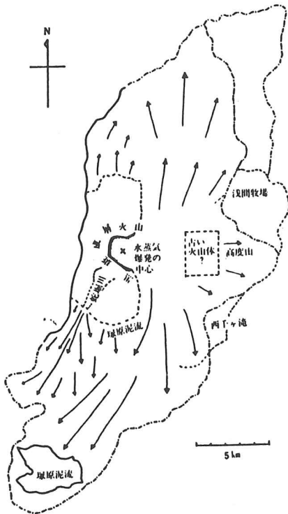
第3図 黒斑山東部の破壊によって生じた塚原泥流の流下した状態を示す図(荒牧重雄著『浅間火山の地質』による)
