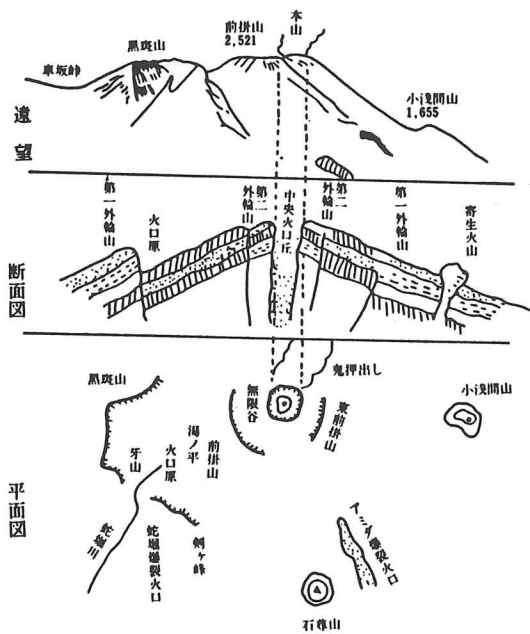
第2図 浅間山の形態と構造(白倉原図)
