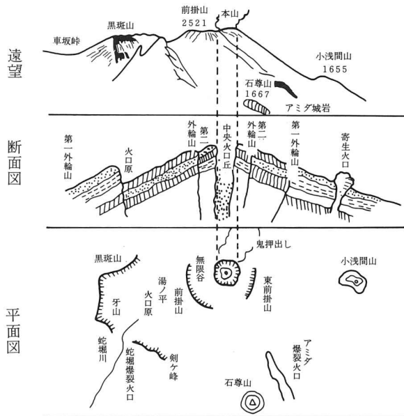
第2図 浅間山の形態と構造（白倉原図）
