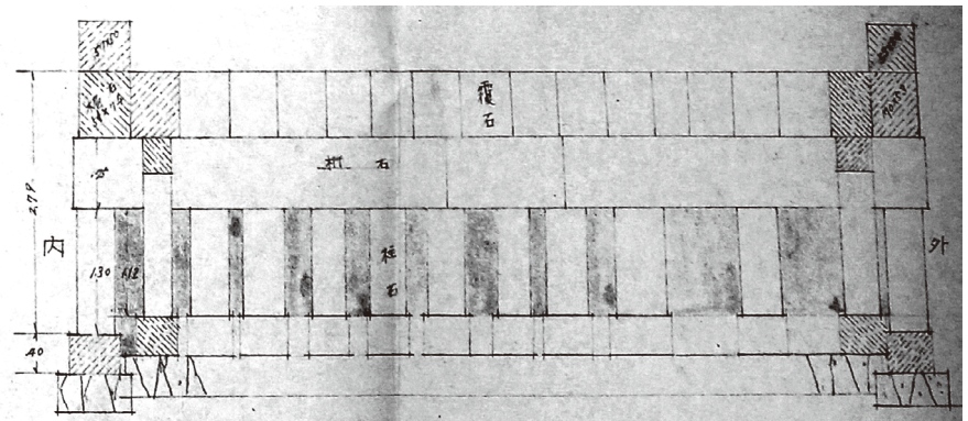
図3-13 石門縦断面図
