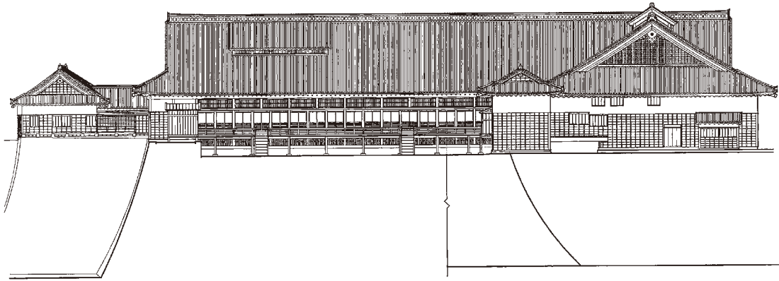
図 4-131 本丸御殿大広間・大台所・数寄屋南立面図
