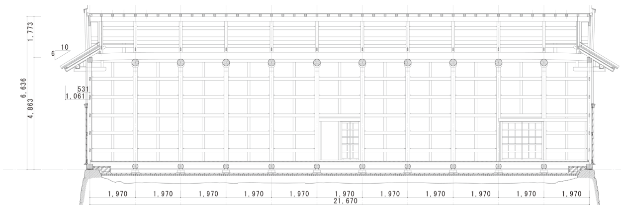
図 4-184 馬具櫓桁行断面図
