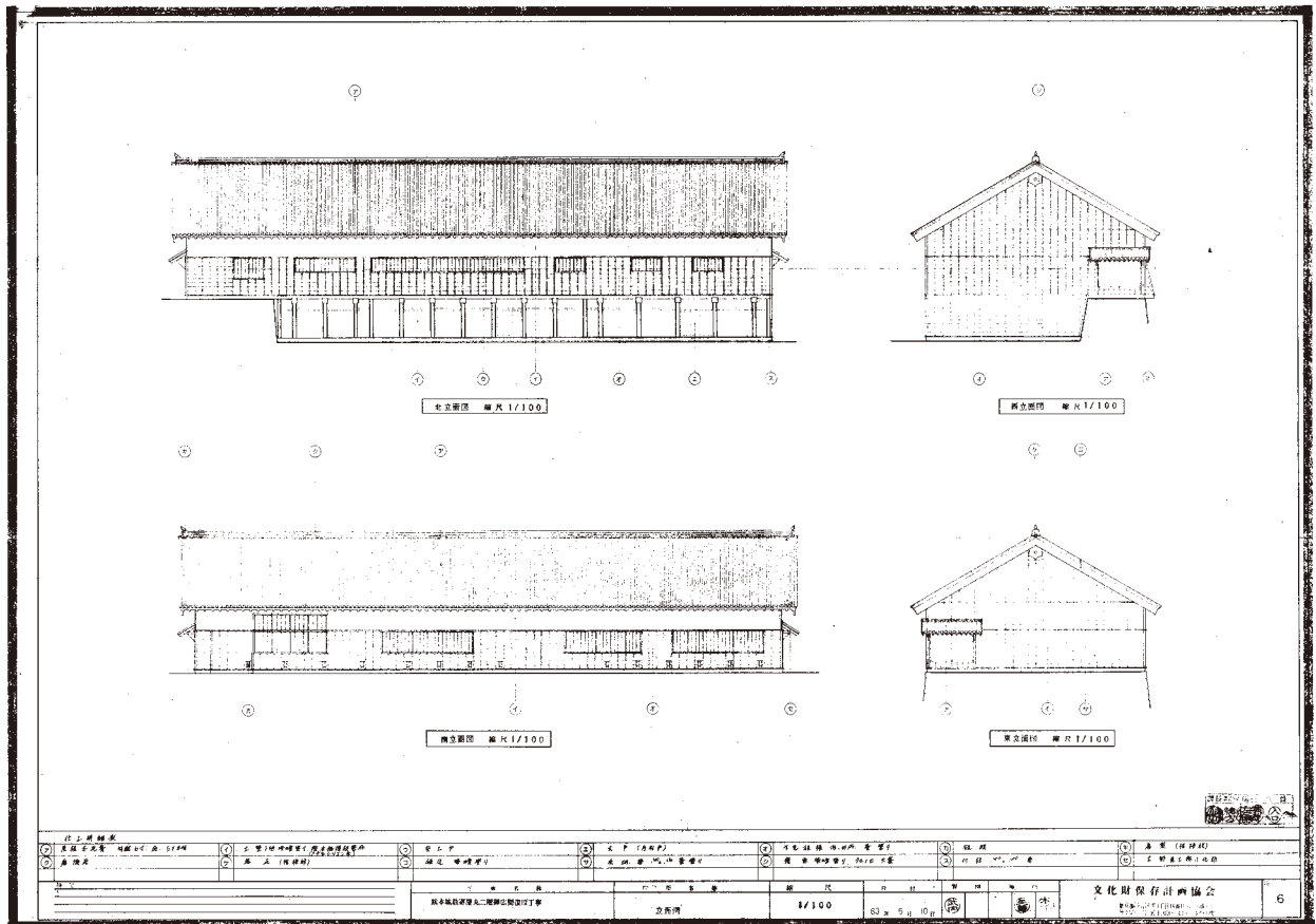
図 4-92 立面図
