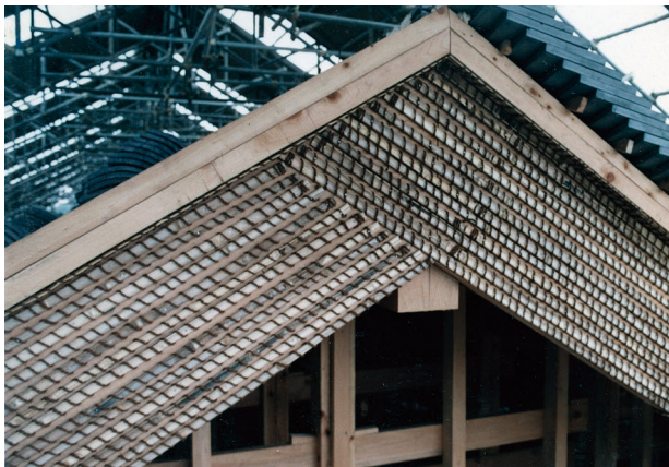
図 4-70 左官工事 西面破風板巻竹打完了
