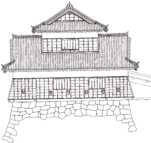
図 4-100 戌亥櫓西面立面図
