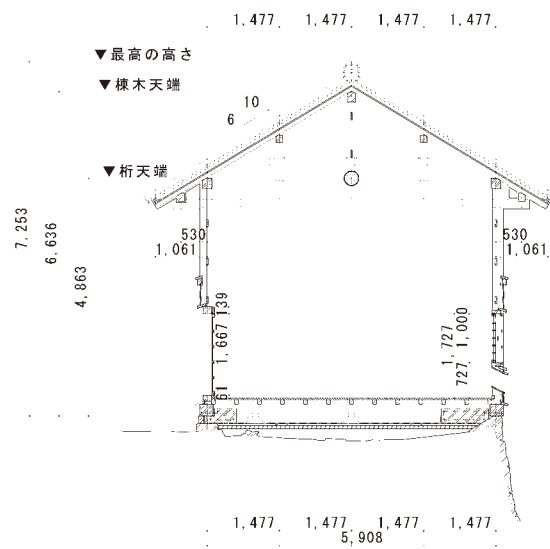
図 4-183 馬具櫓梁間断面図
