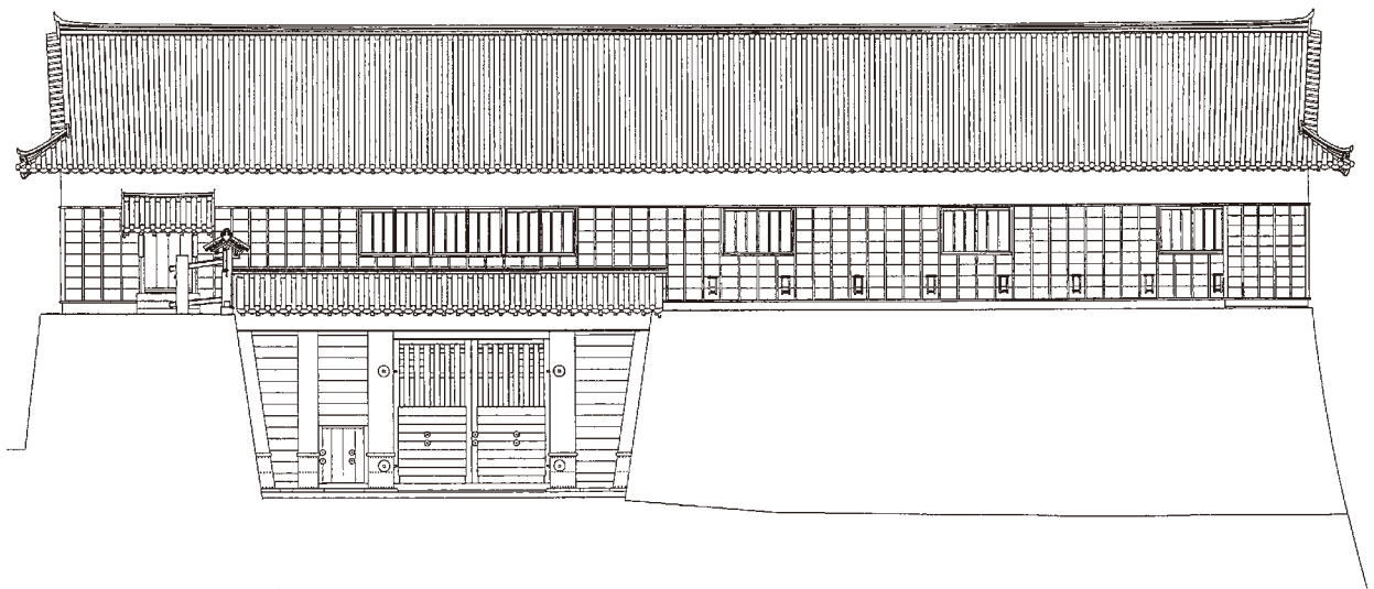
図 4-96 南大手門南面立面図
