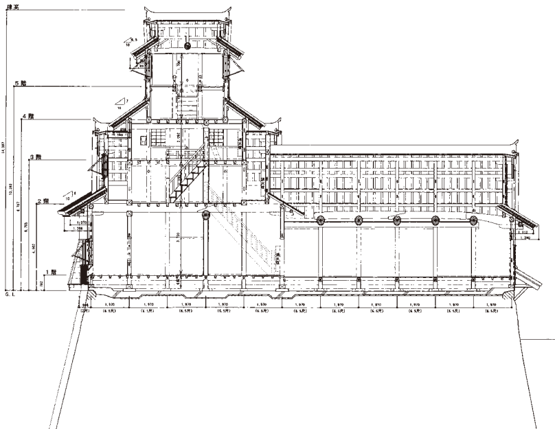
图 4-113 飯田丸五階櫓桁行断面図
