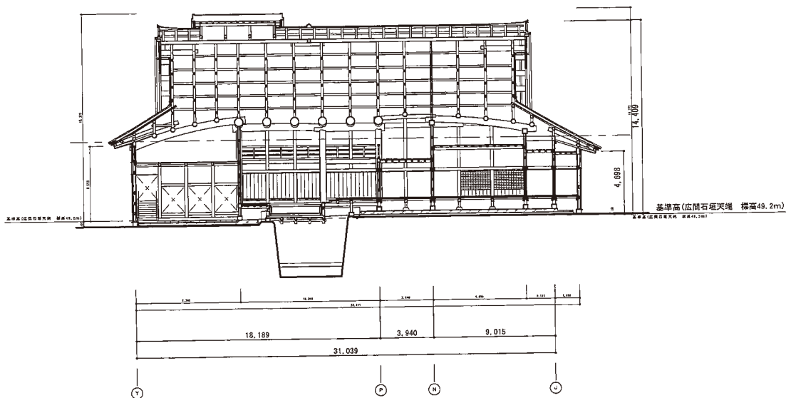
図 4-133 本丸御殿大台所桁行断面図
