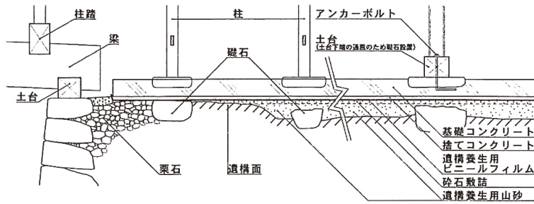
図 4-123 遺構養生方法概念図
