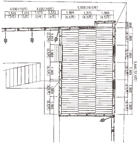
図 4-104 元太鼓櫓一階平面図
