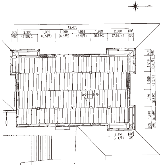
図 4-98 戌亥櫓一階平面図
