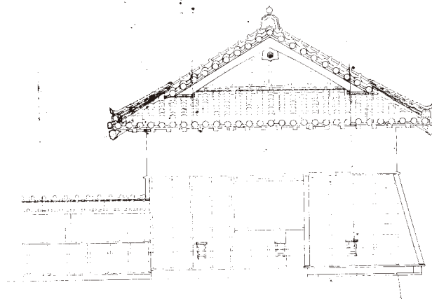
図 4-5 平御櫓復元南立面図
