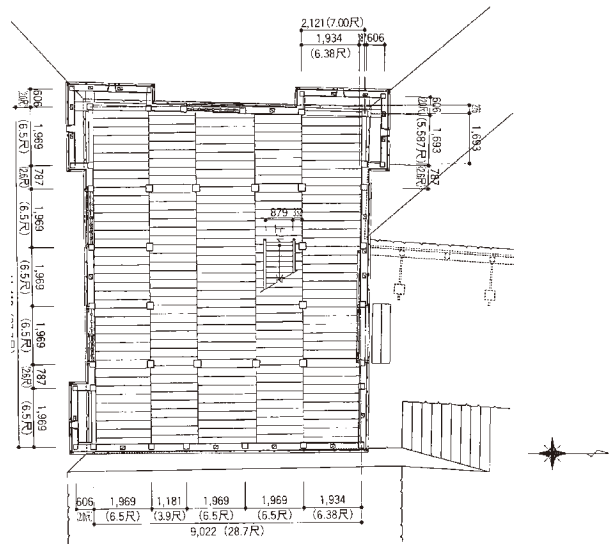
図 4-99 未申櫓一階平面図
