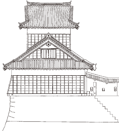
図 4-101 未申櫓東面立面図
