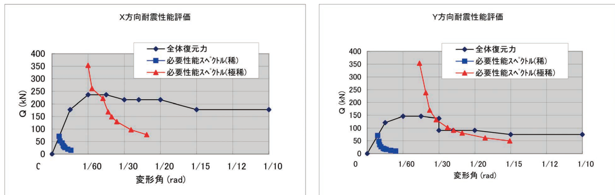
図 4-141 限界耐力計算による耐震性能評価
