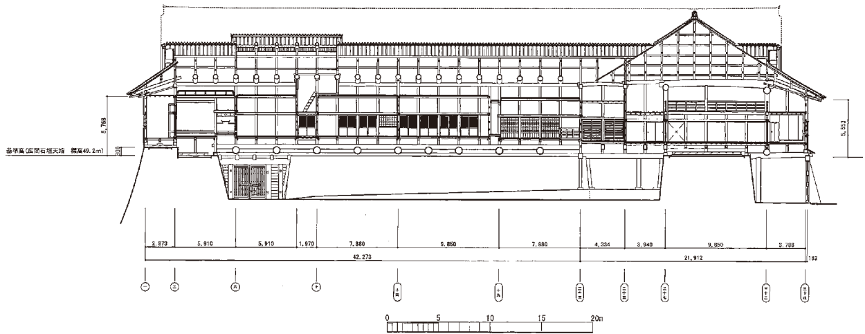
図 4-132 本丸御殿大広間桁行断面図
