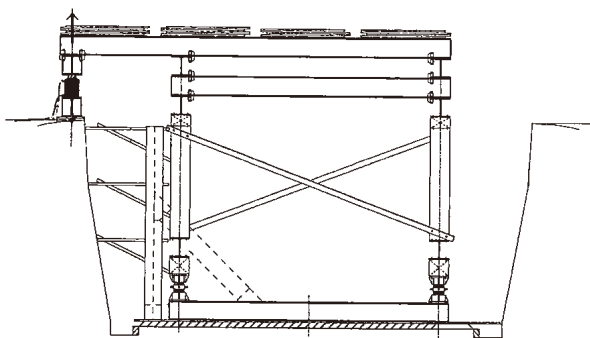
図 4-124 石垣載荷試験の載荷台
