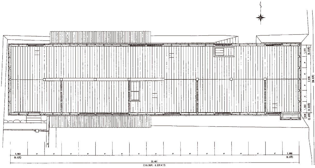
図 4-95 南大手門二階平面図
