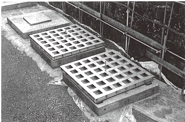
図 4-125 闇り通路ステンレス基礎
