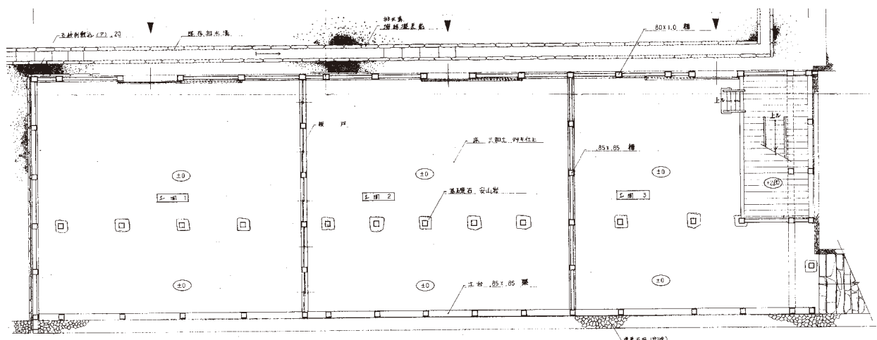
図 4-18 1階平面図
