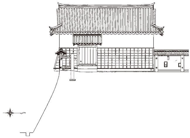
図 4-105 元太鼓櫓南面立面図
