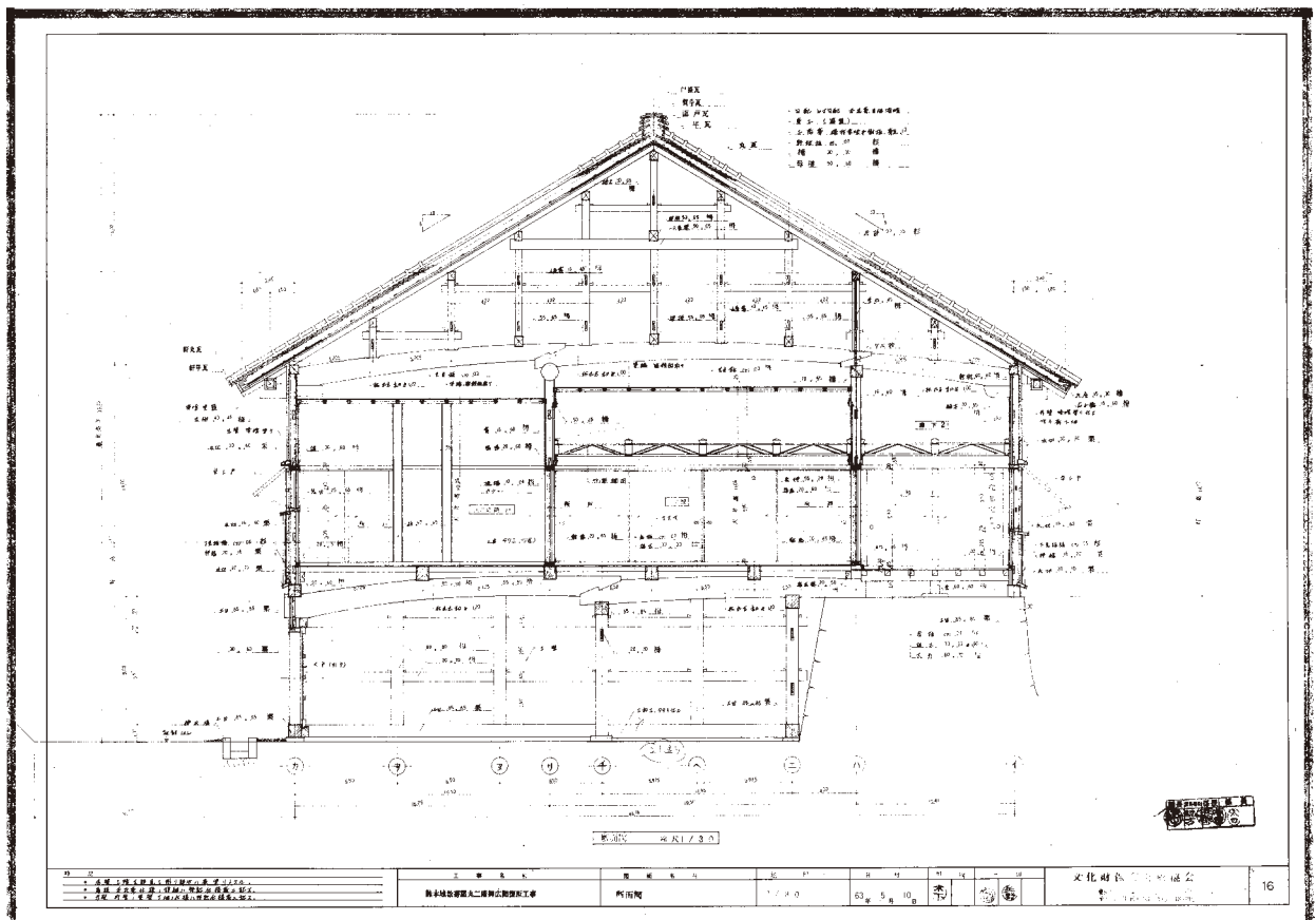
図 4-93 梁間断面詳細図
