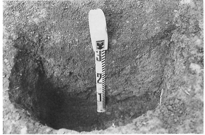
Pit 2 セクション (W→)
