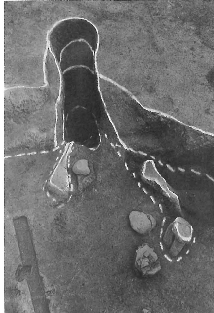
カマド完掘 (W→)
