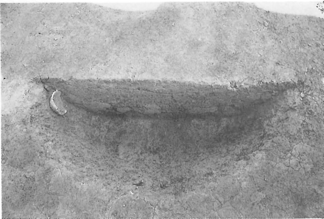
Pit33セクション (S→)
