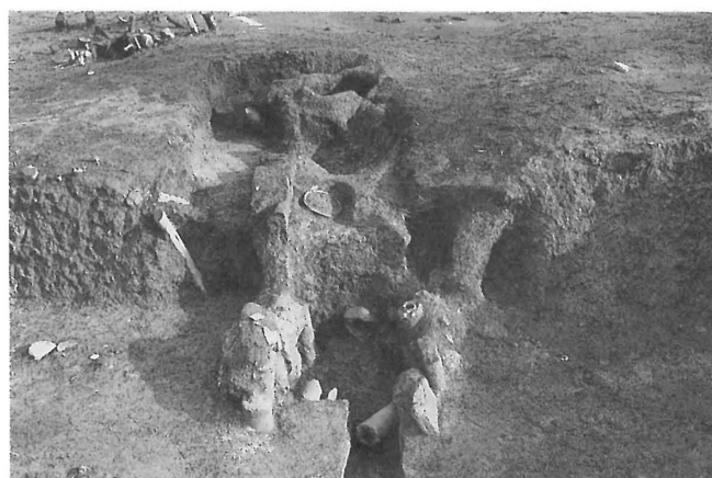
カマドA遺物出土状況 (N→)
