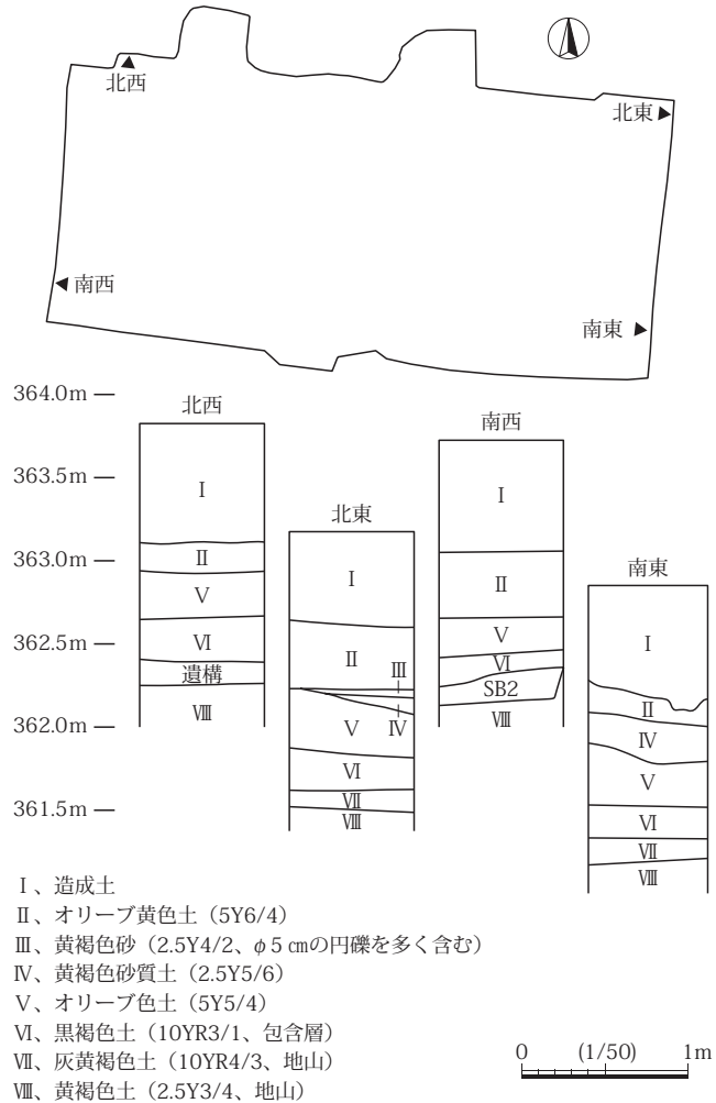
図6 基本層序
