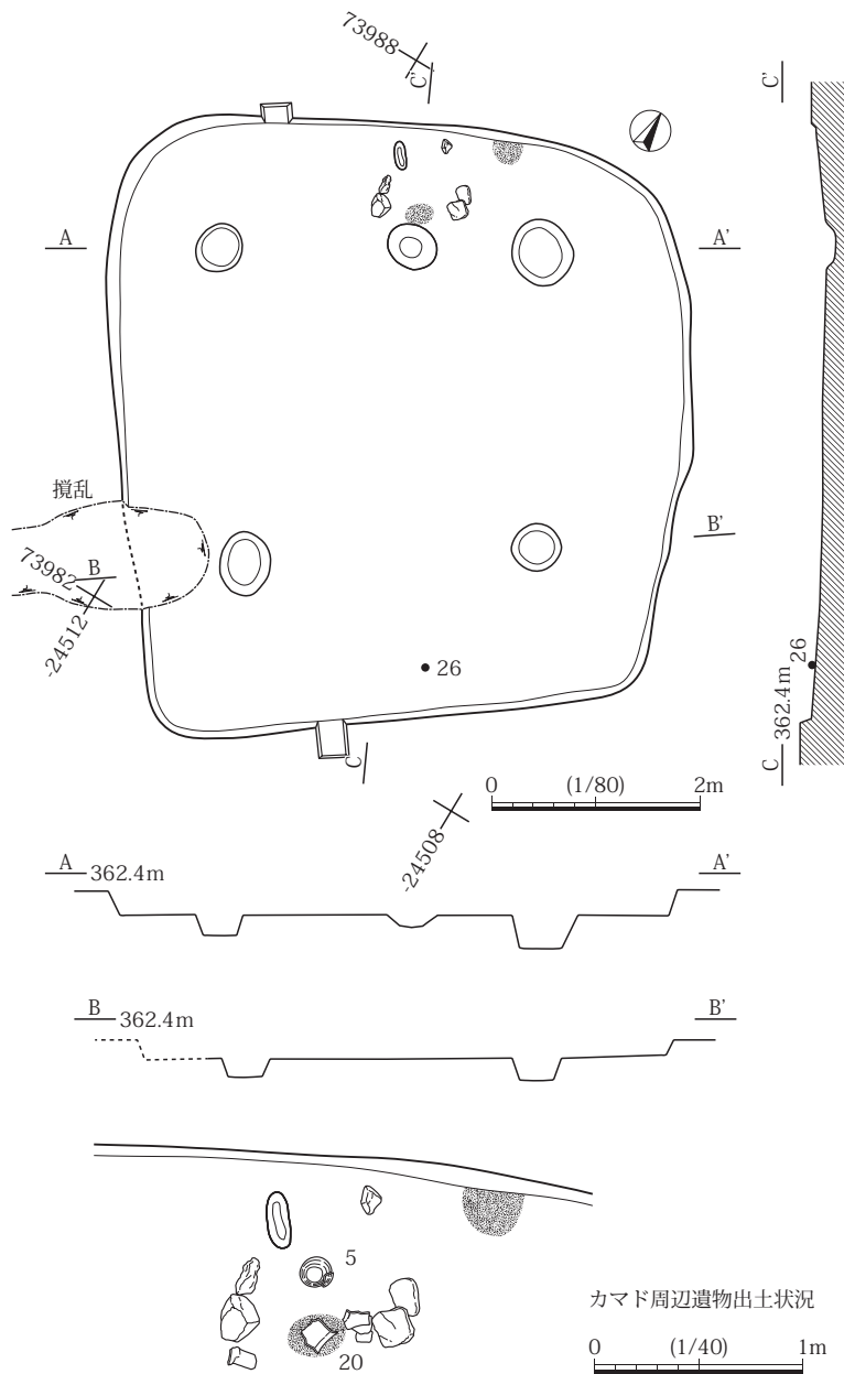
図24 SB 6 実測図
