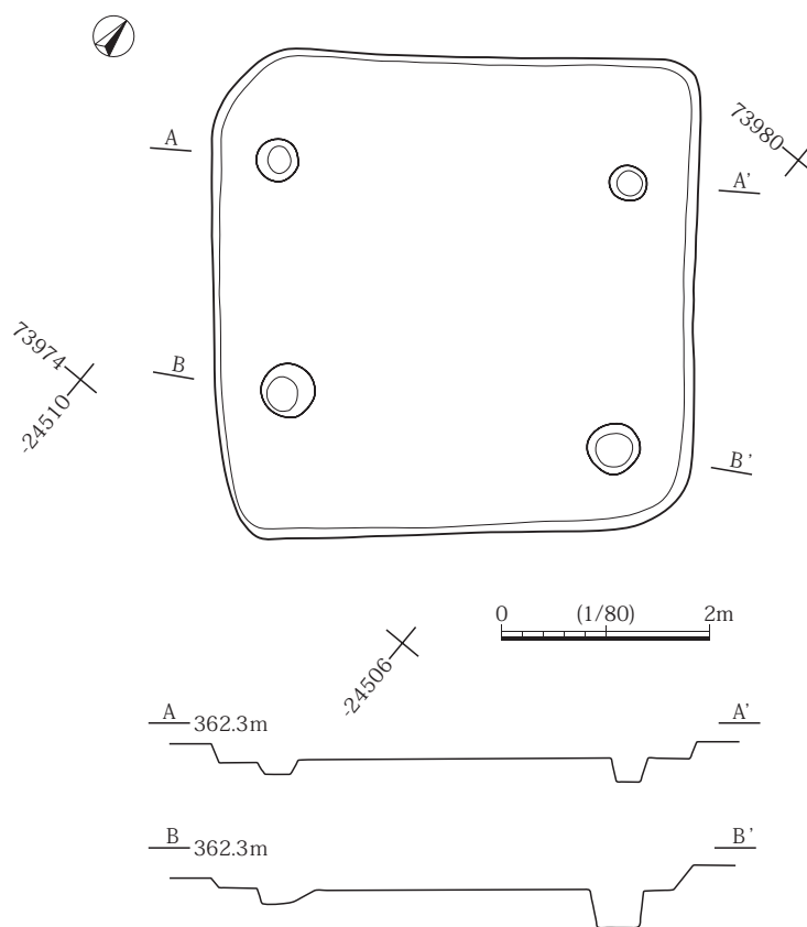
図20 SB 4 実測図
