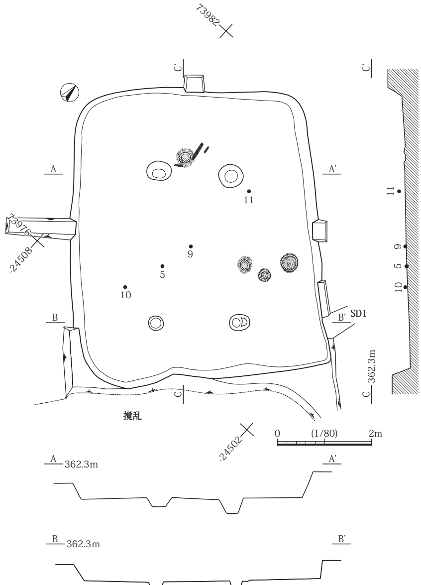
図10 SB13実測図
