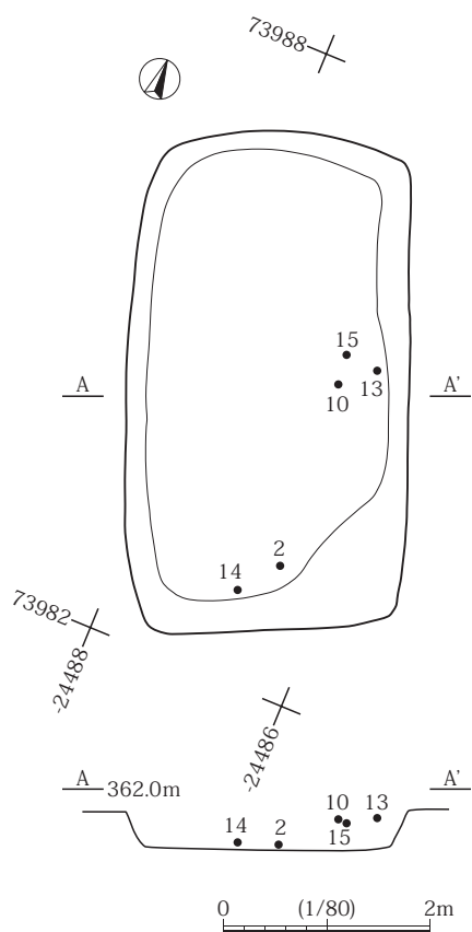
図12 SX 1 実測図
