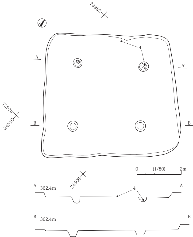
図22 SB 5 実測図
