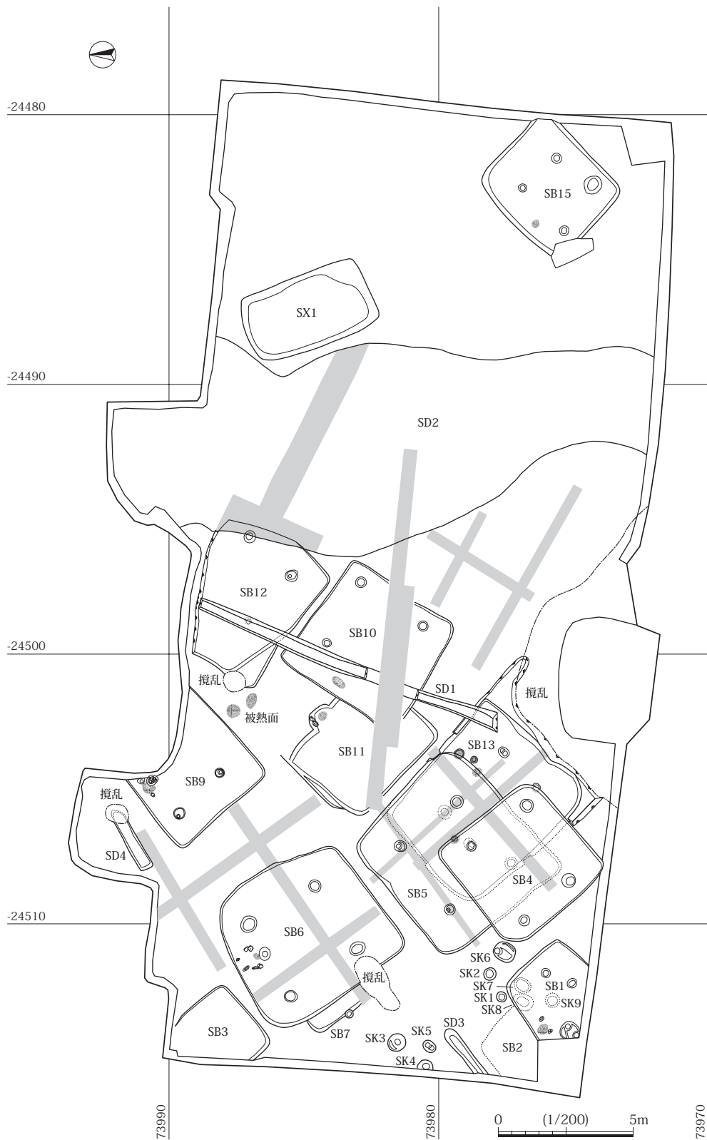
図7 遺構配置図
