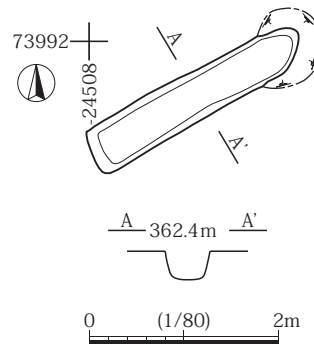
図14 SD 4 実測図
