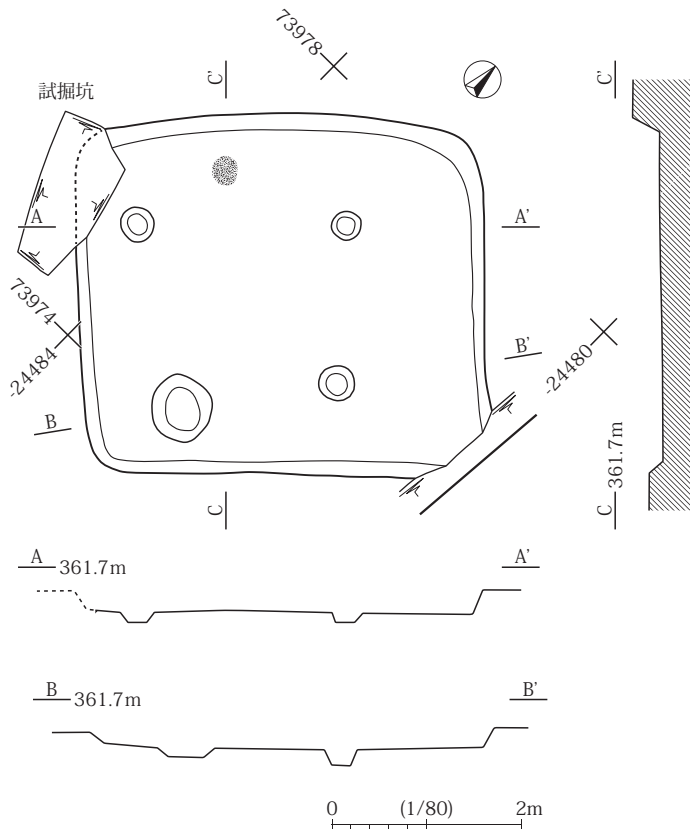
図35 SB15実測図
