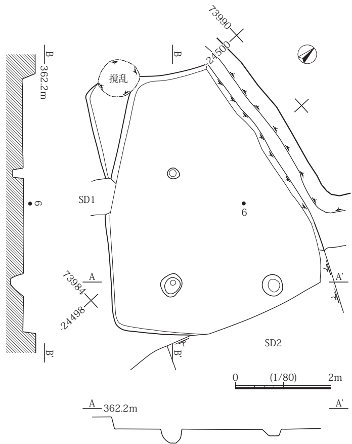
図8 SB12実測図
