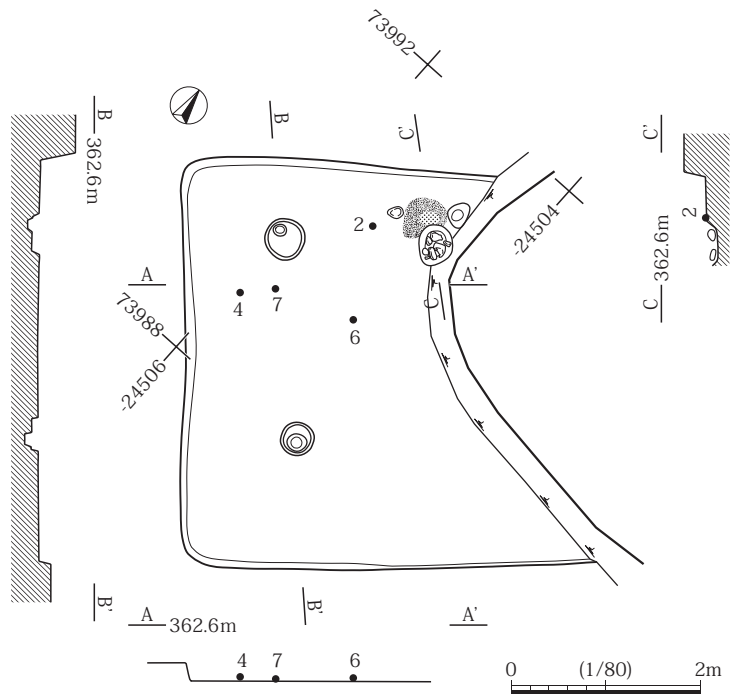
図29 SB 9 実測図
