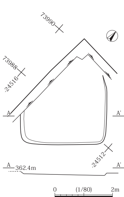
図18 SB3実測図
