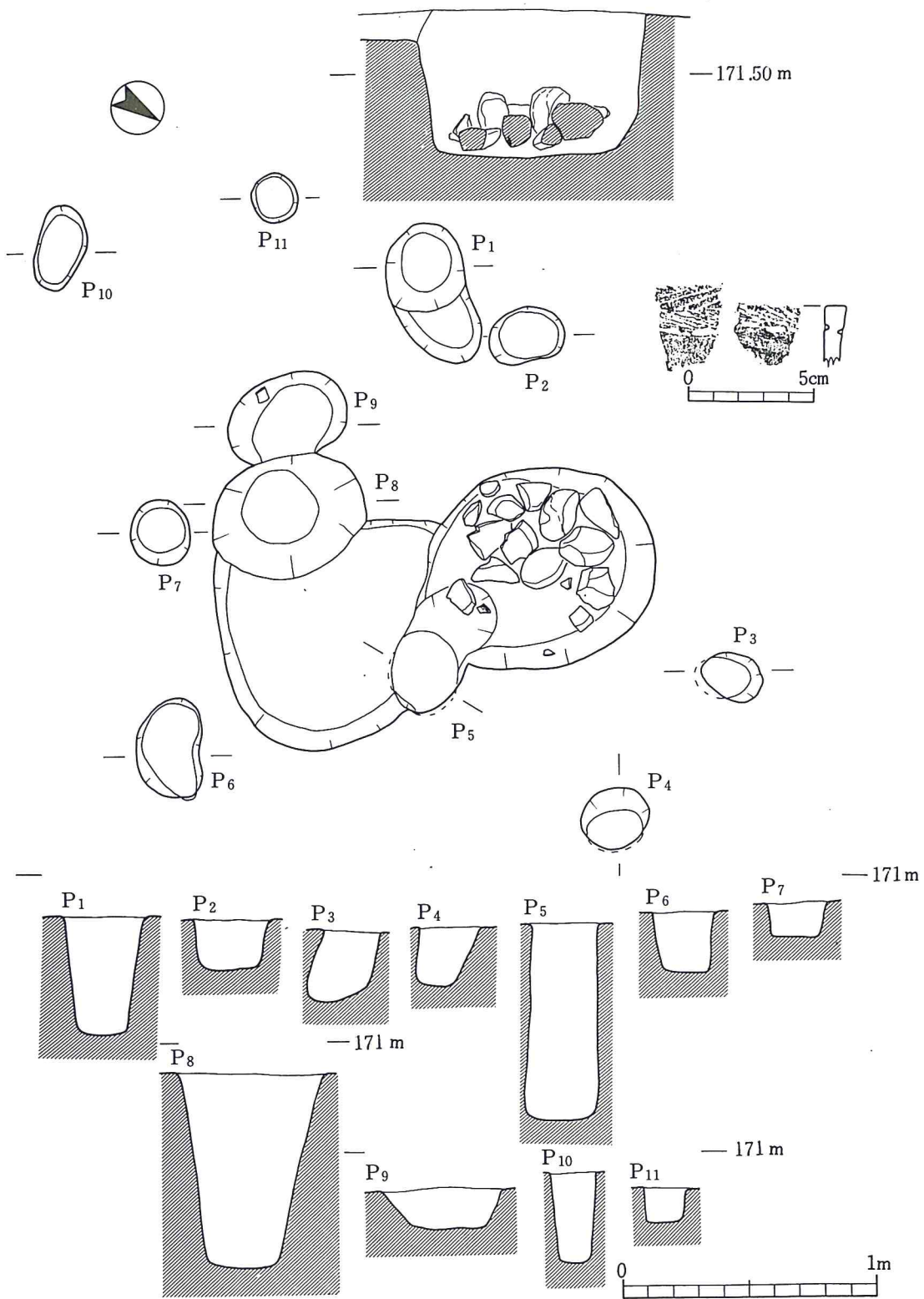
第6图 1号土坑平面图·断面图
