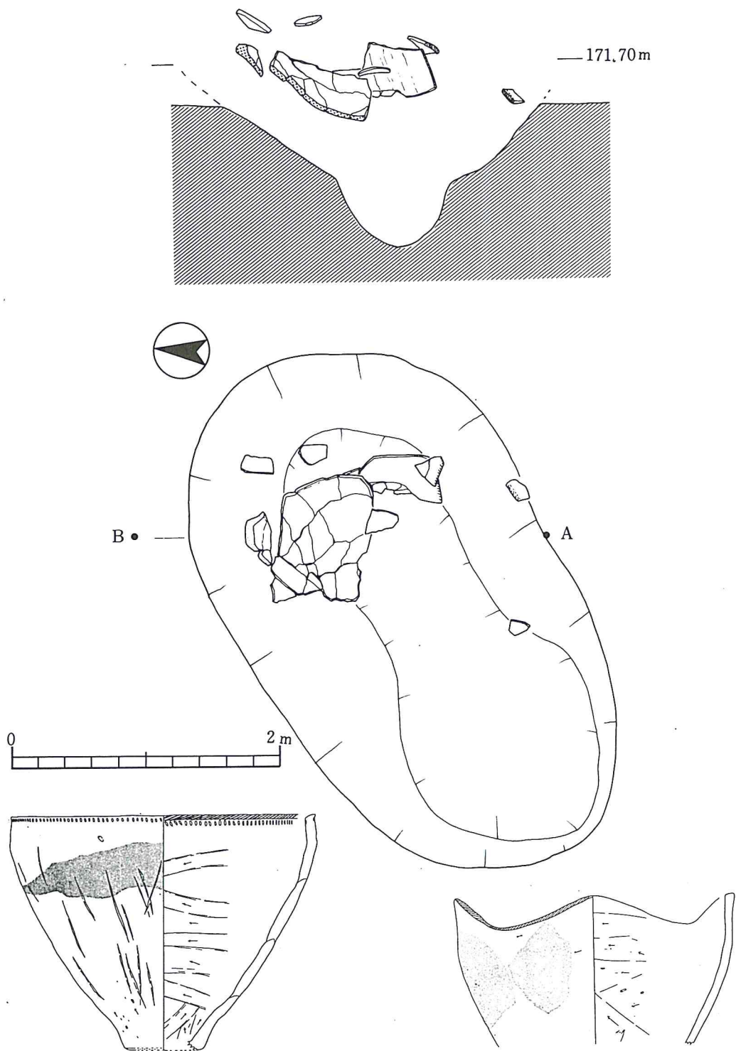
第8图 2号土坛平面图·断面图
