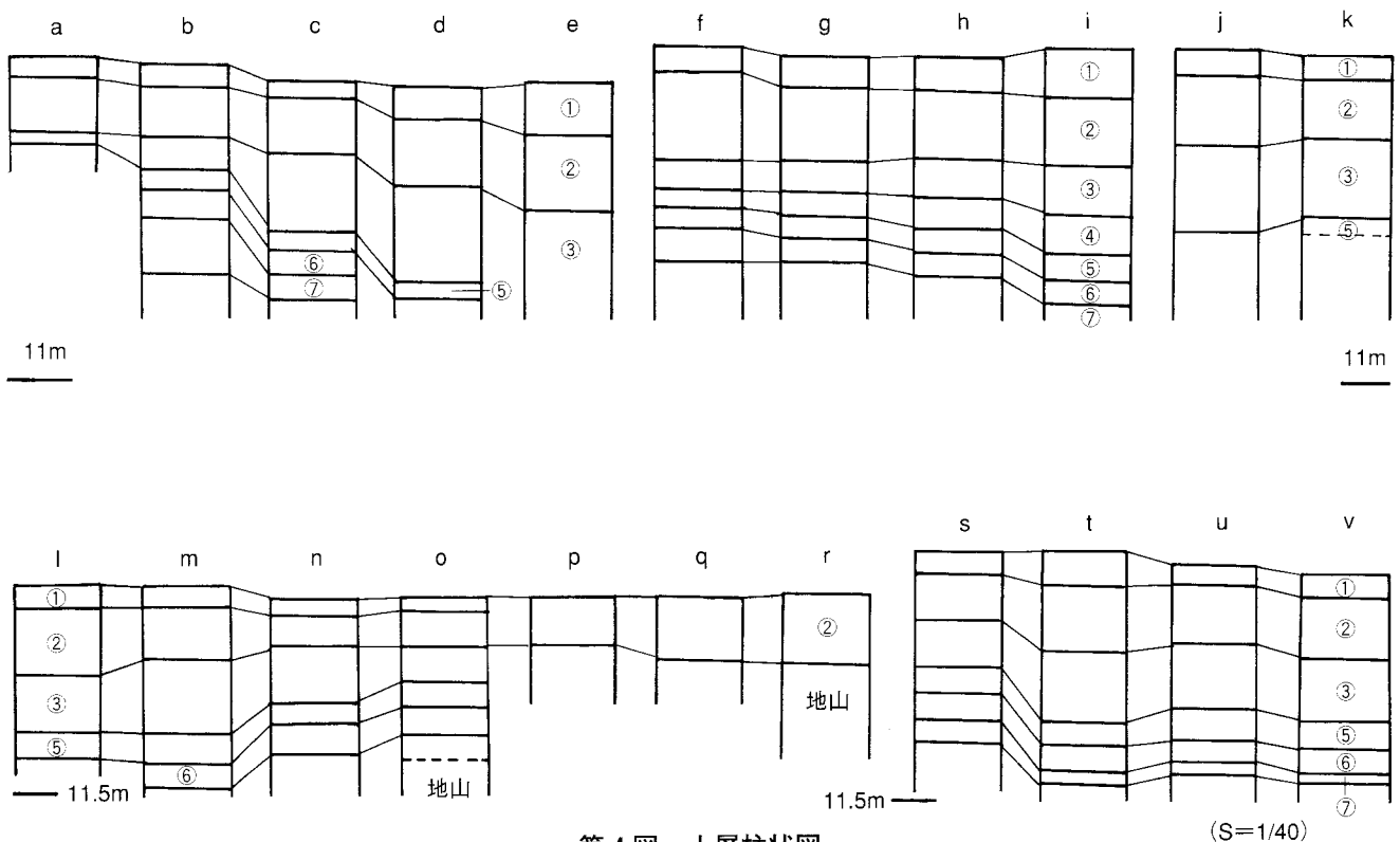
第4図 土層柱状図
