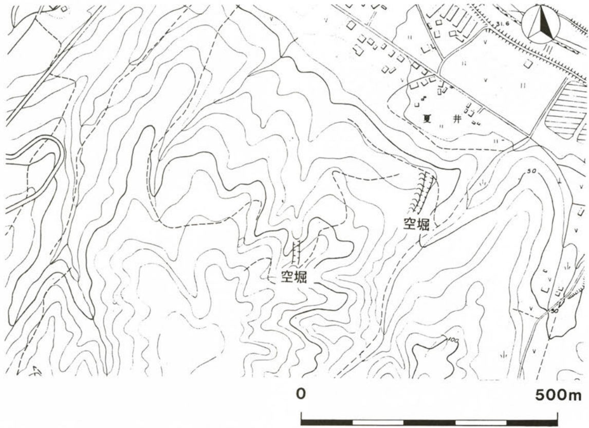
第6図 館の平館跡平面略図
